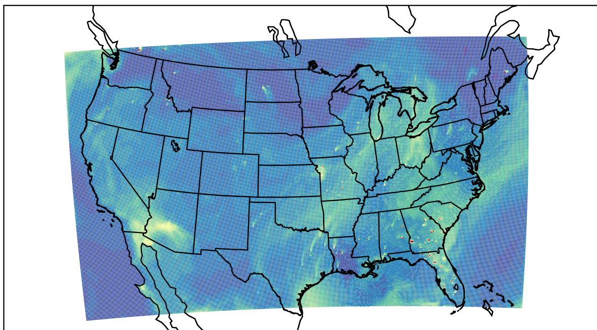
WRF 2022-08-03_20:00:00
