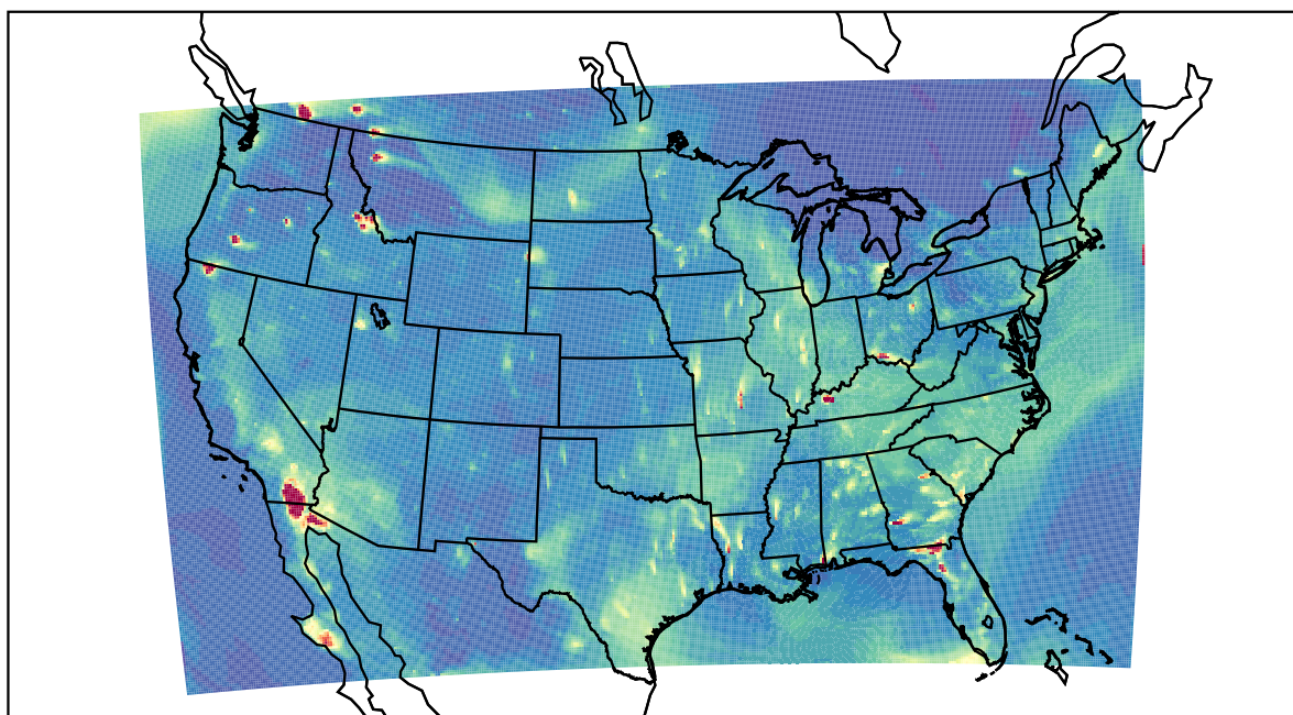
WRF 2022-08-03_03:00:00
