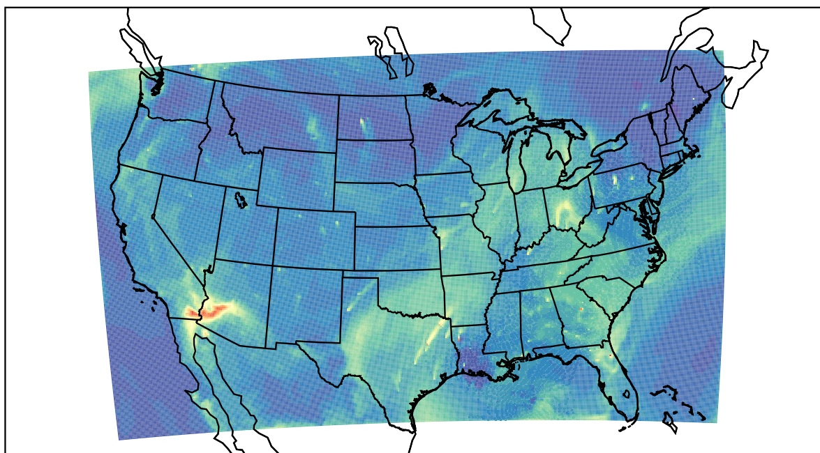
WRF 2022-08-03_16:00:00
