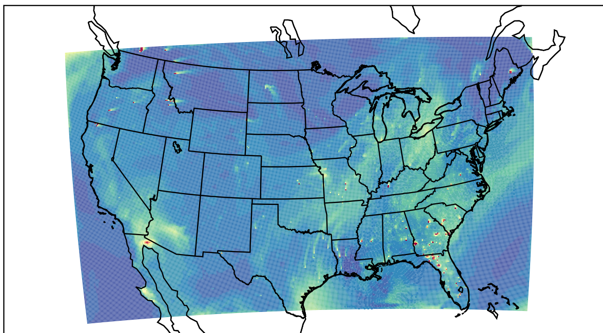
WRF 2022-08-03_23:00:00
