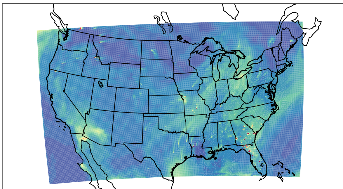
WRF 2022-08-03_22:00:00
