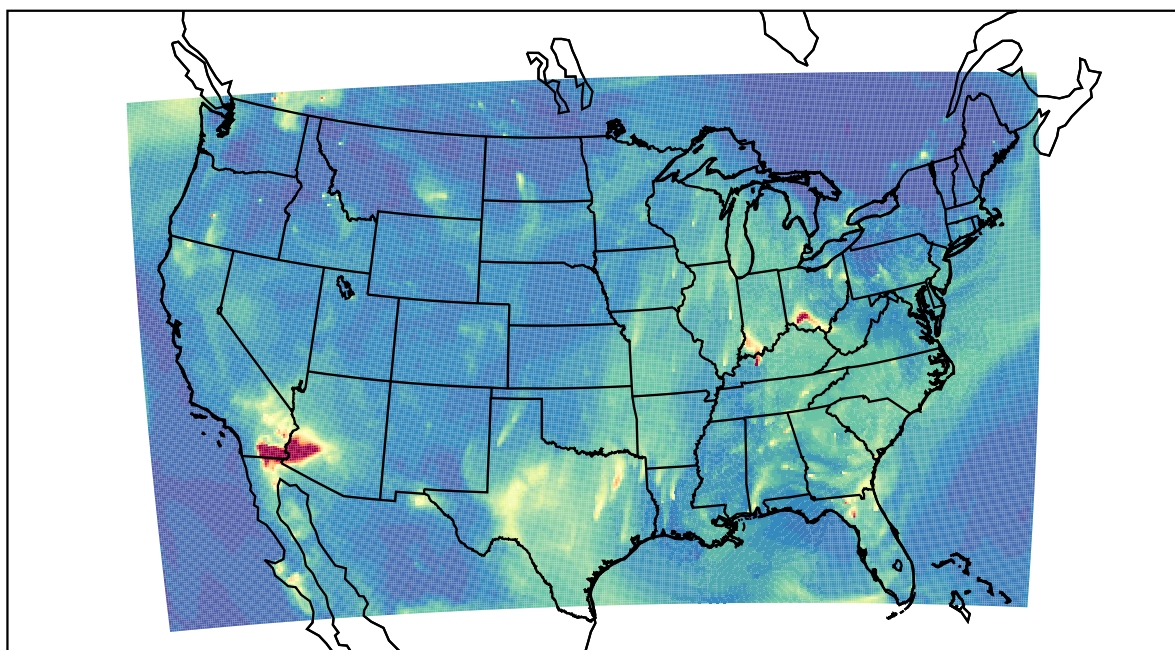
WRF 2022-08-03_10:00:00
