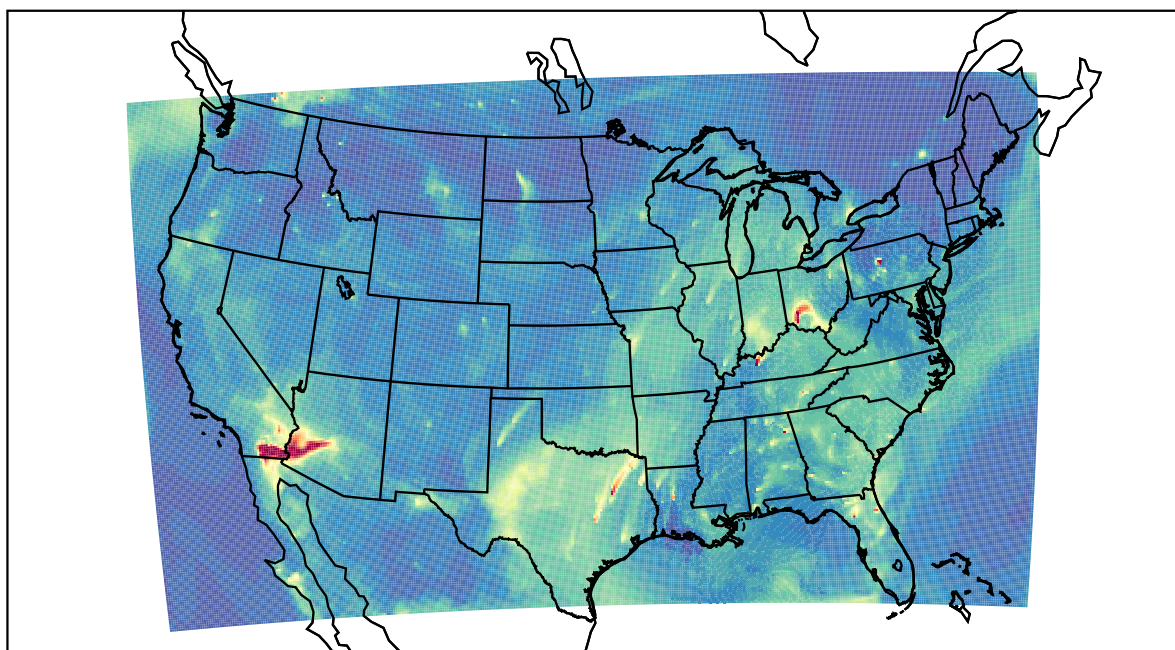
WRF 2022-08-03_13:00:00
