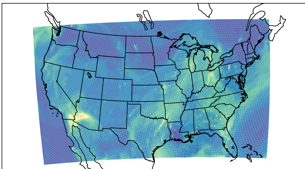
WRF 2022-08-03_18:00:00
