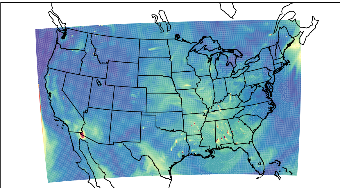
WRF 2022-08-16_20:00:00
