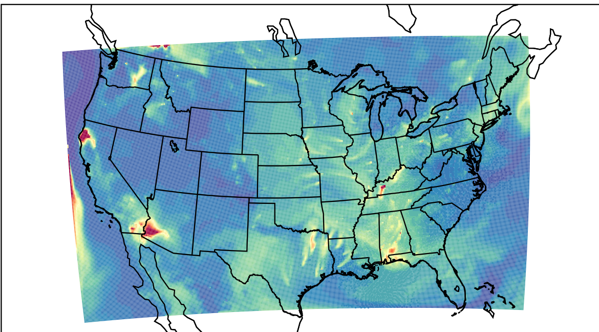
WRF 2022-08-17_09:00:00
