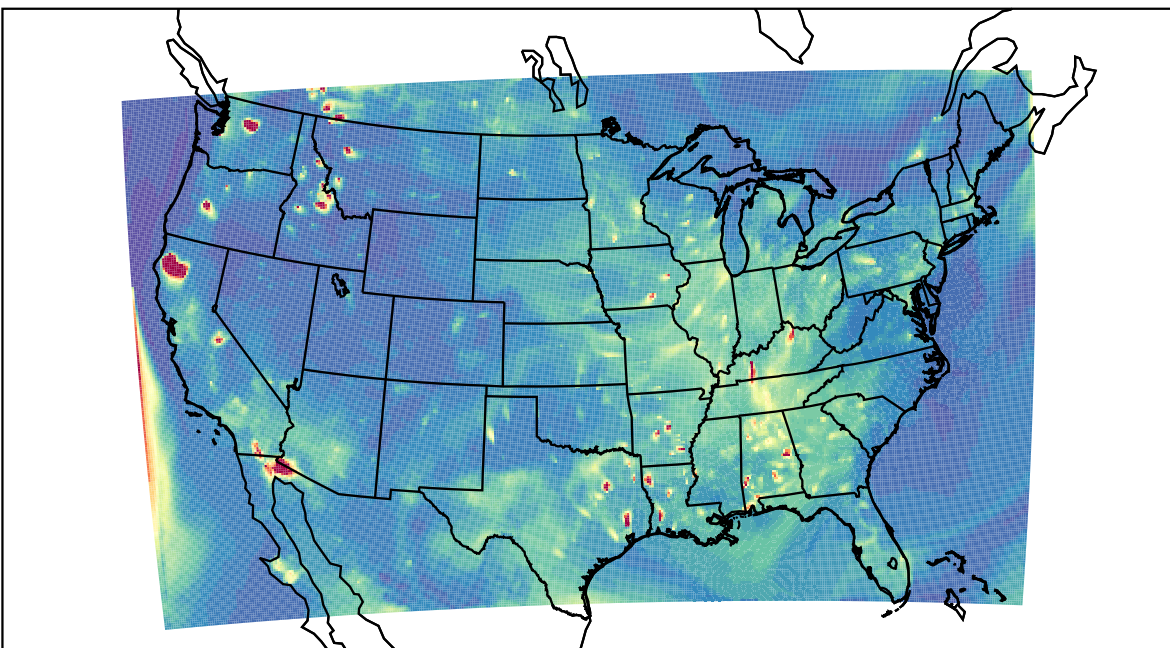
WRF 2022-08-16_03:00:00
