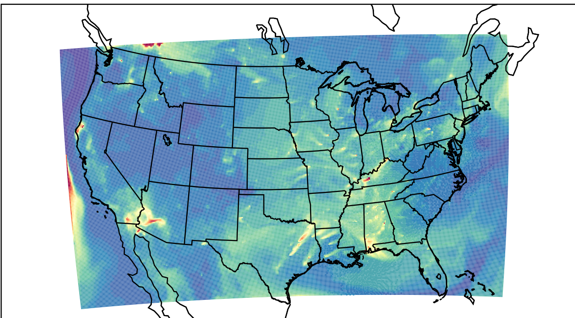
WRF 2022-08-17_13:00:00
