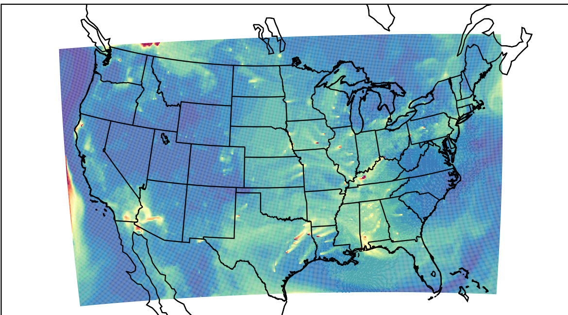
WRF 2022-08-17_14:00:00
