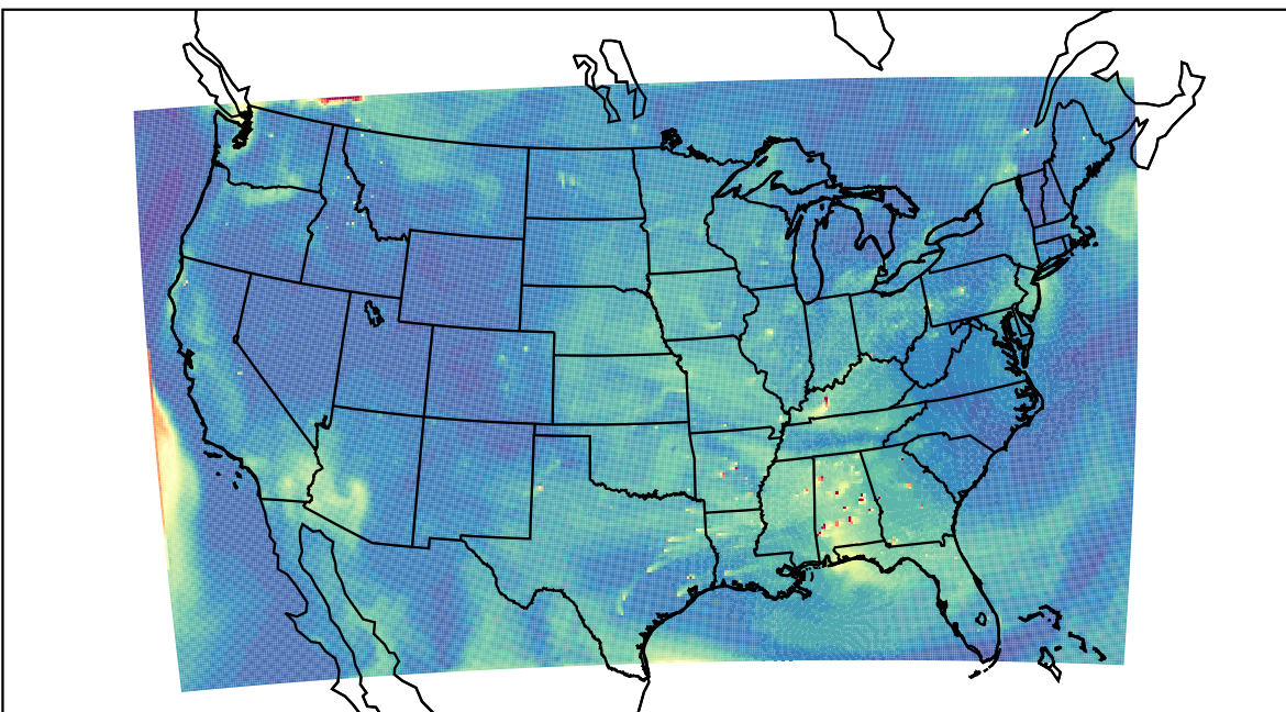
WRF 2022-08-17_19:00:00
