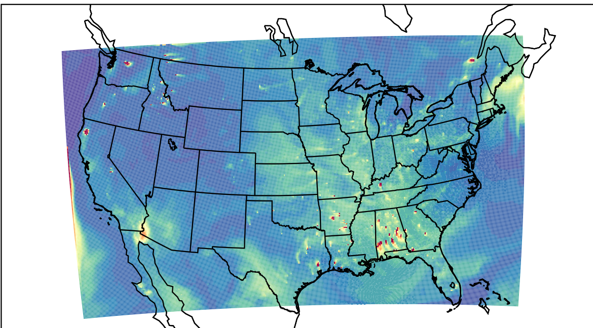
WRF 2022-08-17_00:00:00
