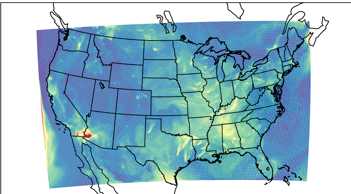
WRF 2022-08-16_10:00:00
