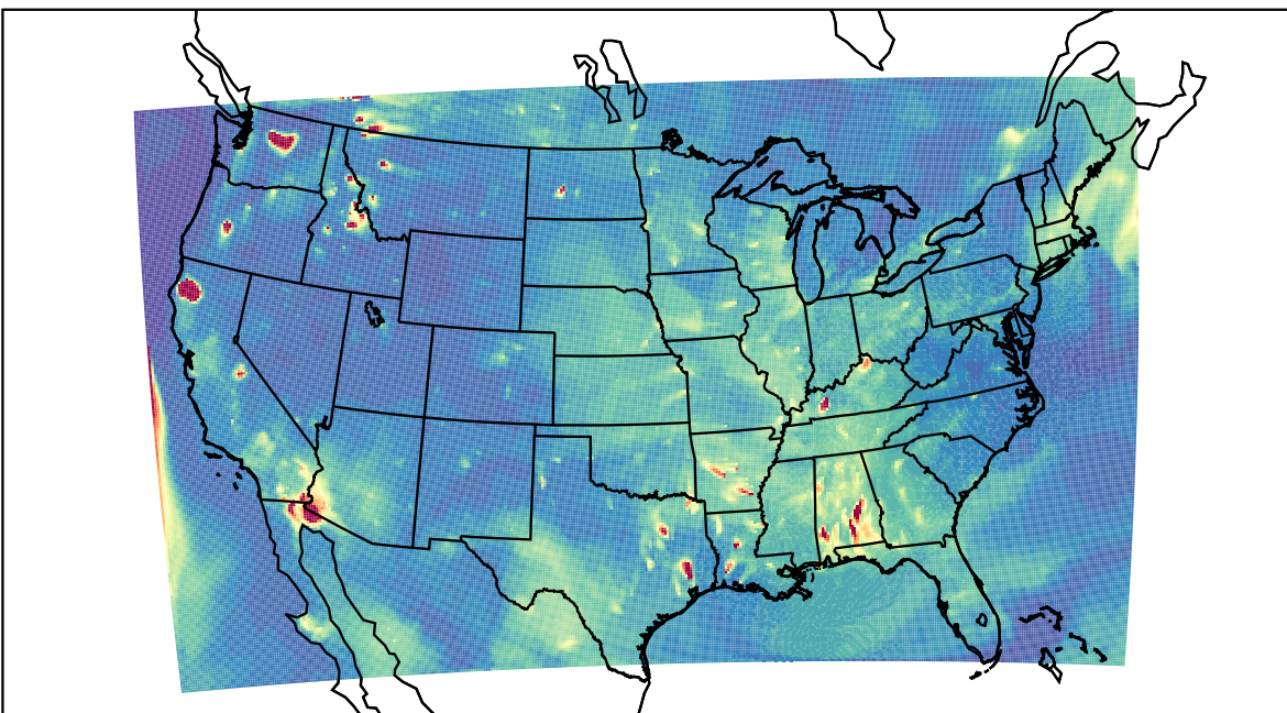
WRF 2022-08-17_03:00:00
