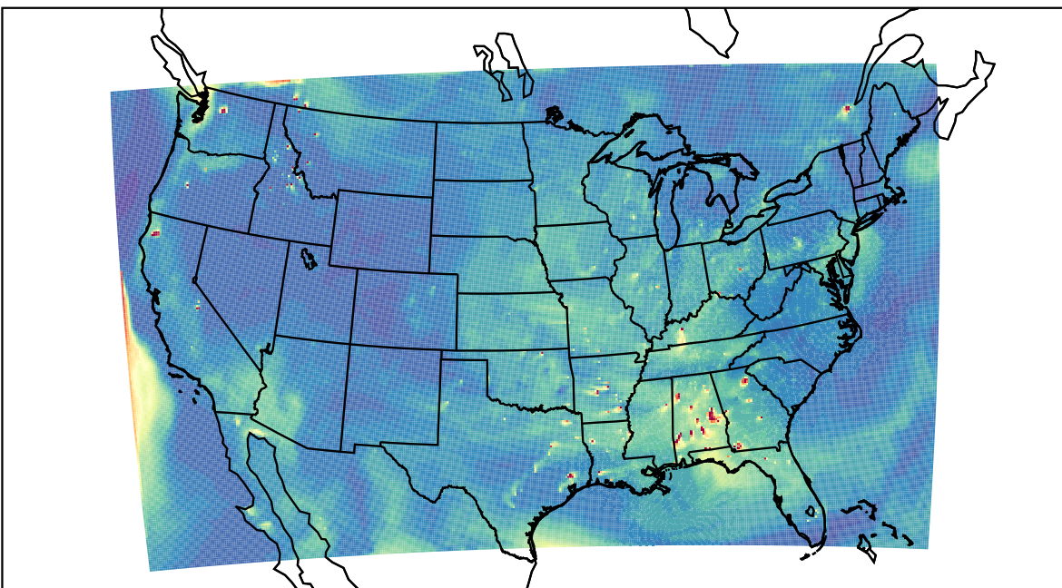
WRF 2022-08-17_23:00:00
