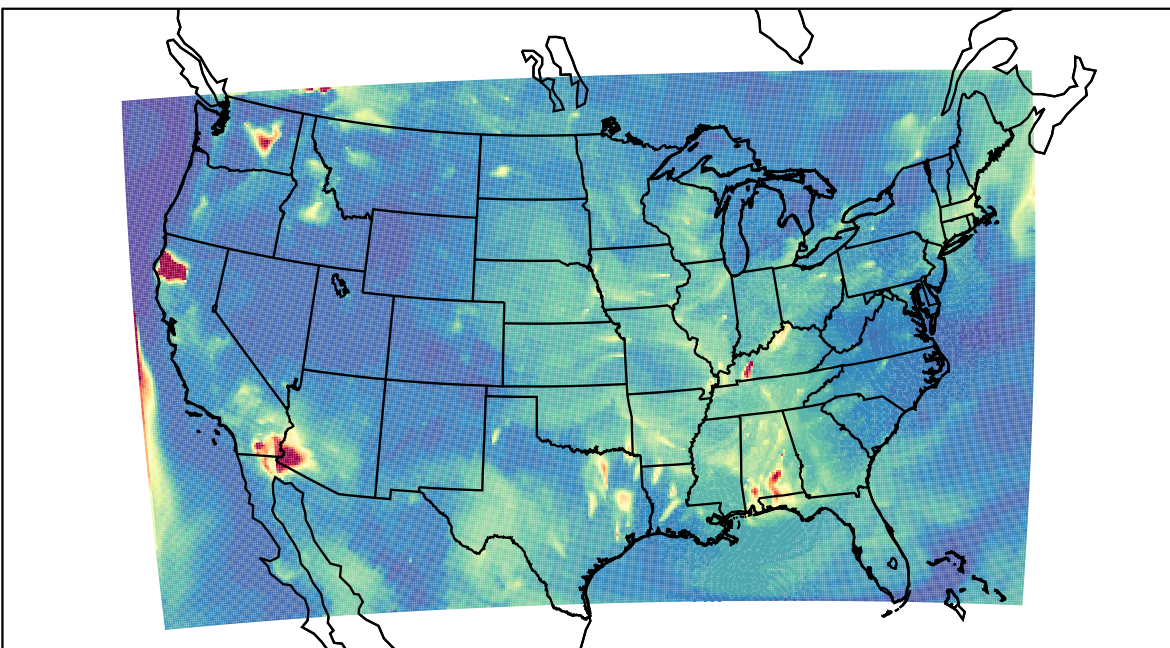
WRF 2022-08-17_06:00:00
