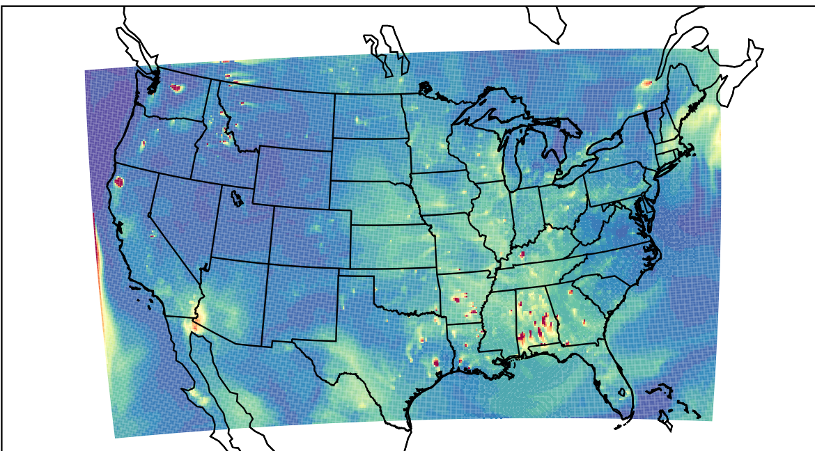
WRF 2022-08-17_01:00:00
