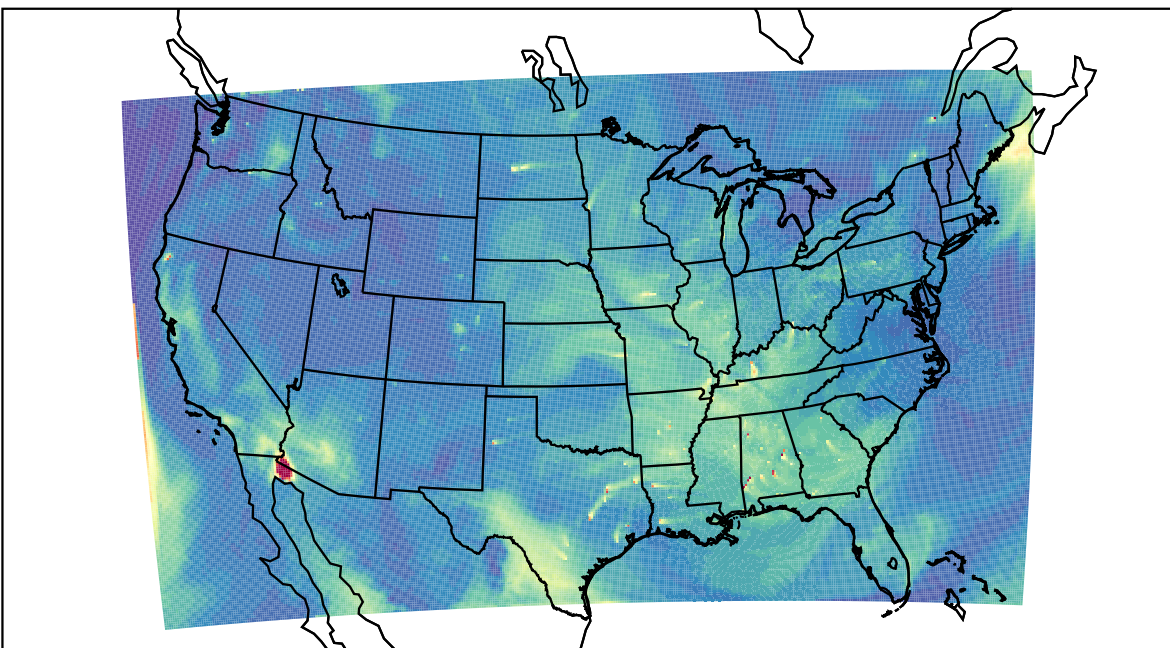
WRF 2022-08-16_18:00:00
