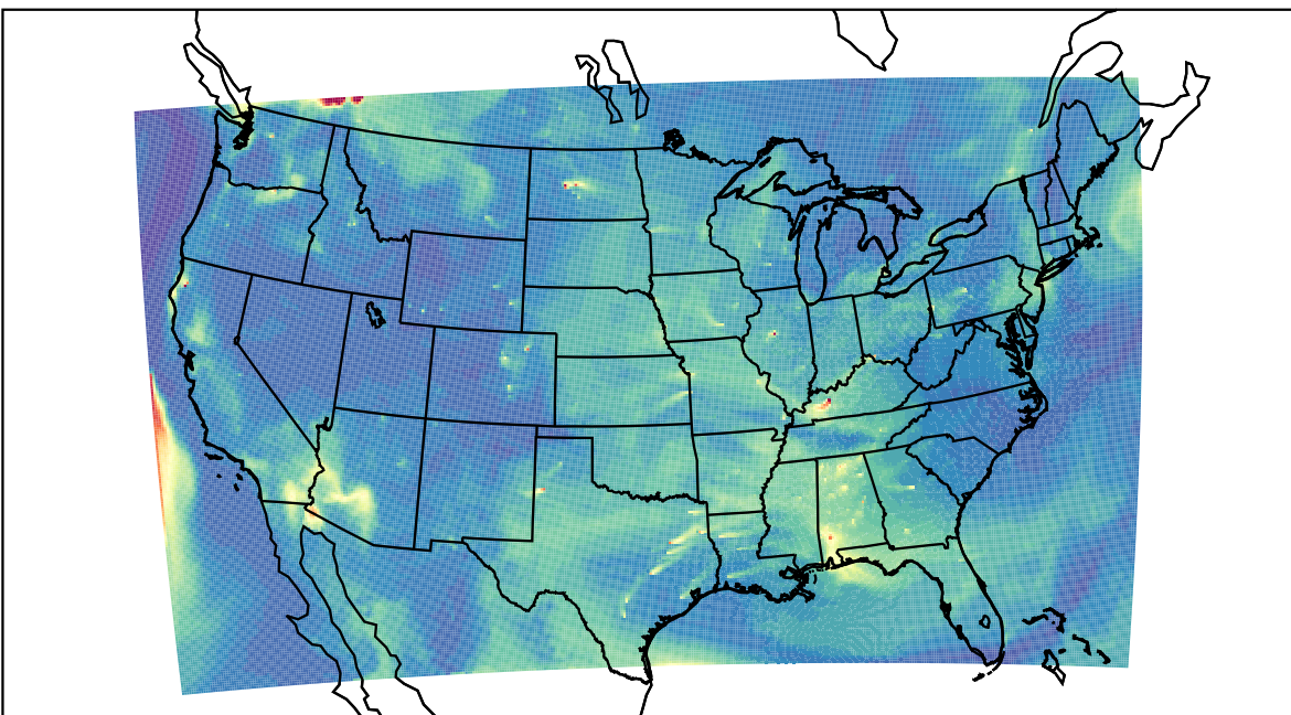
WRF 2022-08-17_16:00:00
