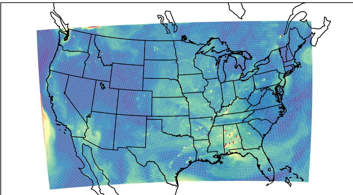
WRF 2022-08-17_20:00:00
