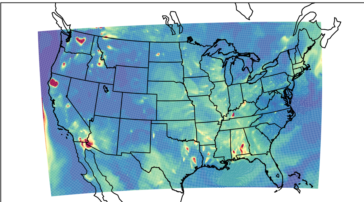
WRF 2022-08-17_04:00:00
