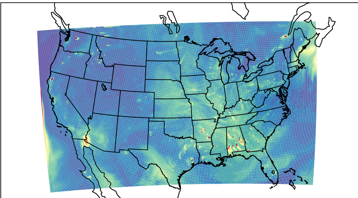
WRF 2022-08-16_23:00:00
