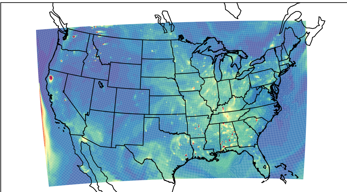
WRF 2022-08-16_01:00:00
