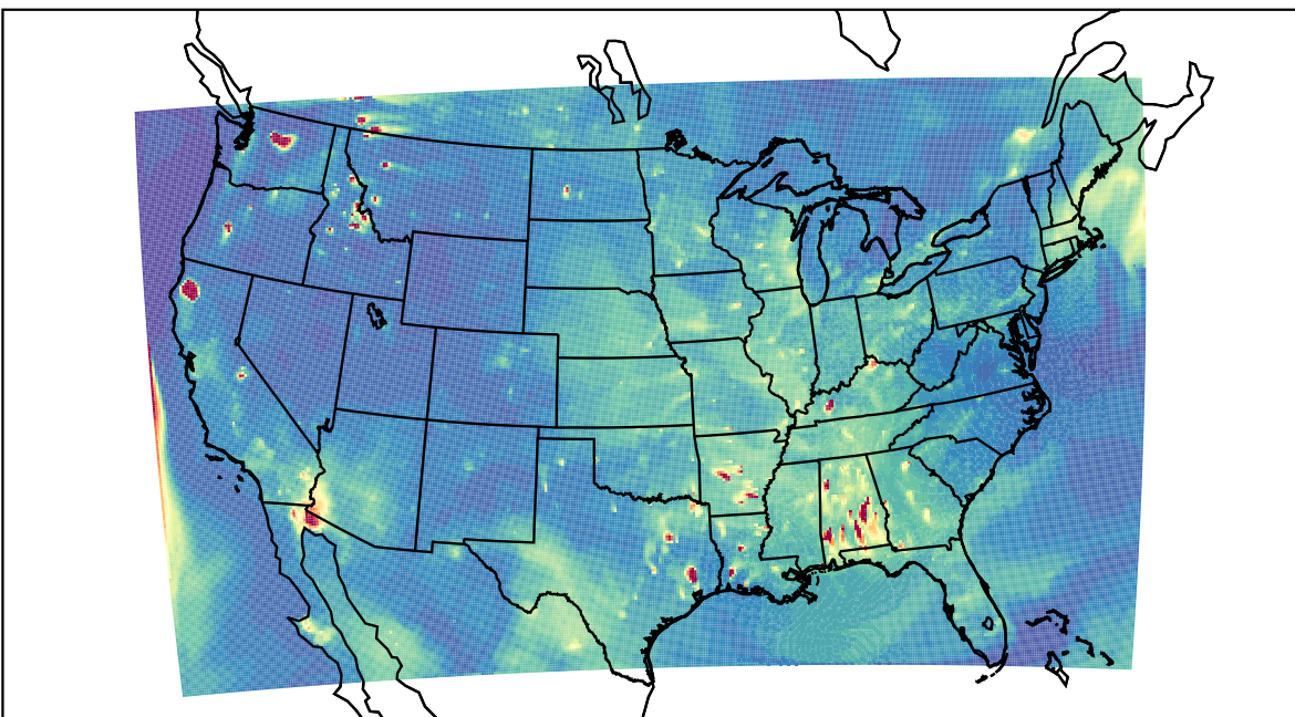
WRF 2022-08-17_02:00:00
