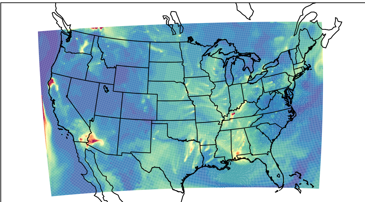
WRF 2022-08-17_10:00:00
