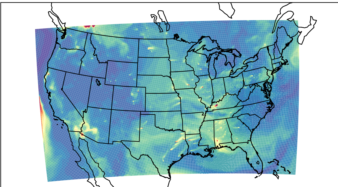
WRF 2022-08-17_15:00:00
