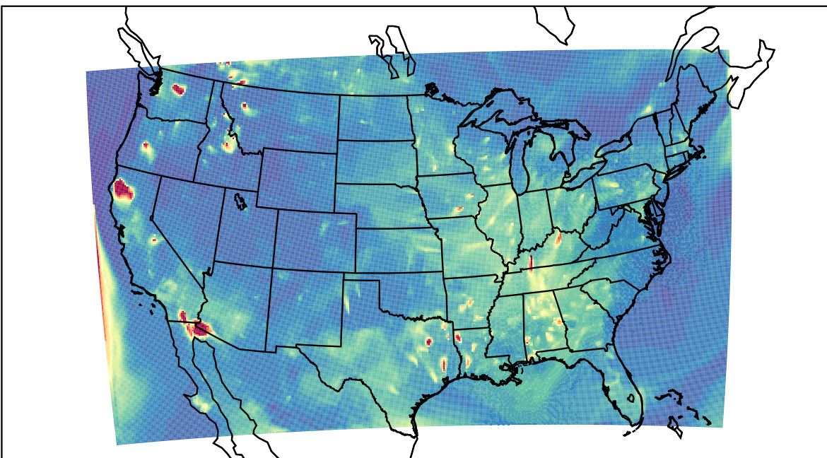
WRF 2022-08-16_04:00:00
