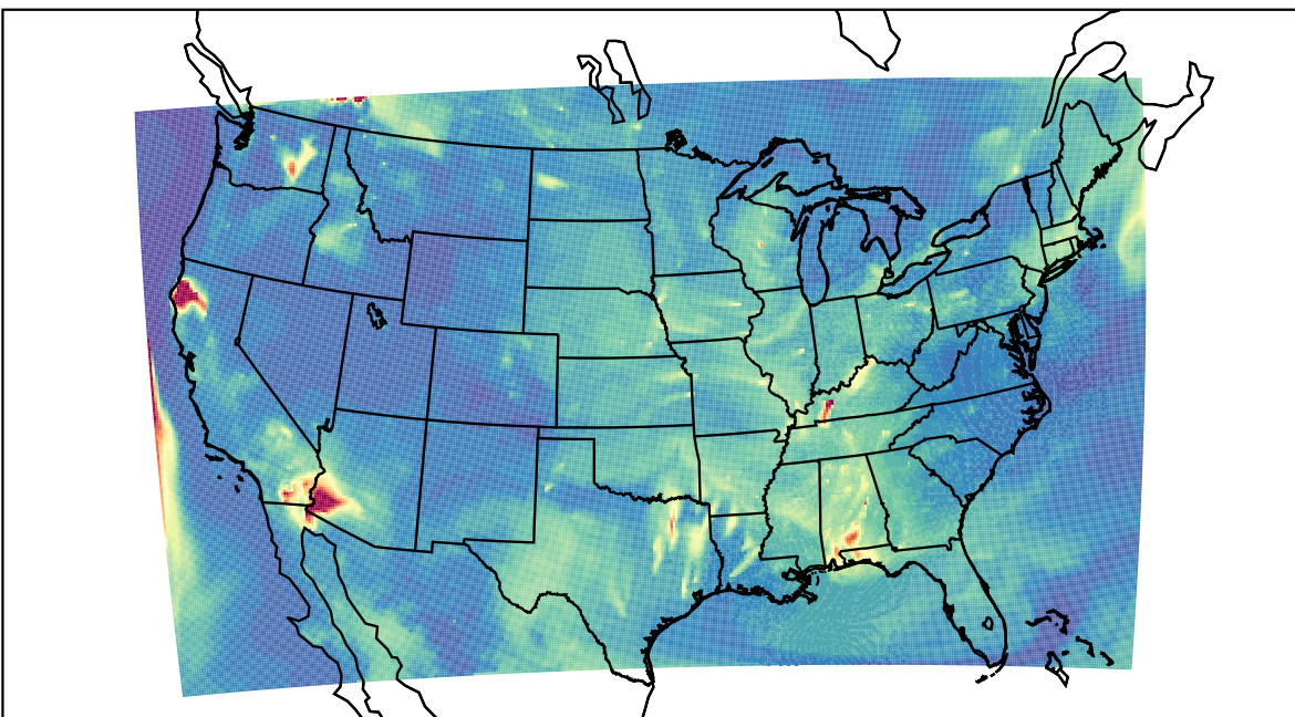
WRF 2022-08-17_08:00:00
