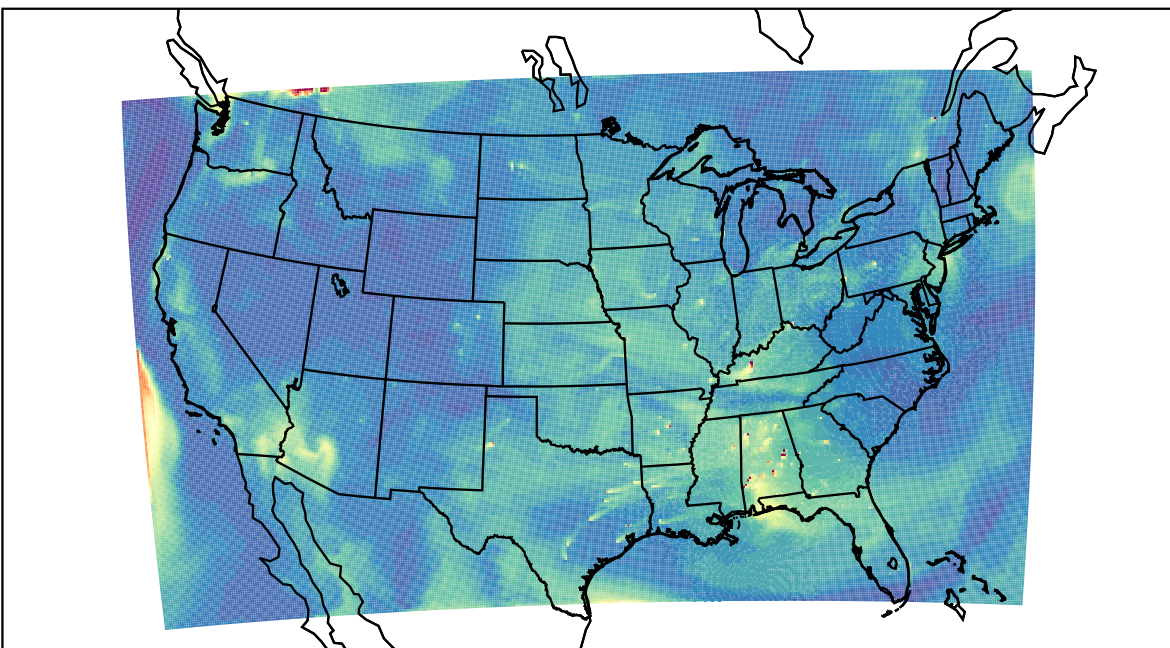
WRF 2022-08-17_18:00:00
