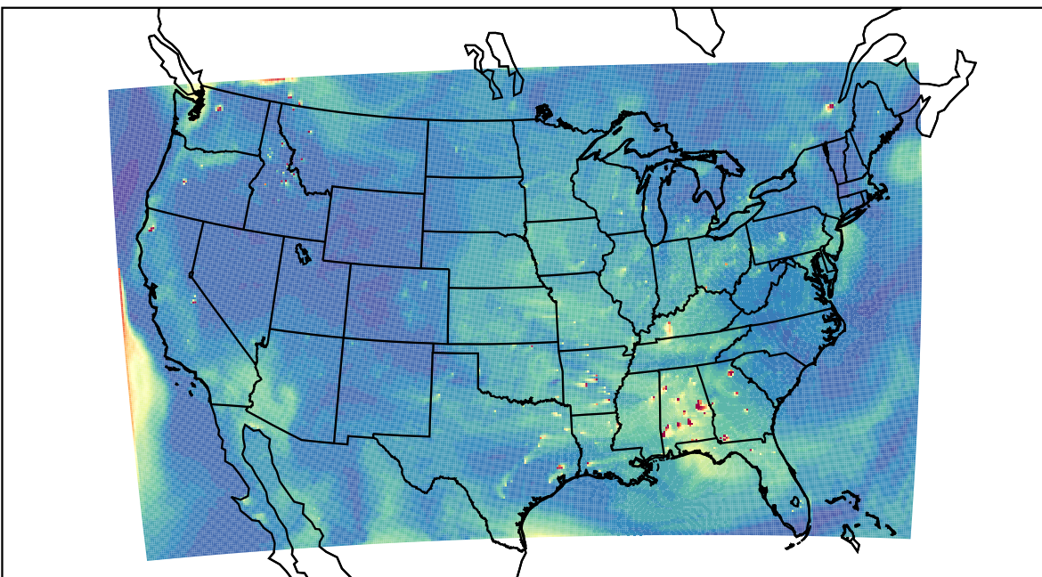
WRF 2022-08-17_22:00:00
