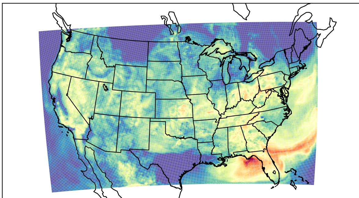
WRF (2022-08-18_14:00:00)
