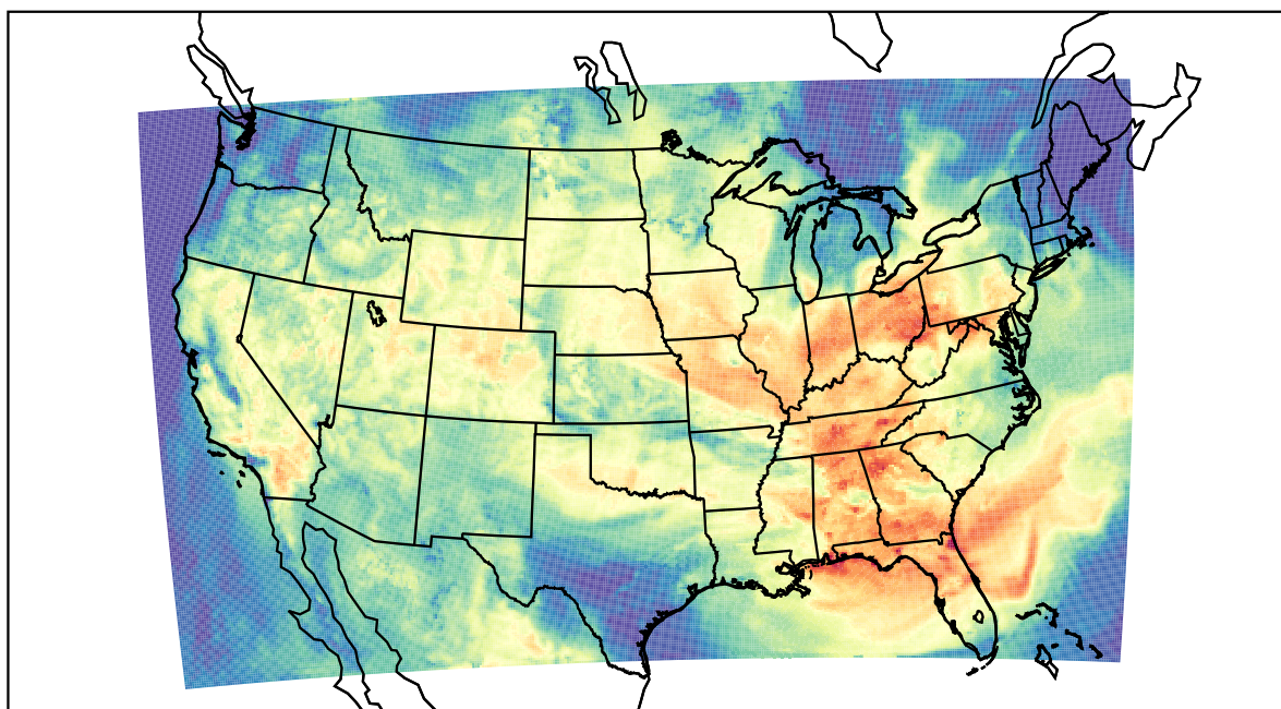
WRF (2022-08-17_16:00:00)
