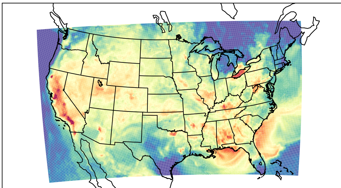
WRF (2022-08-17_01:00:00)
