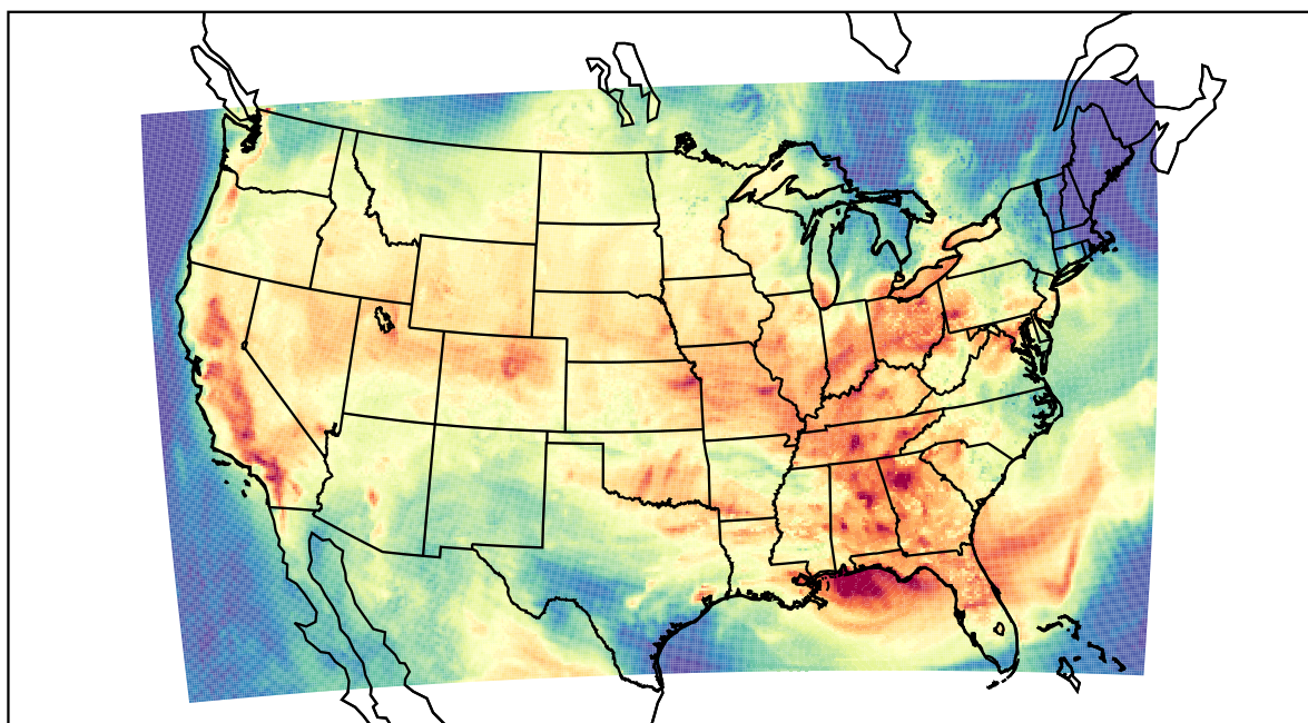
WRF (2022-08-17_20:00:00)
