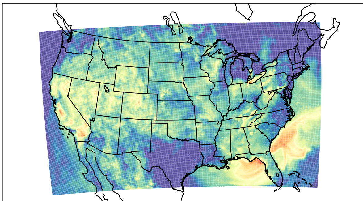
WRF (2022-08-17_10:00:00)
