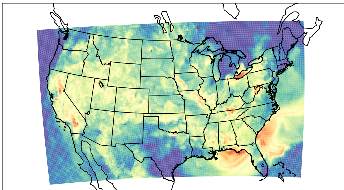
WRF (2022-08-17_04:00:00)
