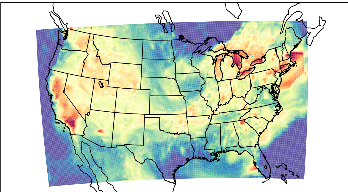
WRF (2022-08-21_01:00:00)
