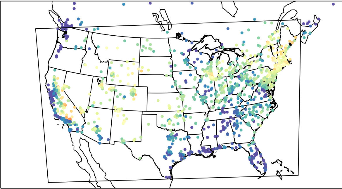
AirNOW (2022-08-21_16:00:00)
