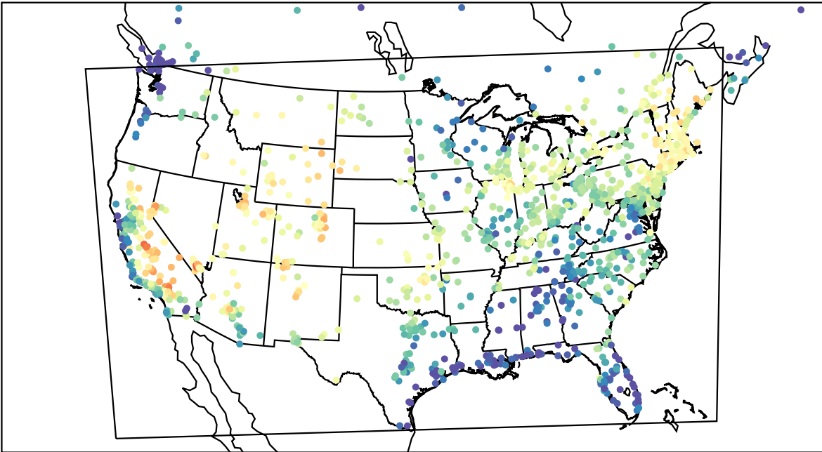
AirNOW (2022-08-21_18:00:00)
