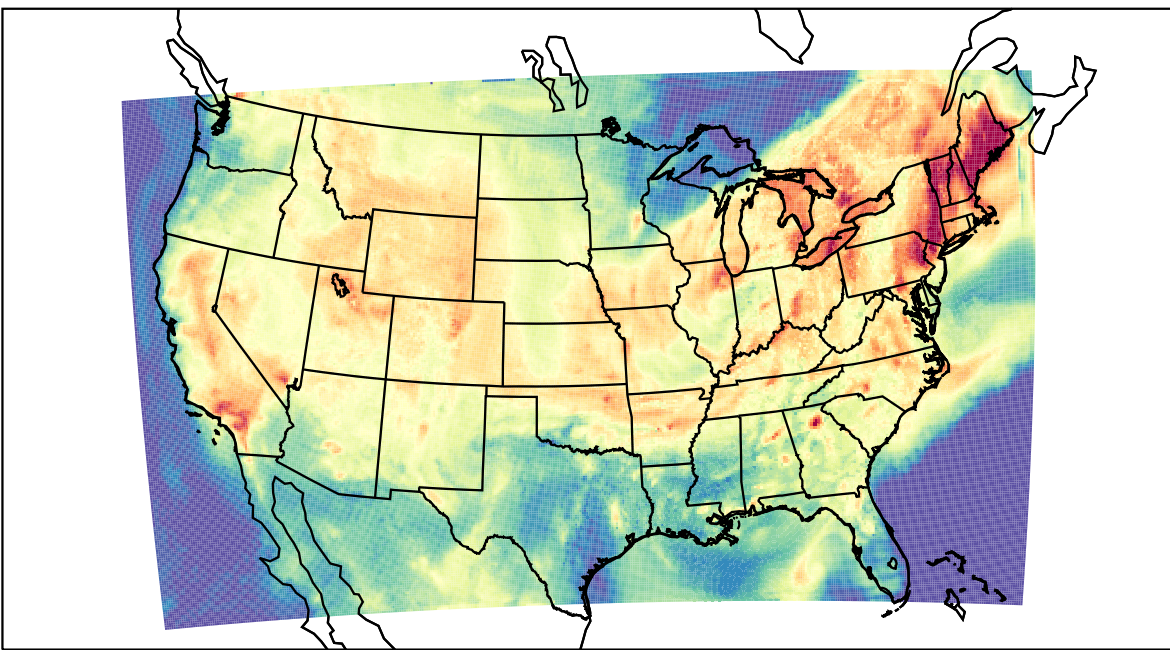
WRF (2022-08-21_20:00:00)
