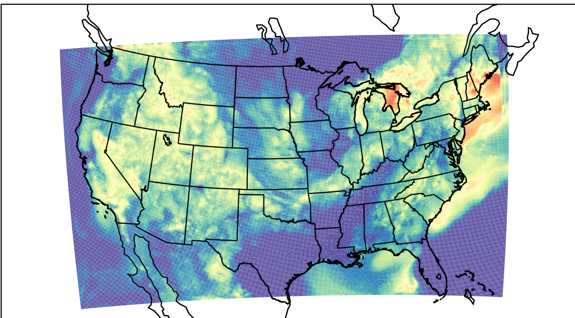
WRF (2022-08-21_10:00:00)
