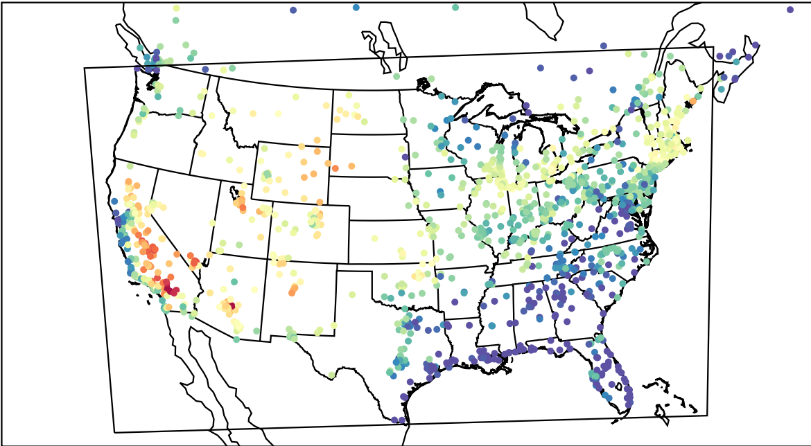
AirNOW (2022-08-21_23:00:00)
