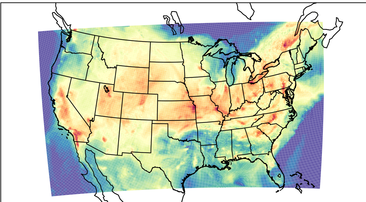
WRF (2022-08-22_20:00:00)
