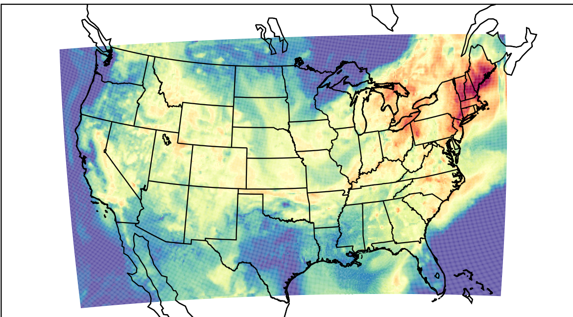
WRF (2022-08-21_16:00:00)
