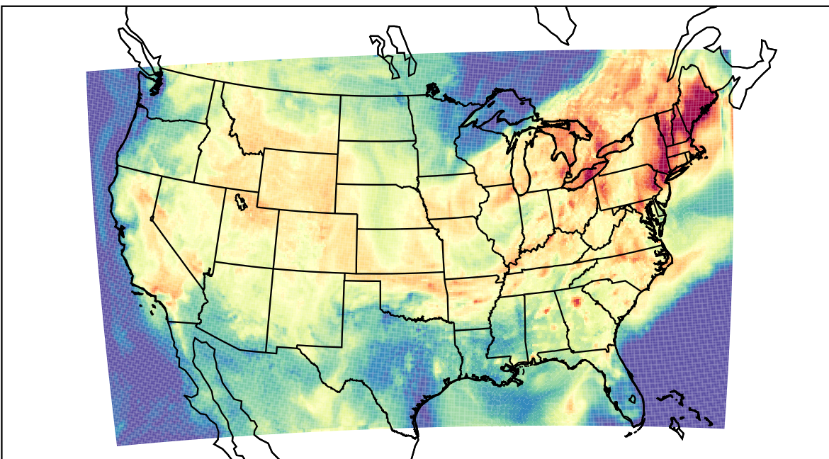
WRF (2022-08-21_18:00:00)
