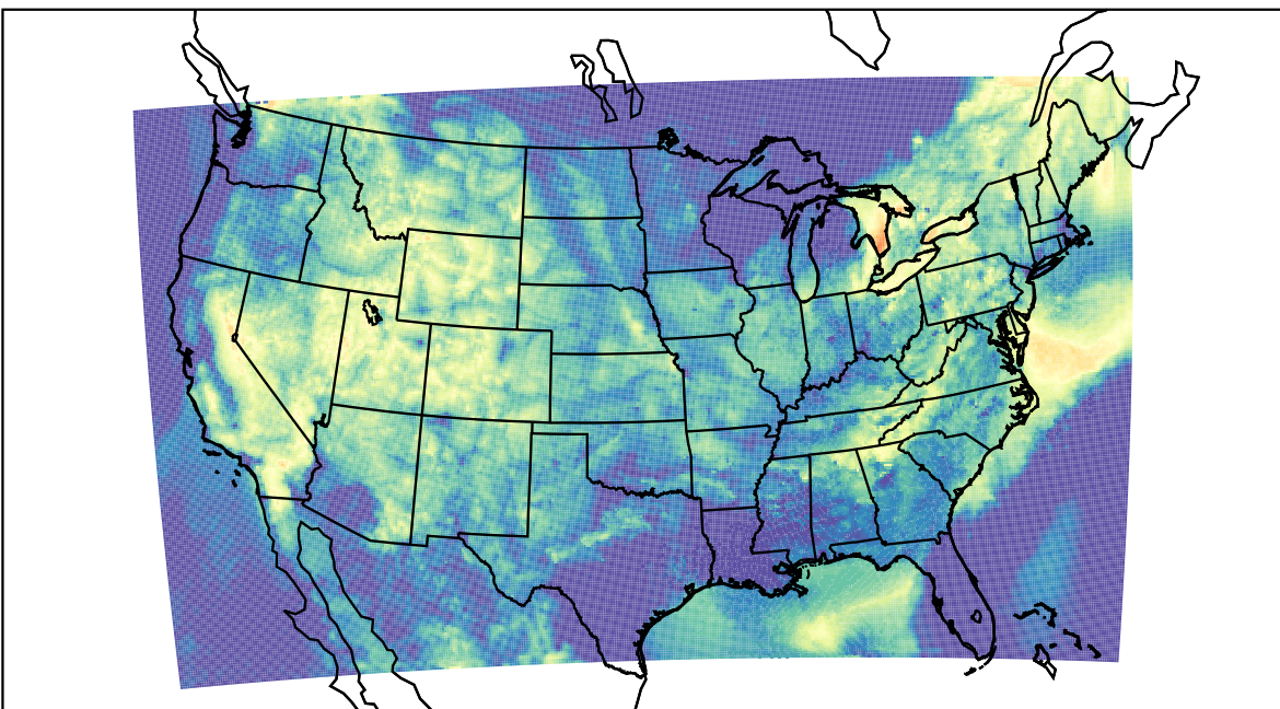
WRF (2022-08-22_13:00:00)
