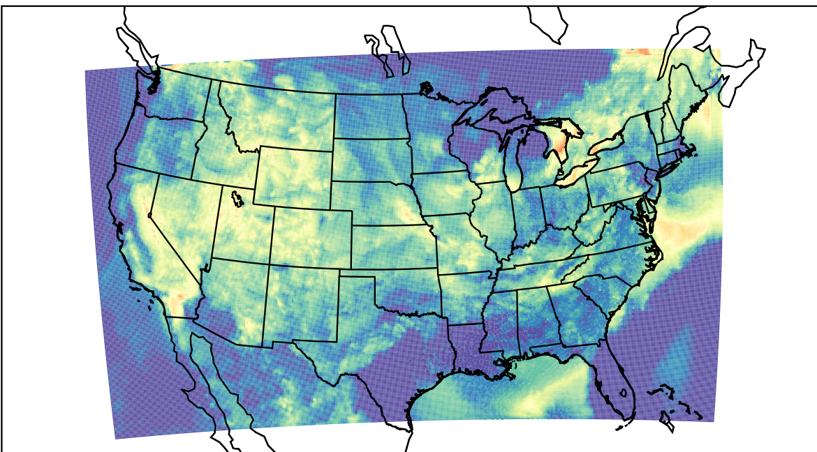
WRF (2022-08-22_10:00:00)
