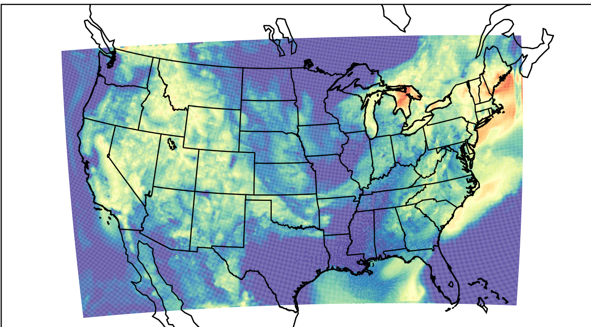
WRF (2022-08-21_13:00:00)
