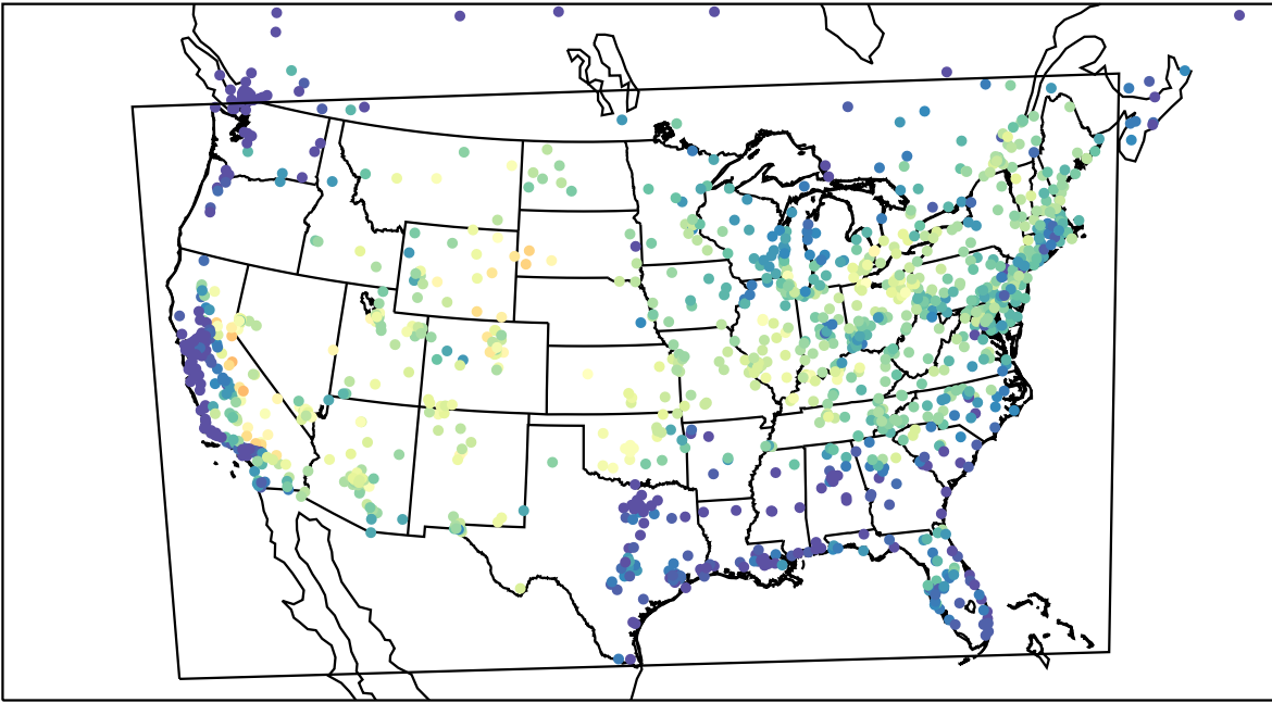
AirNOW (2022-08-22_16:00:00)
