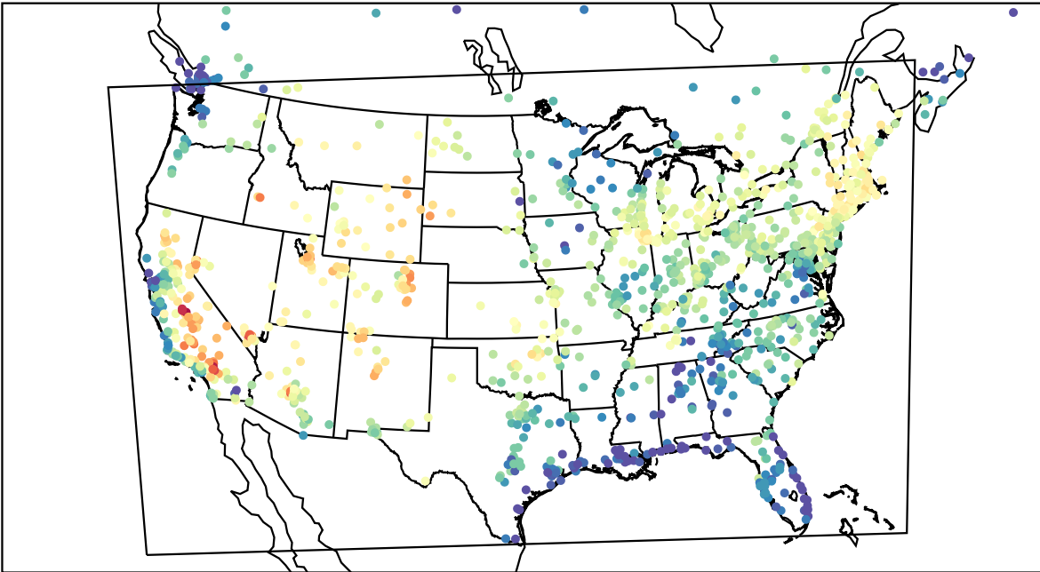
AirNOW (2022-08-21_19:00:00)
