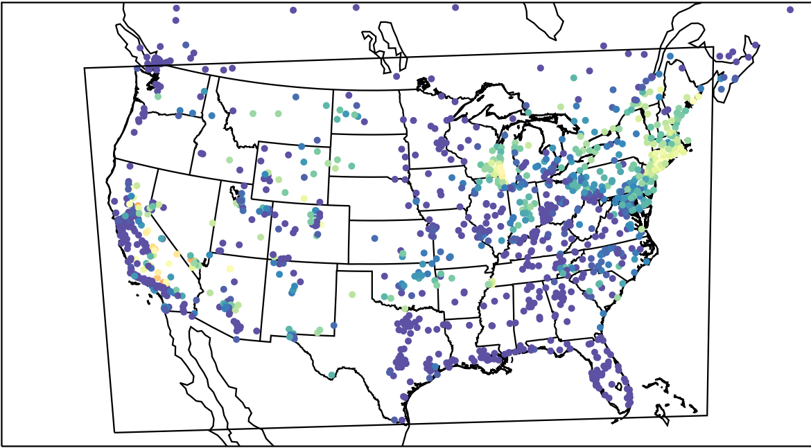
AirNOW (2022-08-21_13:00:00)
