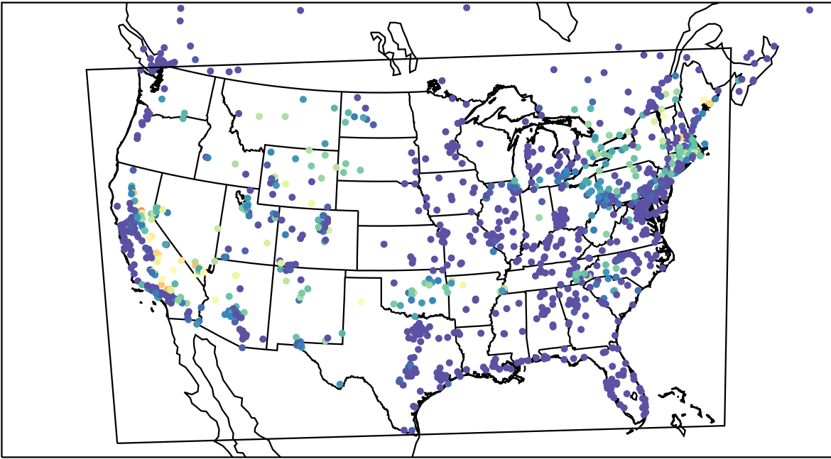
AirNOW (2022-08-21_10:00:00)
