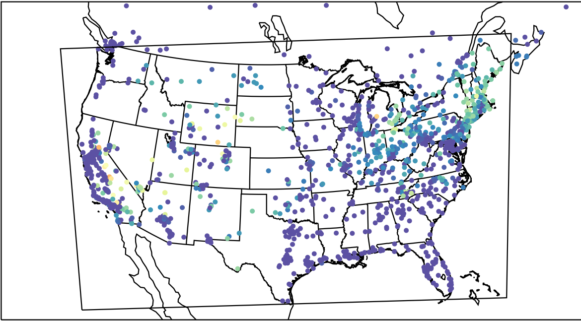
AirNOW (2022-08-22_13:00:00)
