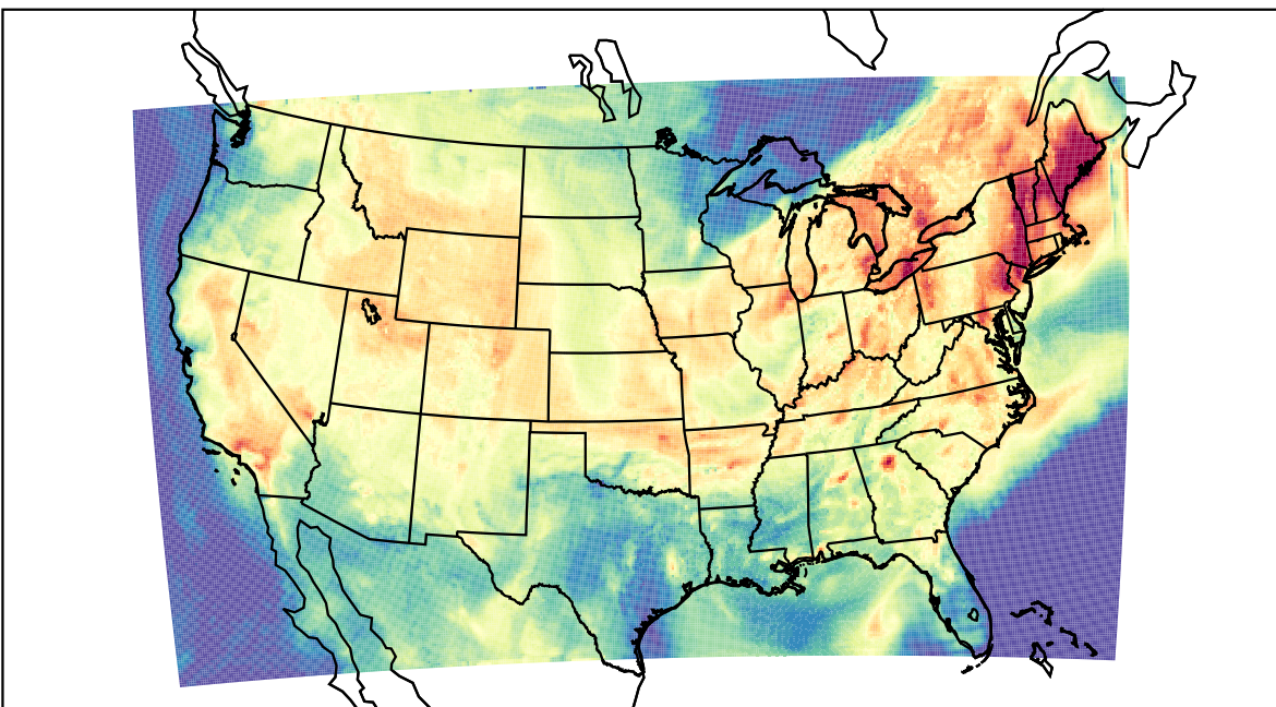
WRF (2022-08-21_19:00:00)
