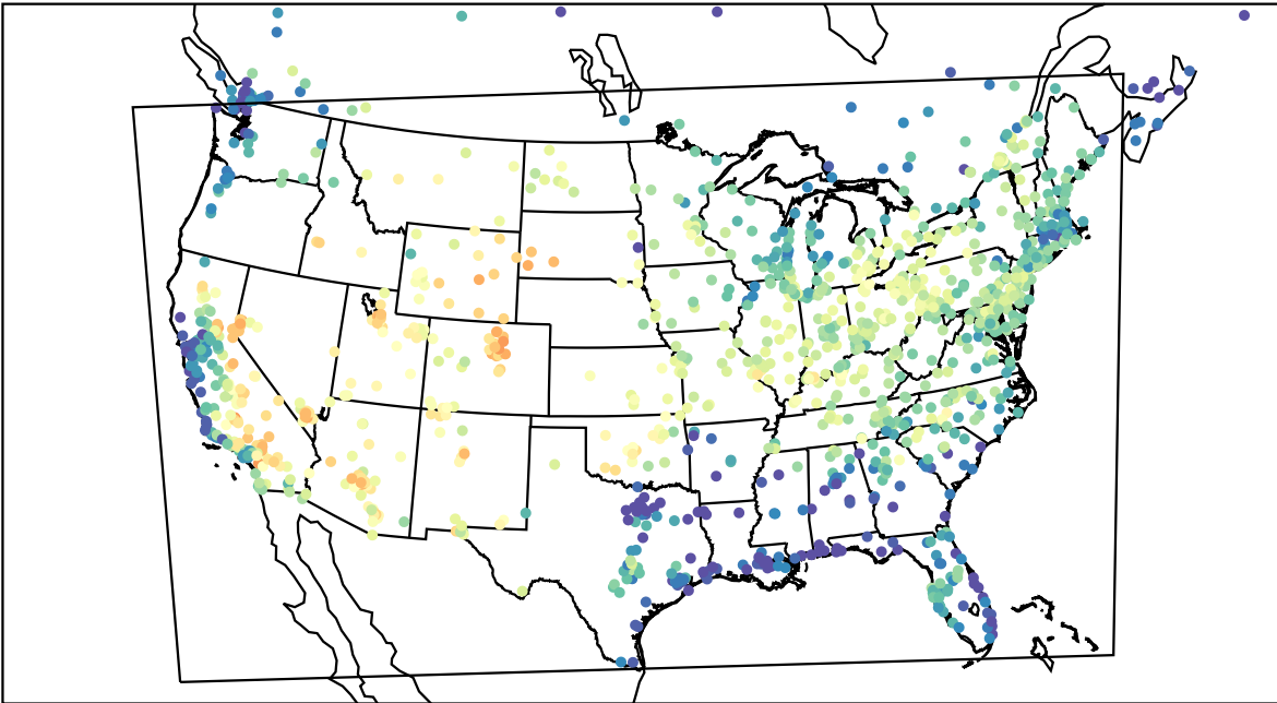
AirNOW (2022-08-22_18:00:00)
