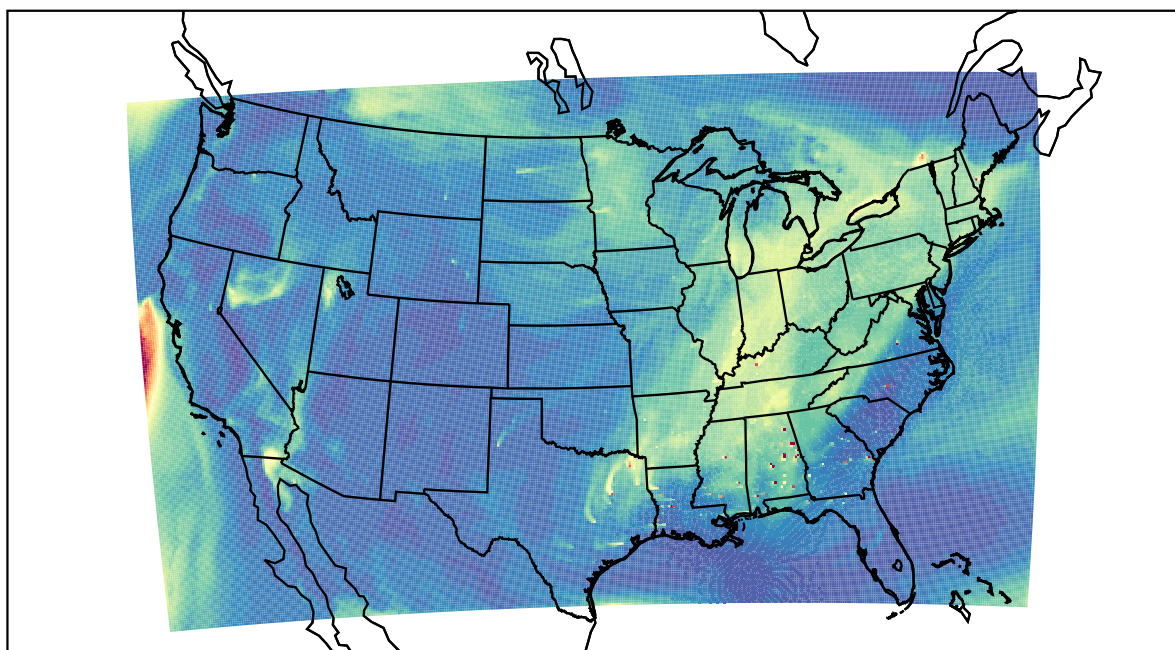
WRF 2022-09-18_18:00:00
