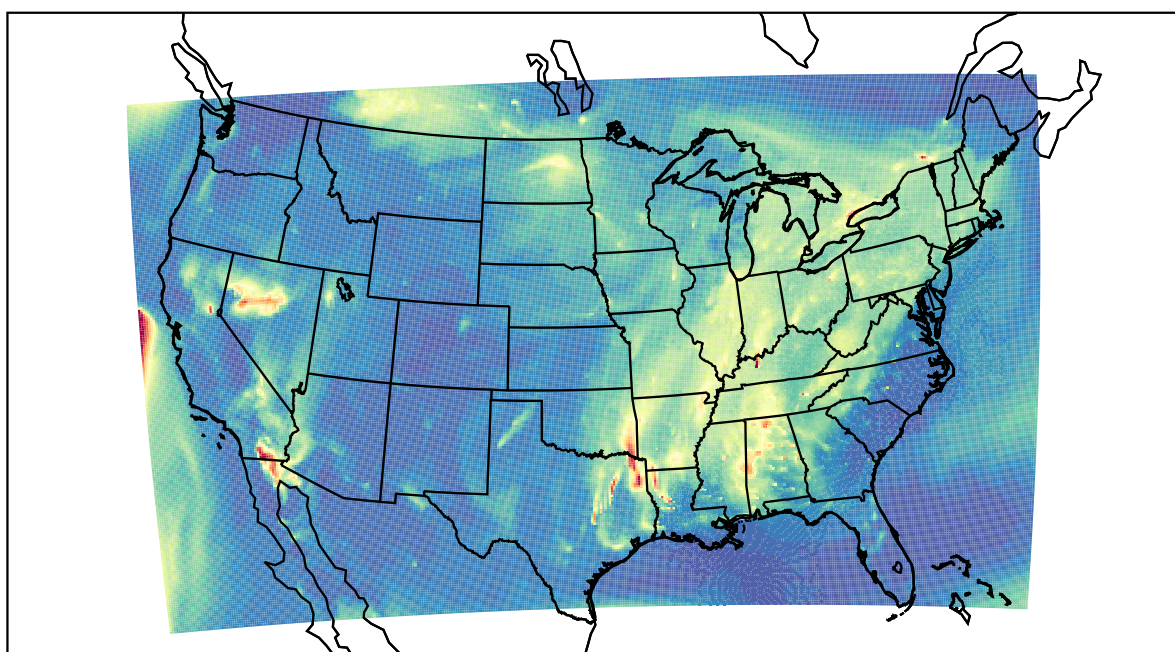
WRF 2022-09-18_13:00:00
