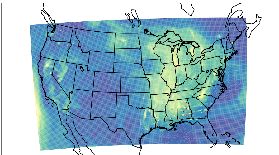
WRF 2022-09-17_20:00:00
