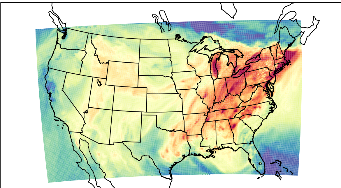
WRF (2022-09-18_20:00:00)
