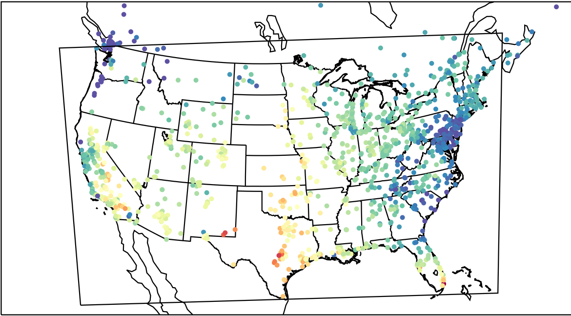
AirNOW (2022-10-03_18:00:00)
