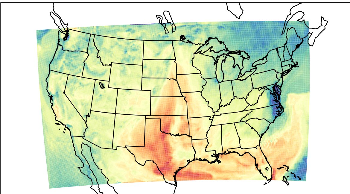
WRF (2022-10-03_18:00:00)
