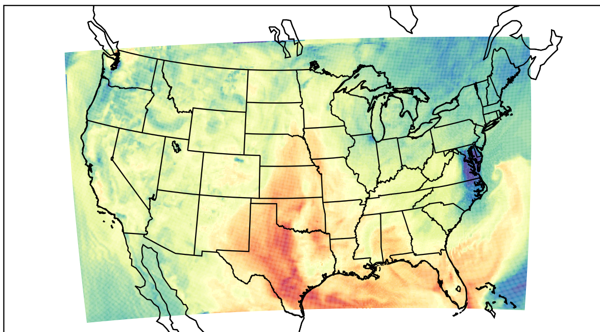
WRF (2022-10-03_18:00:00)
