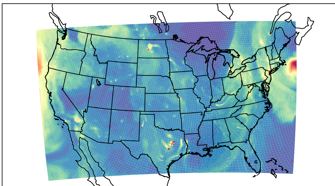
WRF 2022-10-26_16:00:00
