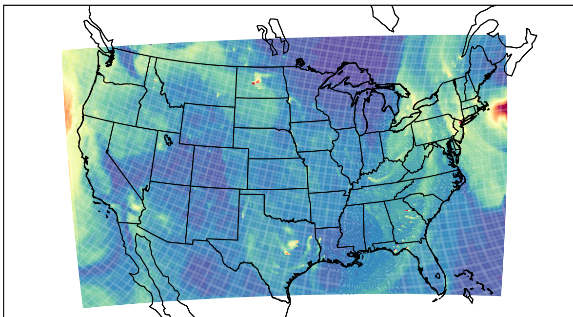
WRF 2022-10-26_18:00:00
