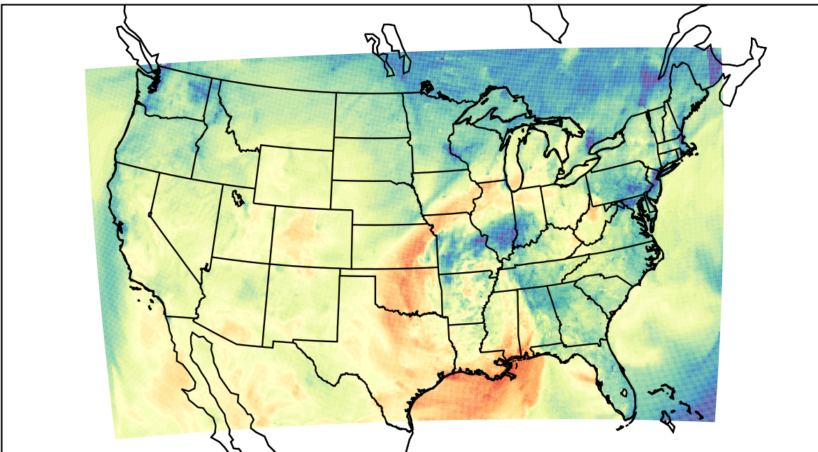
WRF (2022-10-30_22:00:00)
