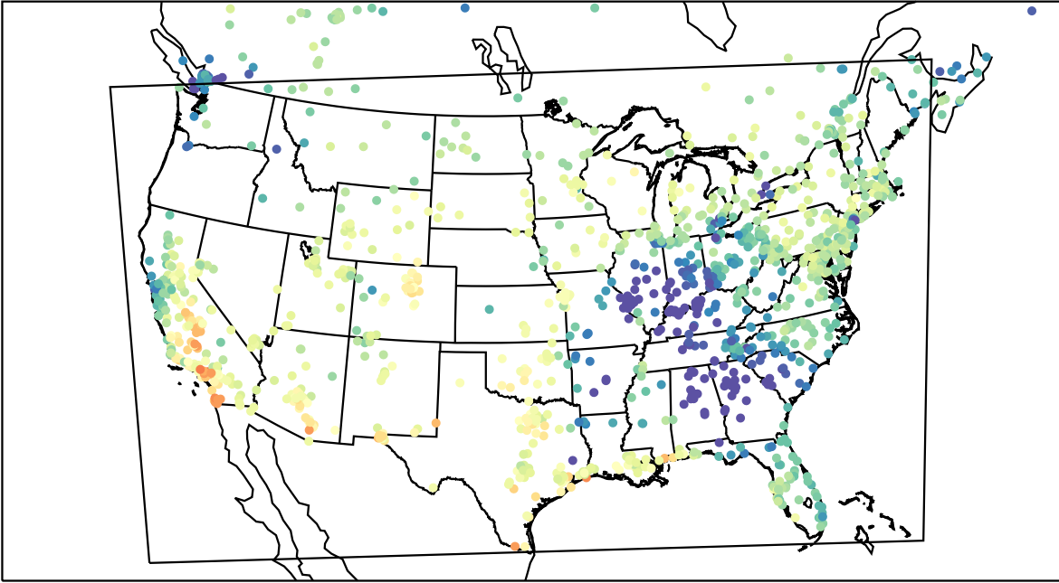
AirNOW (2022-10-30_20:00:00)
