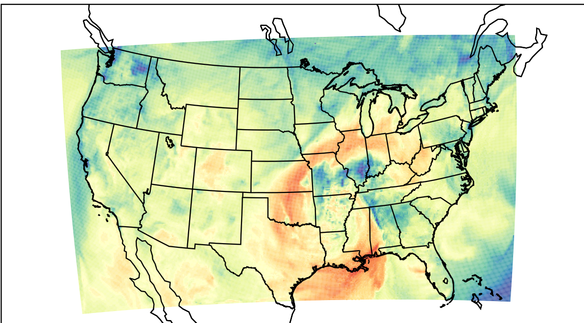
WRF (2022-10-30_20:00:00)
