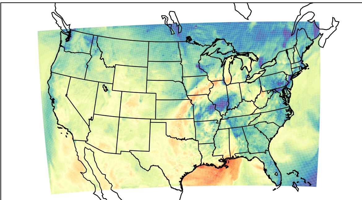
WRF (2022-10-30_23:00:00)
