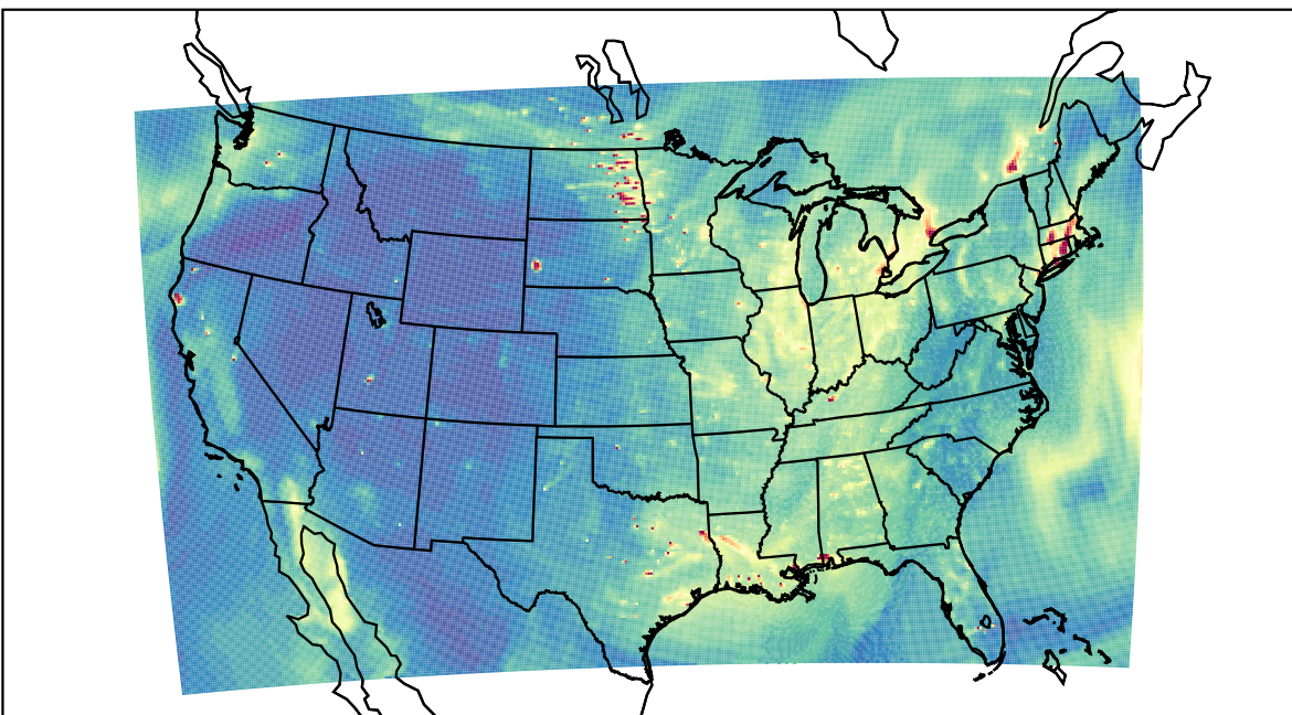
WRF 2022-10-31_23:00:00
