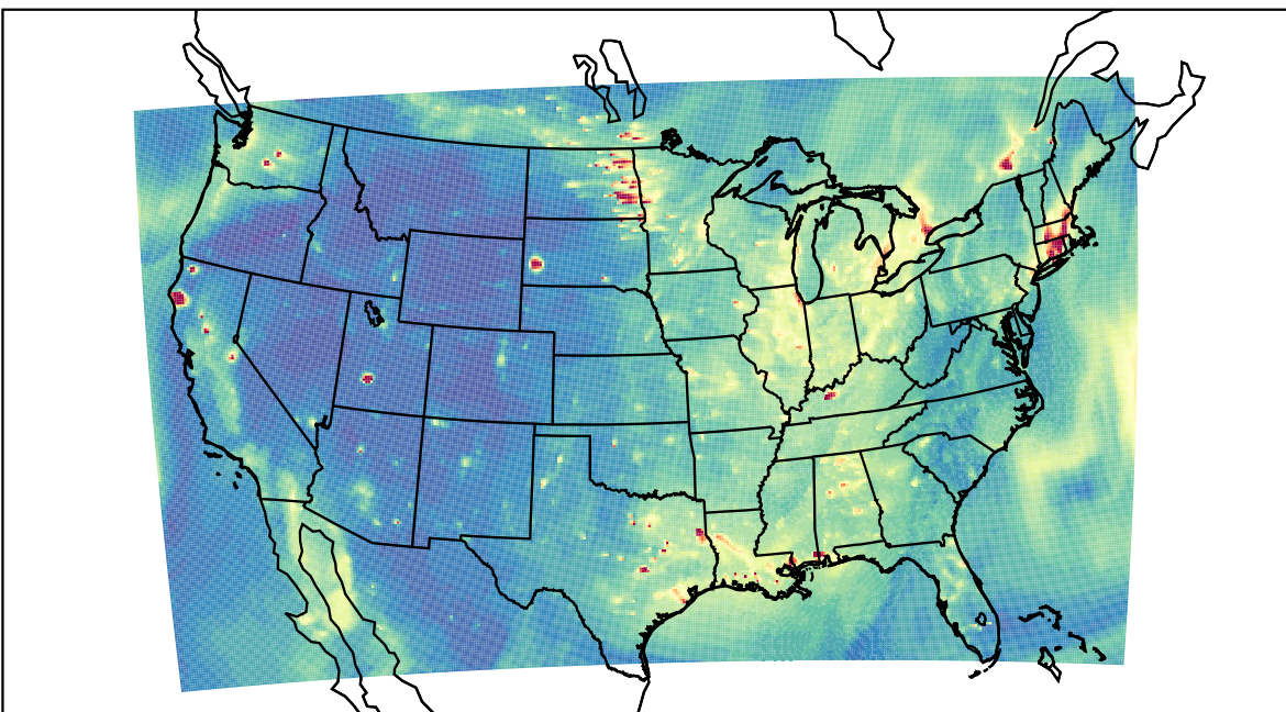
WRF 2022-11-01_01:00:00
