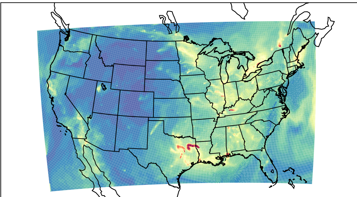
WRF 2022-11-01_11:00:00
