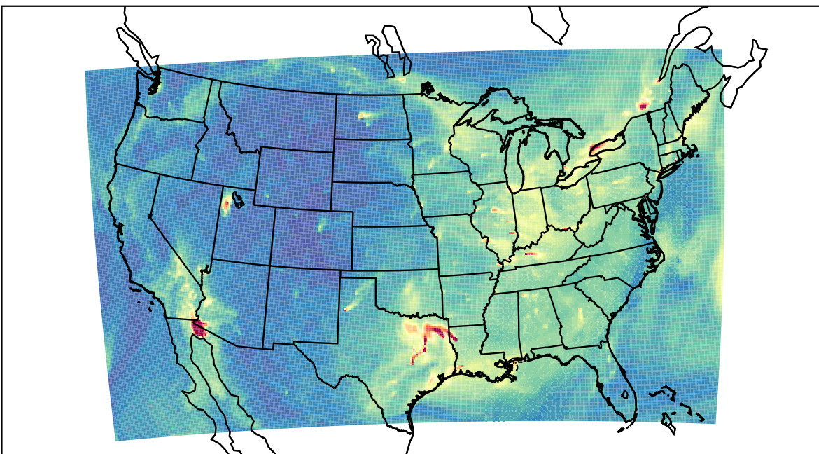
WRF 2022-11-01_16:00:00
