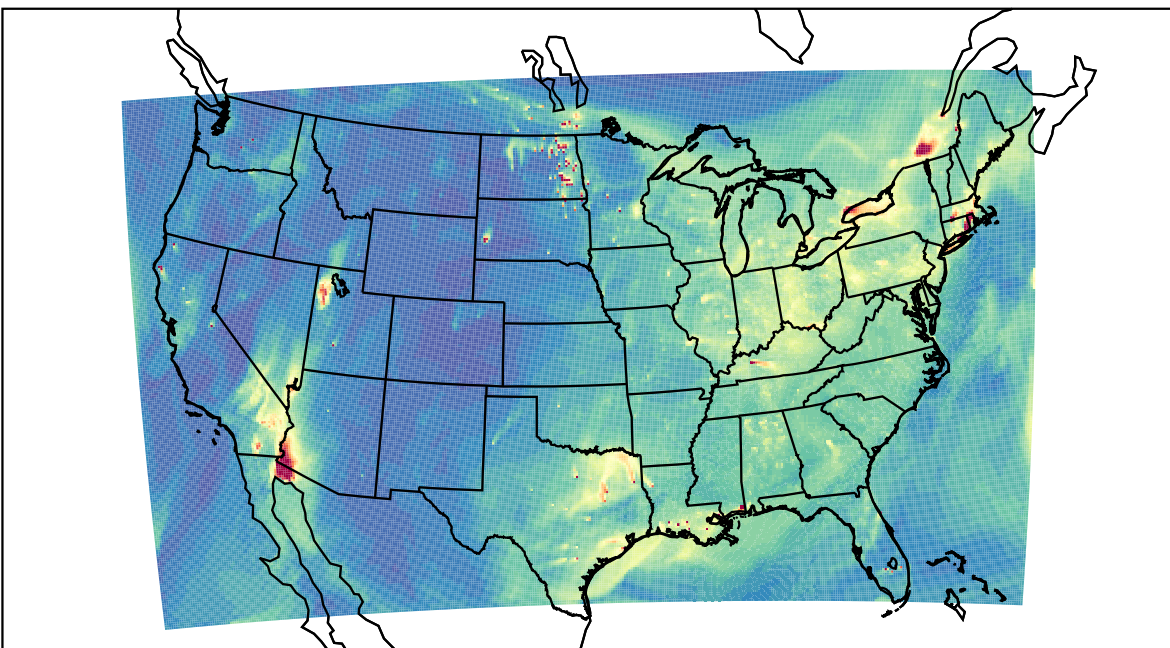
WRF 2022-11-01_22:00:00
