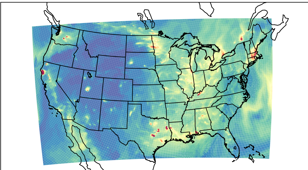
WRF 2022-11-01_04:00:00
