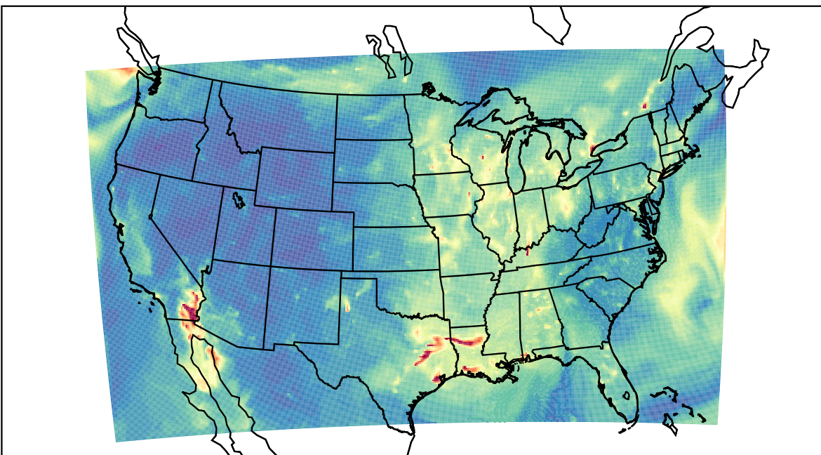
WRF 2022-10-31_13:00:00
