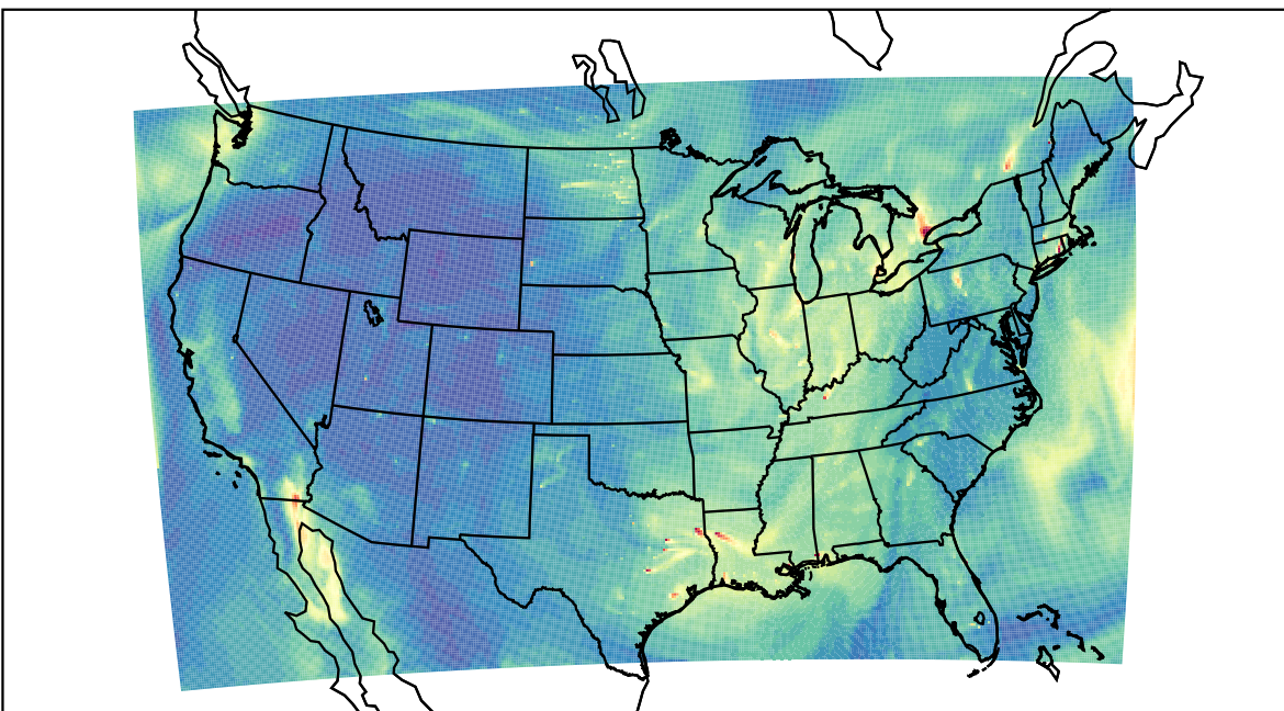
WRF 2022-10-31_19:00:00
