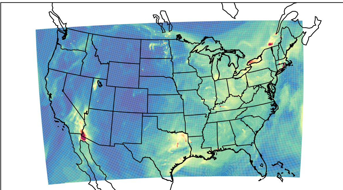
WRF 2022-11-01_20:00:00
