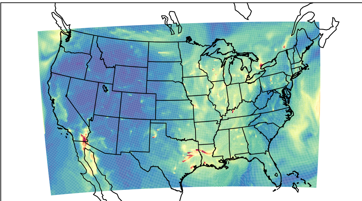
WRF 2022-10-31_16:00:00
