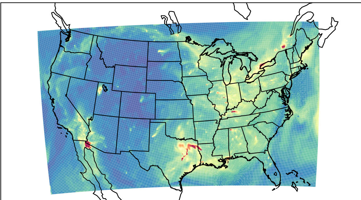
WRF 2022-11-01_15:00:00
