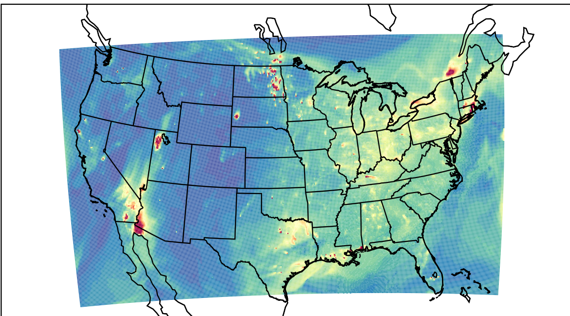
WRF 2022-11-01_23:00:00
