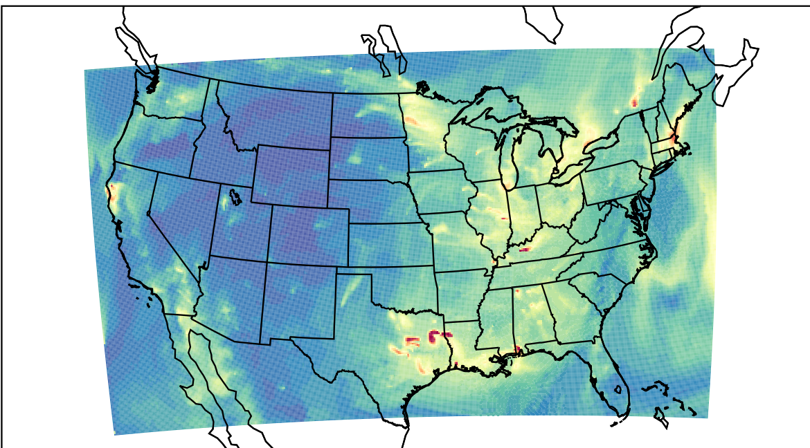
WRF 2022-11-01_08:00:00
