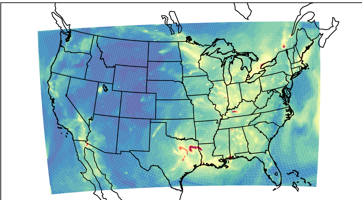
WRF 2022-11-01_12:00:00
