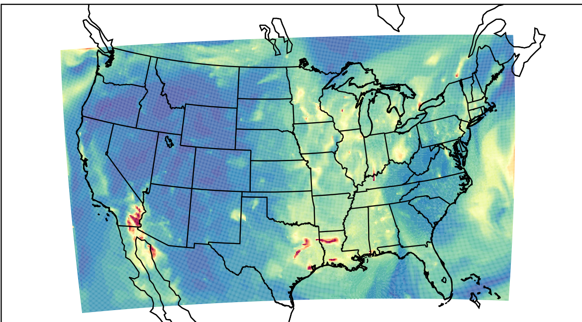
WRF 2022-10-31_10:00:00
