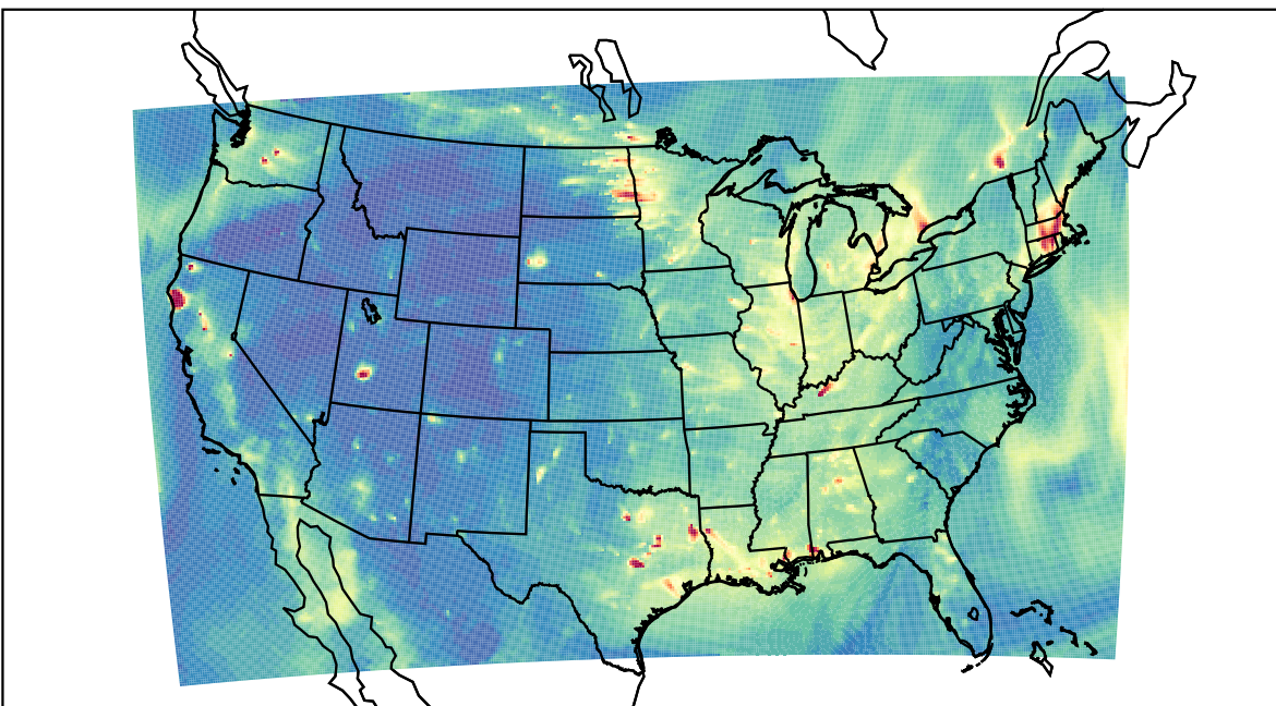
WRF 2022-11-01_03:00:00
