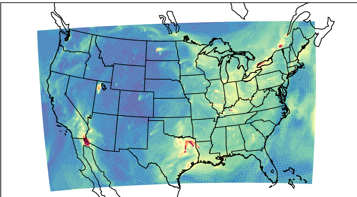
WRF 2022-11-01_17:00:00
