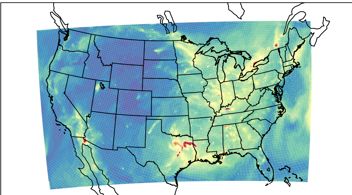
WRF 2022-11-01_13:00:00
