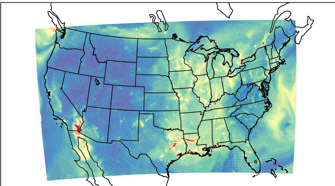
WRF 2022-10-31_14:00:00
