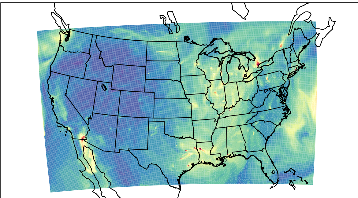
WRF 2022-10-31_18:00:00
