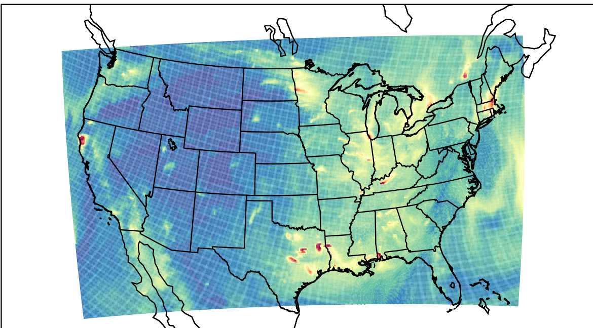
WRF 2022-11-01_06:00:00
