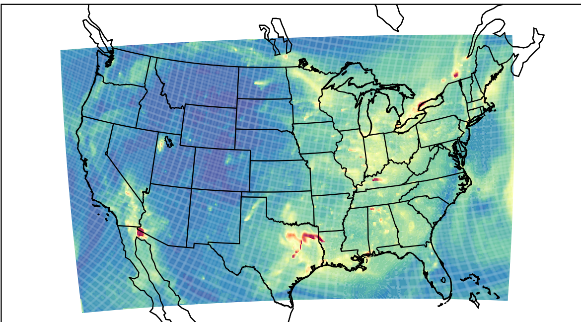
WRF 2022-11-01_14:00:00
