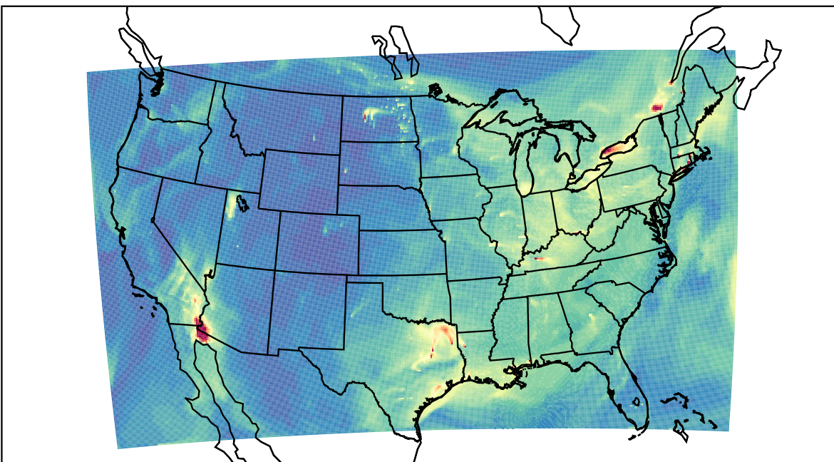
WRF 2022-11-01_19:00:00
