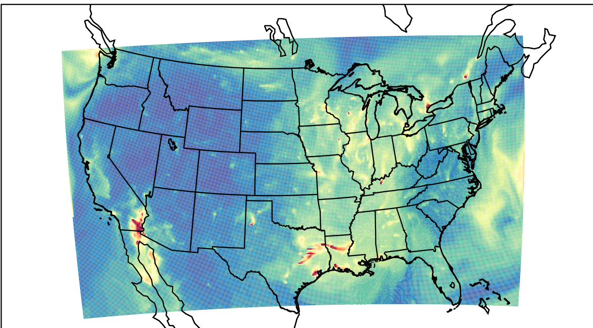
WRF 2022-10-31_15:00:00
