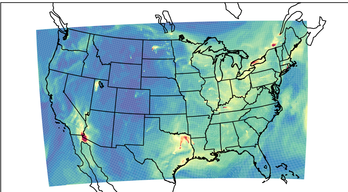
WRF 2022-11-01_18:00:00
