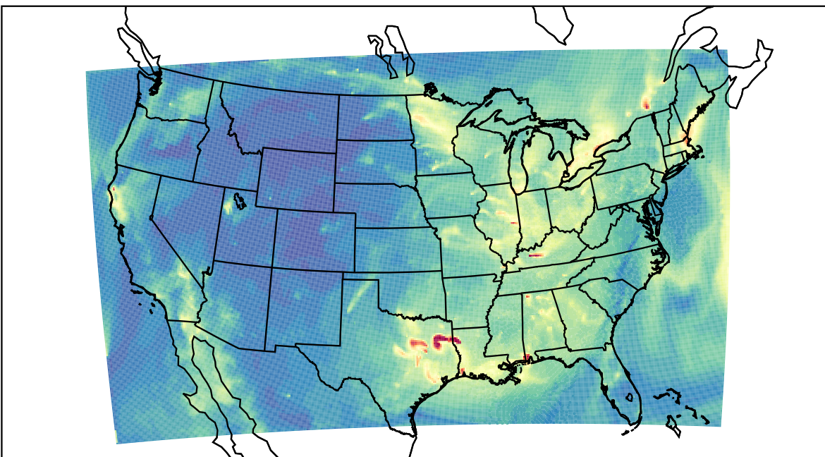
WRF 2022-11-01_10:00:00
