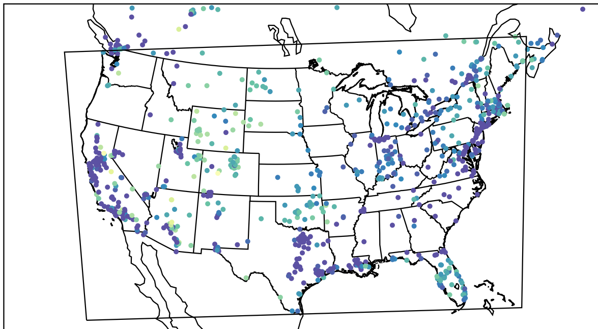
AirNOW (2022-11-18_10:00:00)
