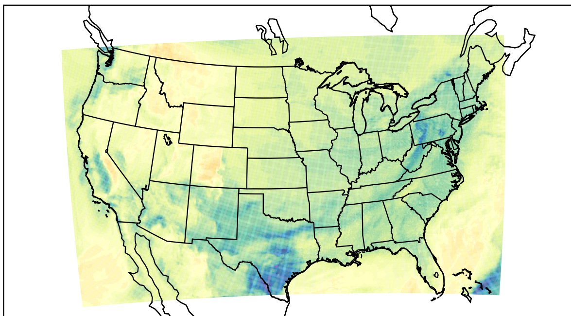
WRF (2022-11-18_19:00:00)
