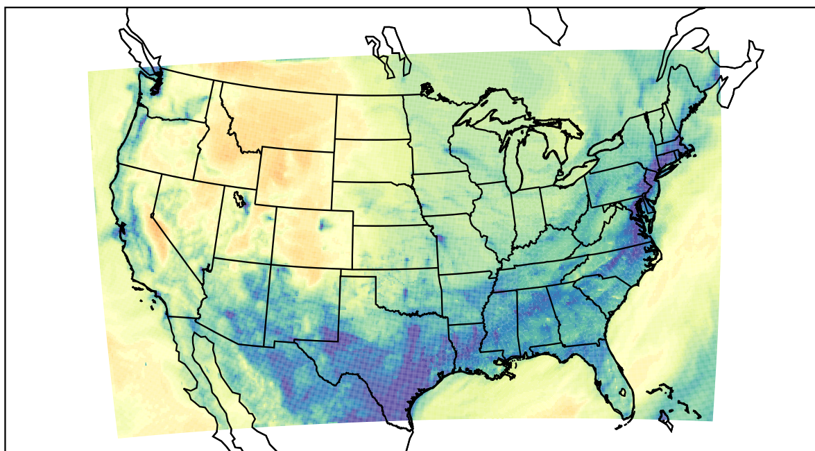
WRF (2022-11-20_04:00:00)
