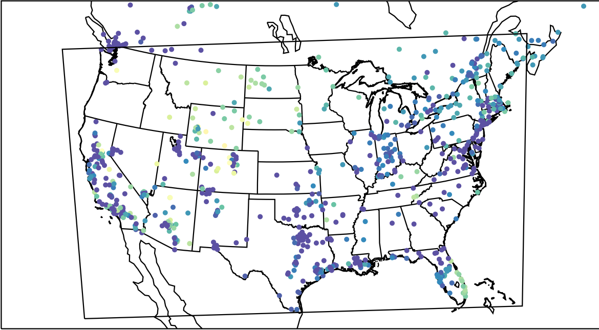
AirNOW (2022-11-21_10:00:00)
