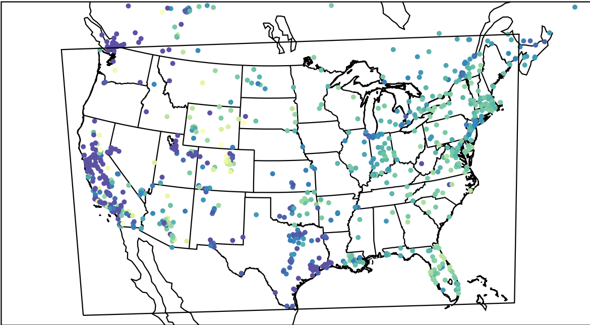
AirNOW (2022-11-21_16:00:00)
