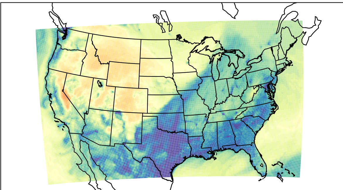
WRF (2022-11-21_13:00:00)
