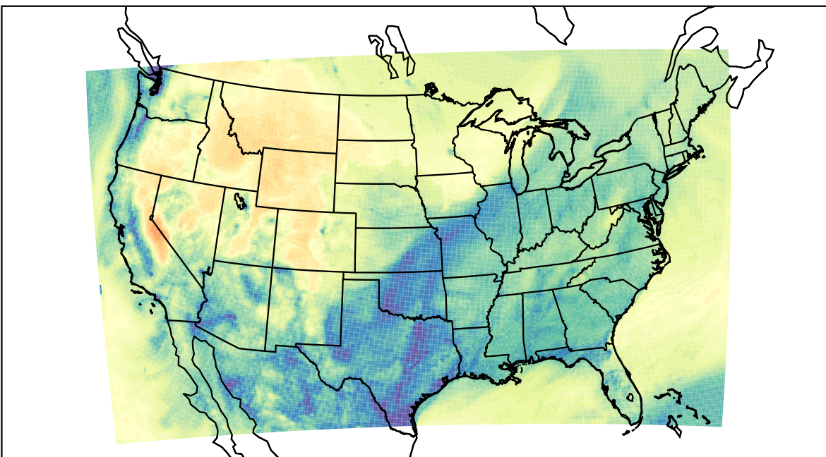
WRF (2022-11-21_16:00:00)
