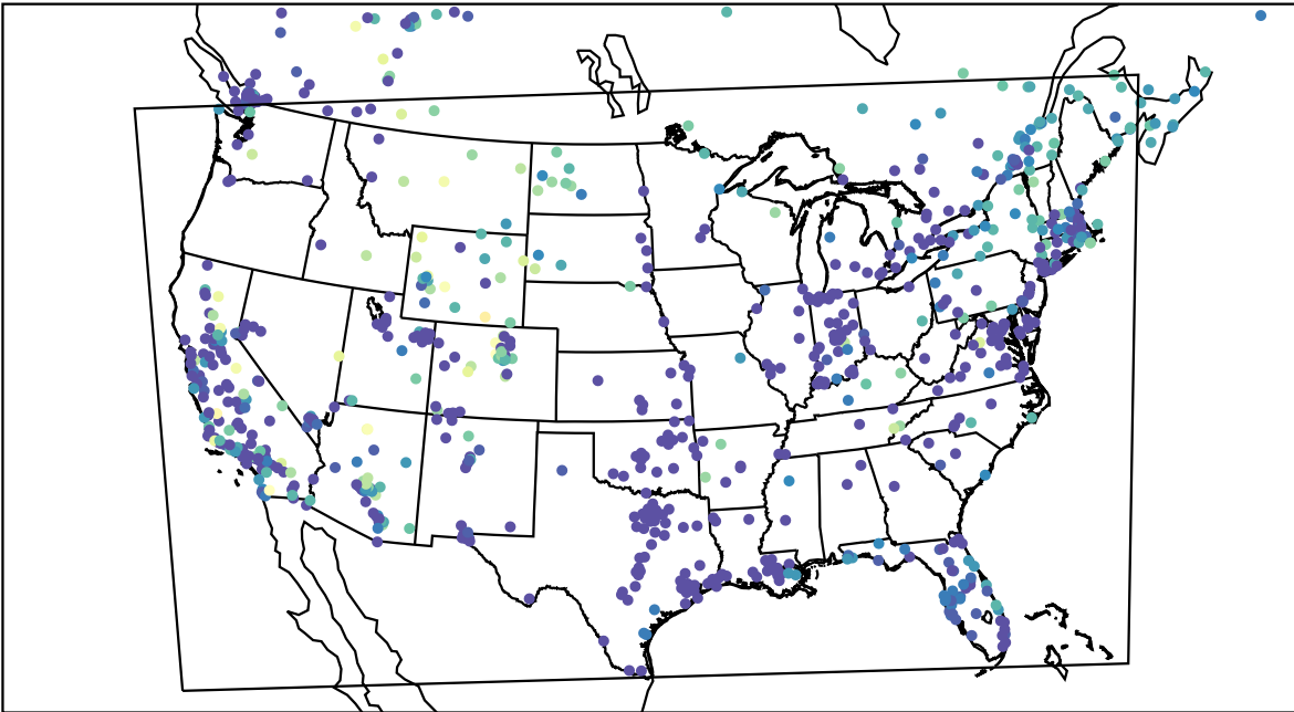
AirNOW (2022-11-22_13:00:00)
