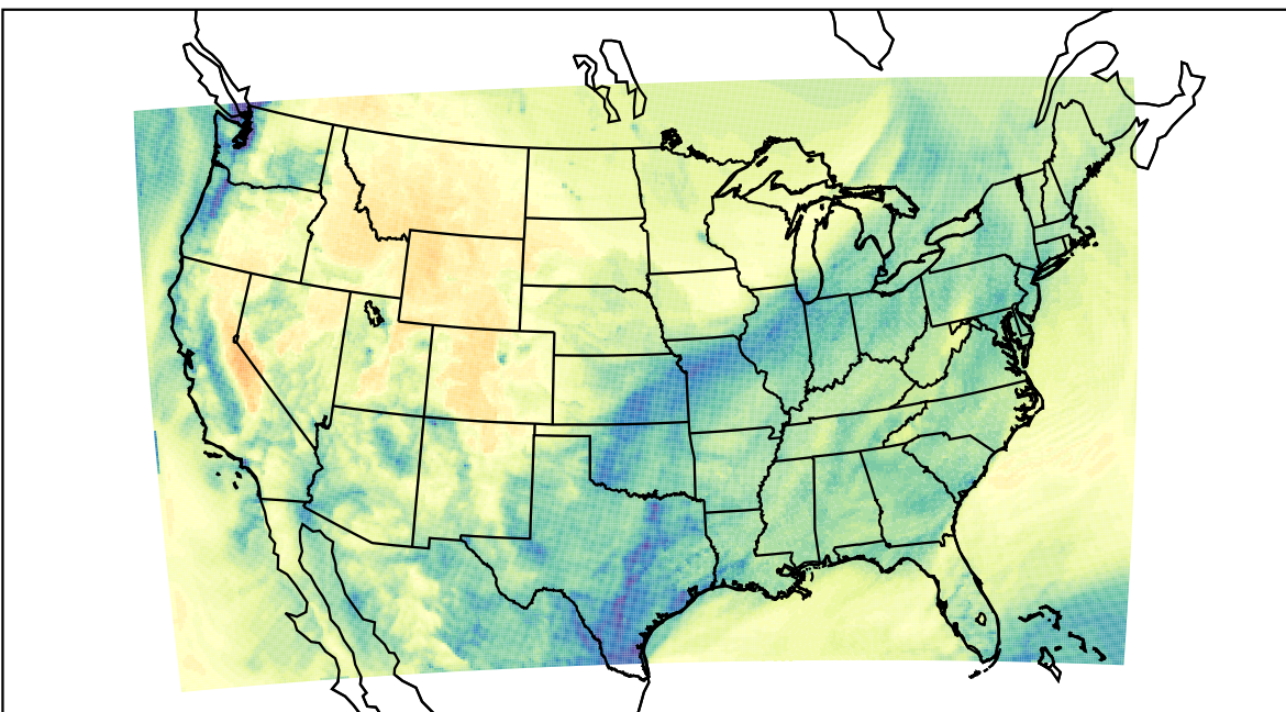
WRF (2022-11-21_18:00:00)
