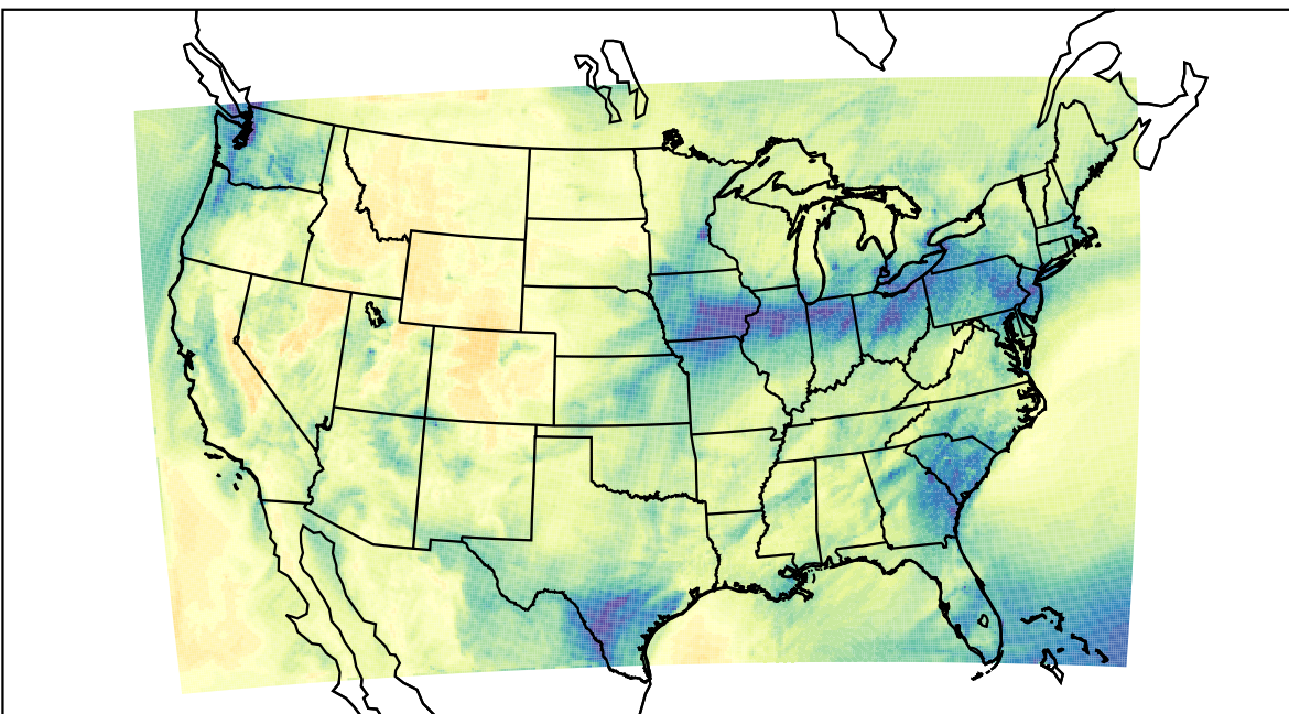
WRF (2022-11-22_20:00:00)
