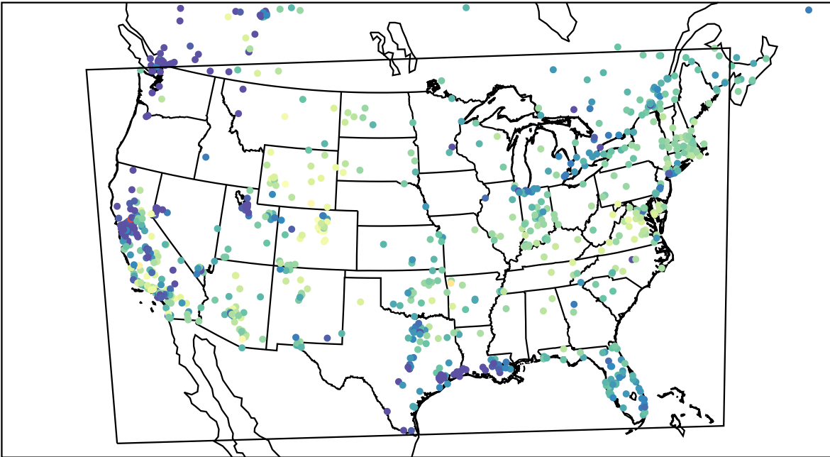
AirNOW (2022-11-22_18:00:00)
