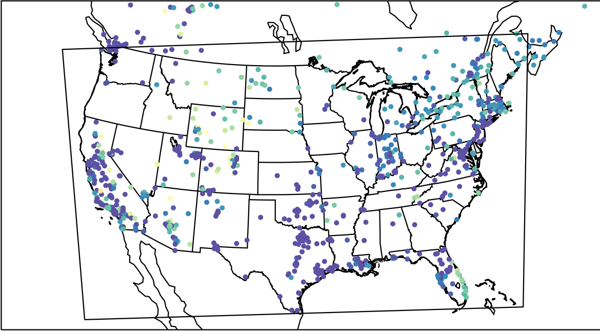
AirNOW (2022-11-21_13:00:00)
