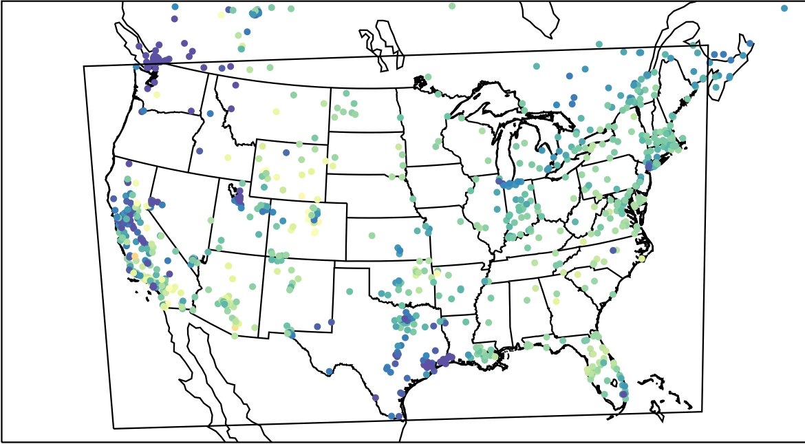
AirNOW (2022-11-21_18:00:00)
