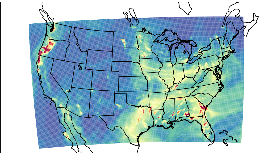
WRF 2022-12-09_04:00:00
