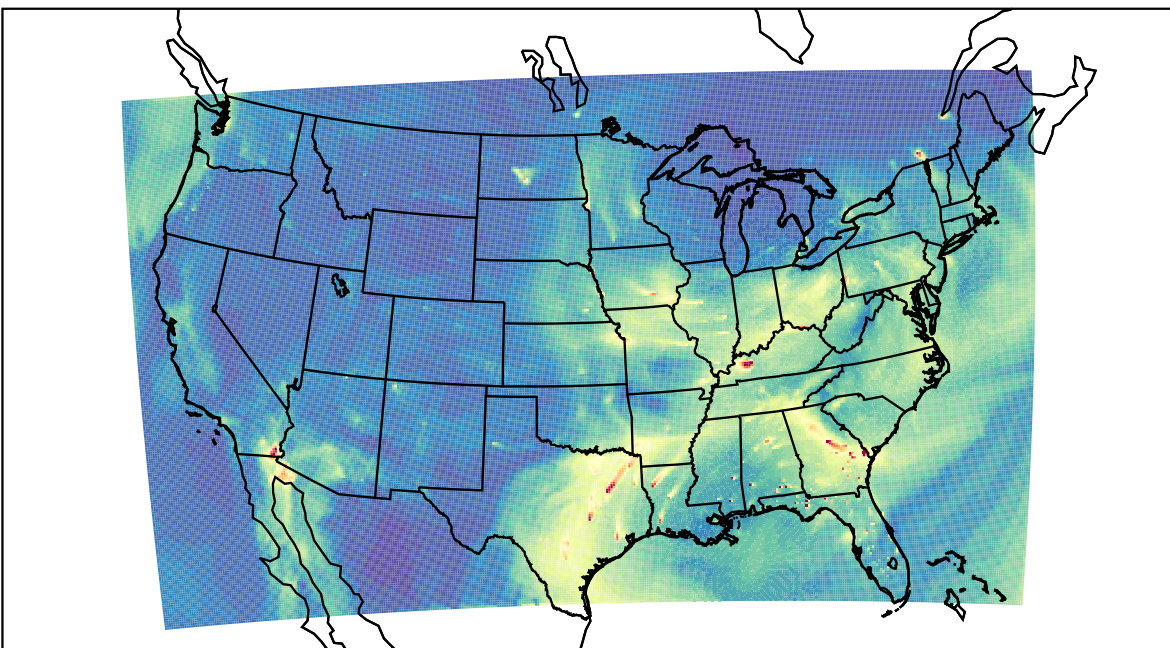
WRF 2022-12-08_18:00:00
