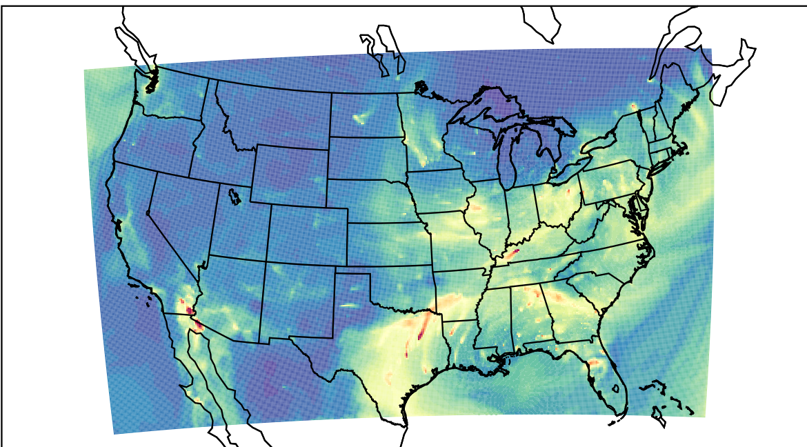
WRF 2022-12-08_14:00:00
