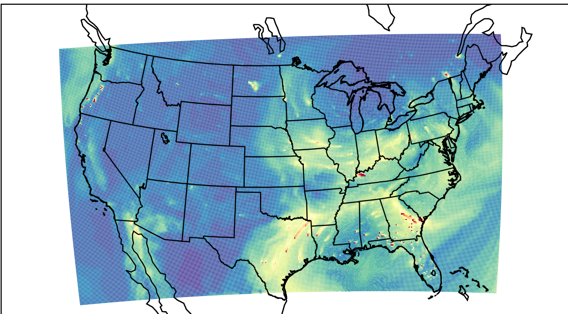
WRF 2022-12-08_20:00:00
