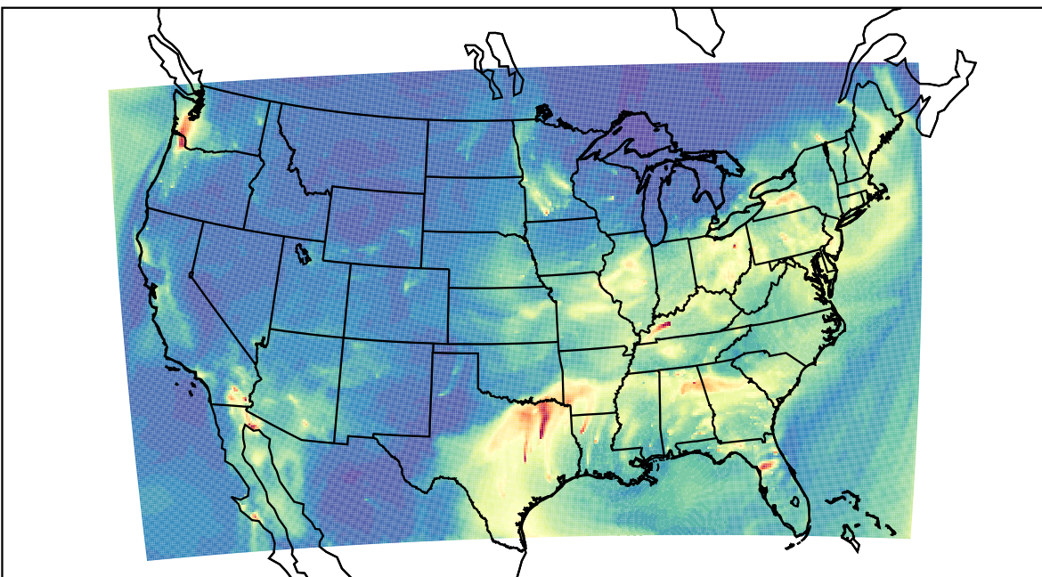
WRF 2022-12-08_10:00:00
