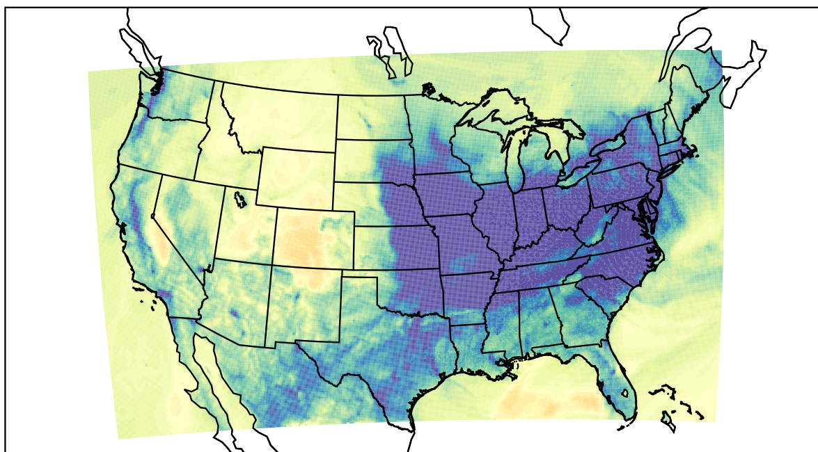
WRF (2022-12-09_04:00:00)
