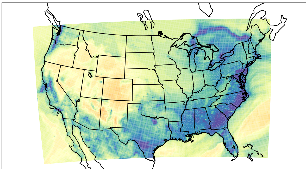
WRF (2022-12-18_10:00:00)
