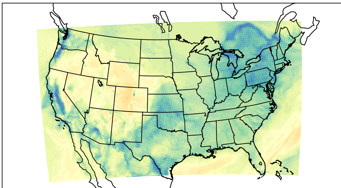
WRF (2022-12-18_18:00:00)
