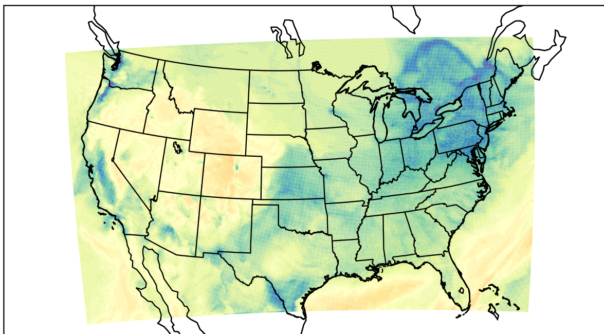
WRF (2022-12-18_20:00:00)
