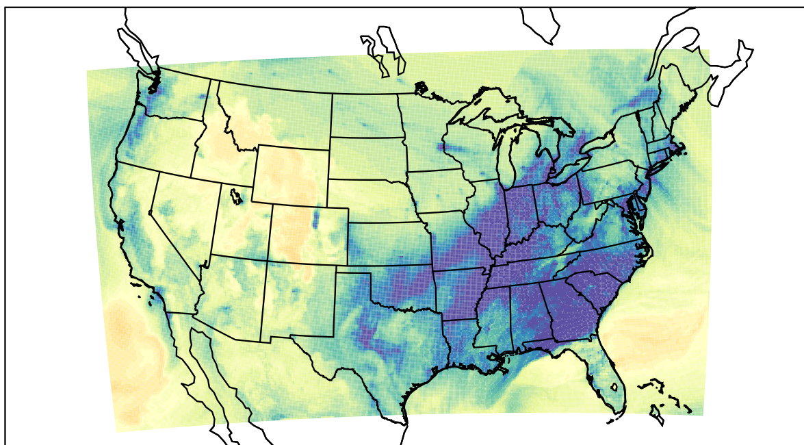
WRF (2022-12-20_23:00:00)
