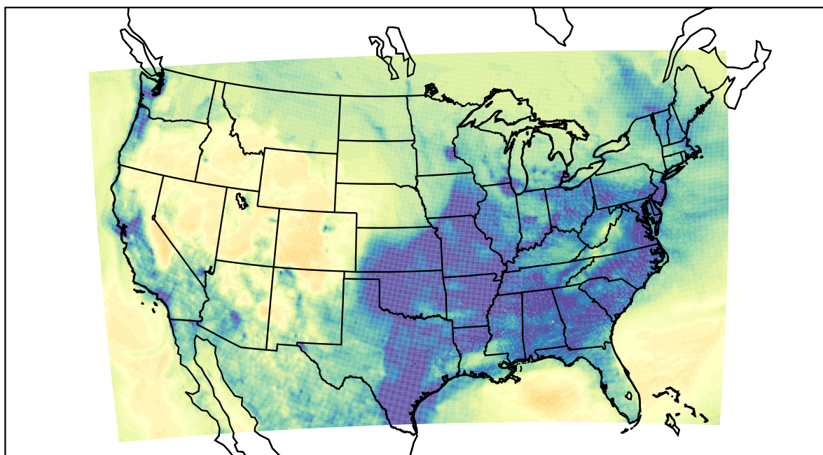
WRF (2022-12-20_04:00:00)
