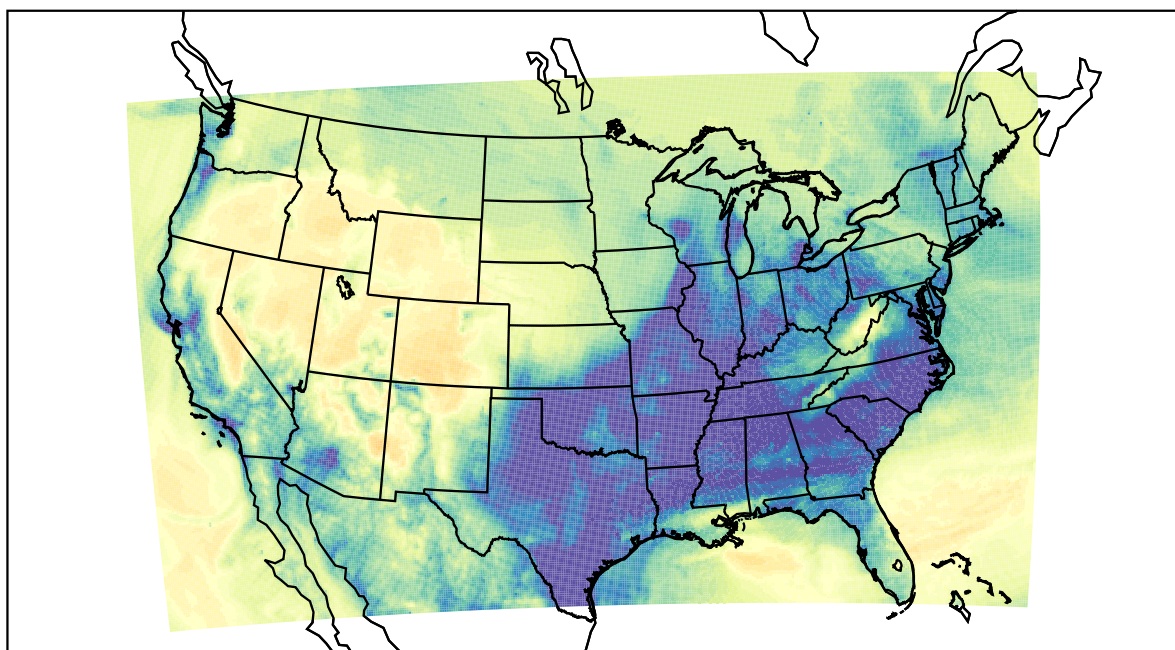
WRF (2022-12-20_10:00:00)
