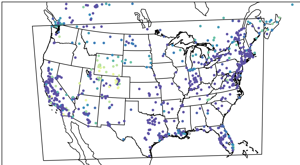
AirNOW (2022-12-21_13:00:00)
