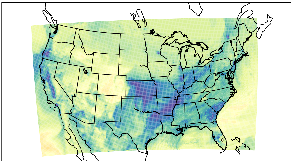
WRF (2022-12-21_18:00:00)
