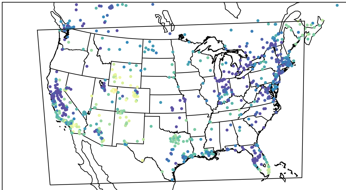
AirNOW (2022-12-20_20:00:00)
