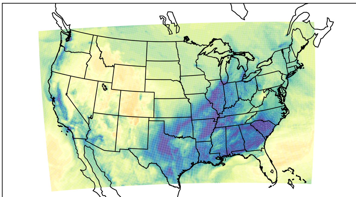
WRF (2022-12-20_18:00:00)
