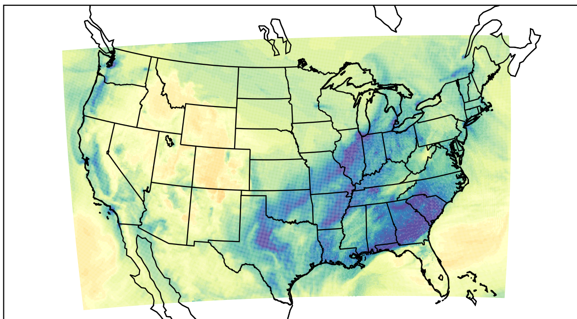
WRF (2022-12-20_20:00:00)
