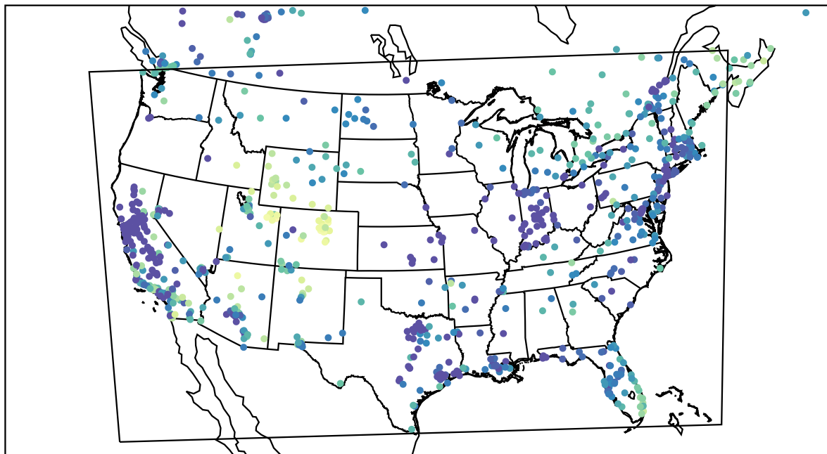
AirNOW (2022-12-21_18:00:00)
