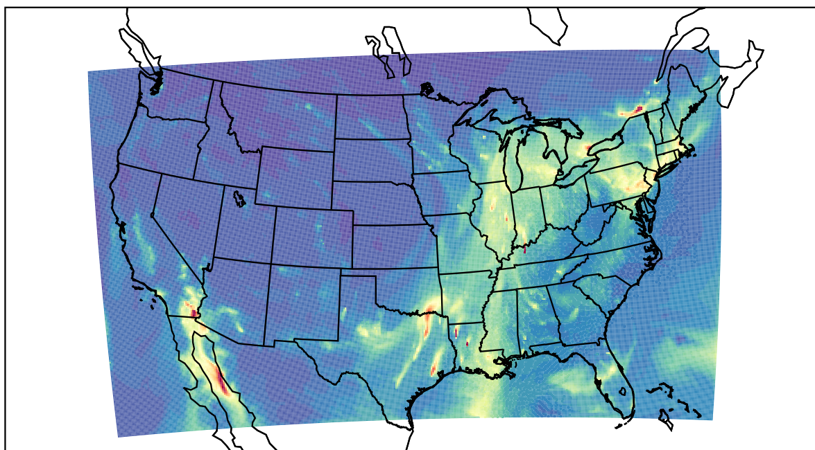
WRF 2022-12-22_13:00:00
