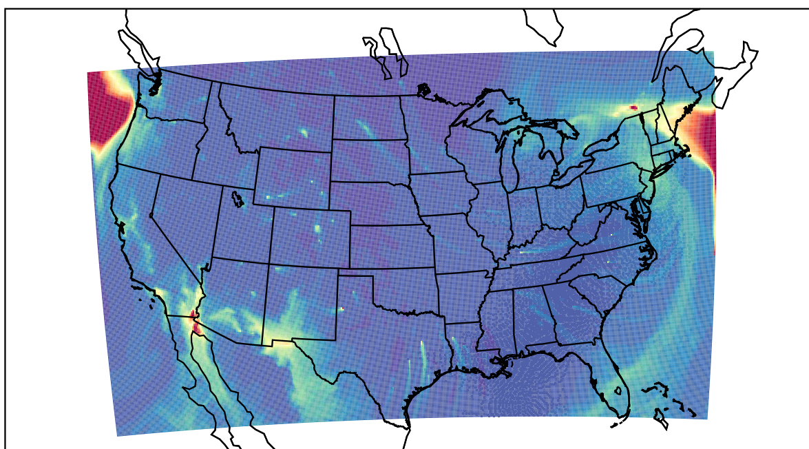
WRF 2022-12-23_18:00:00
