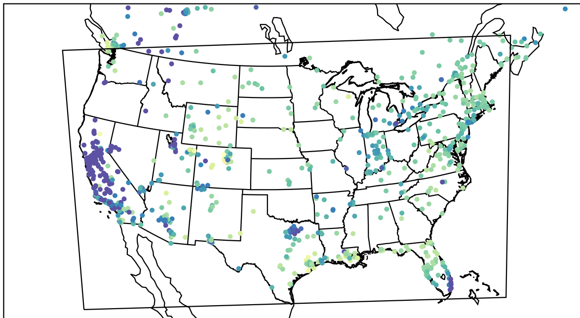
AirNOW (2022-12-26_18:00:00)
