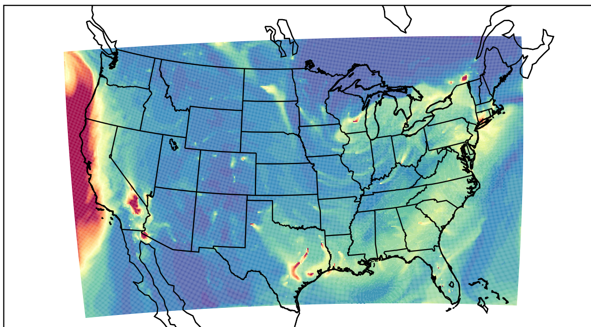
WRF 2023-01-05_18:00:00
