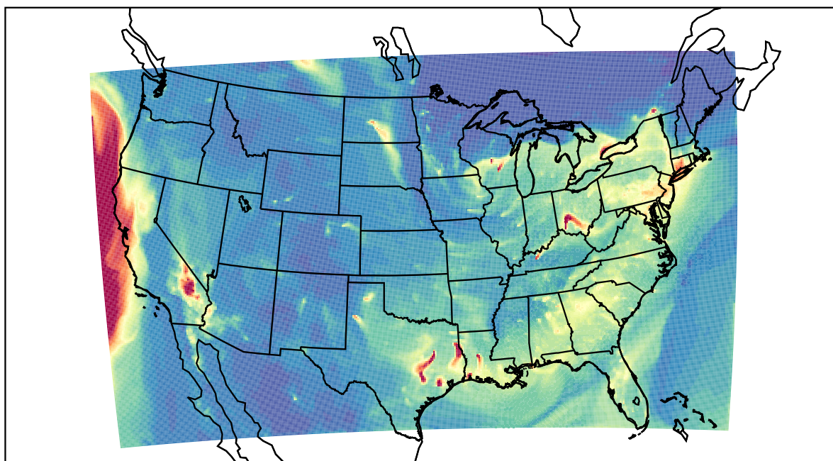
WRF 2023-01-05_13:00:00
