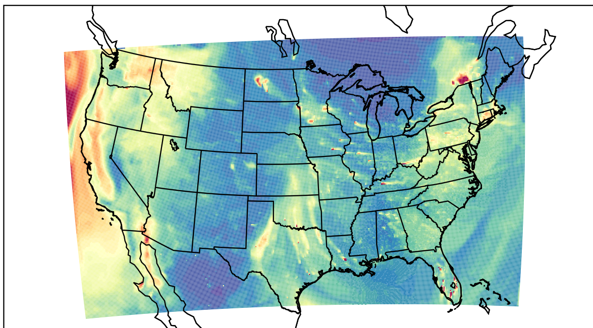
WRF 2023-01-06_23:00:00
