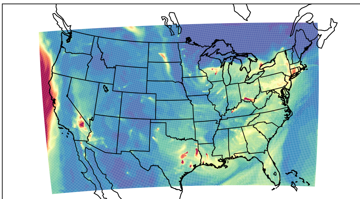
WRF 2023-01-05_10:00:00
