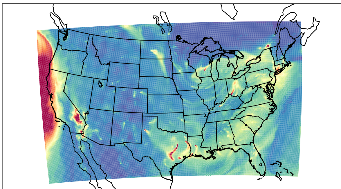
WRF 2023-01-05_16:00:00
