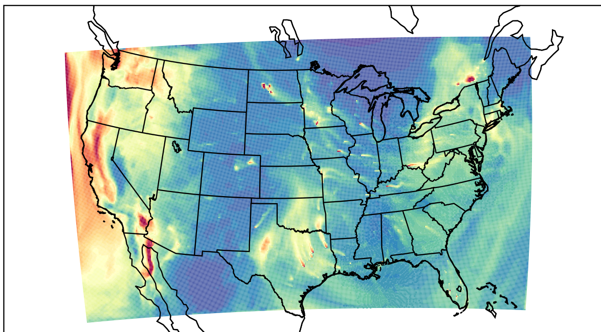
WRF 2023-01-06_18:00:00
