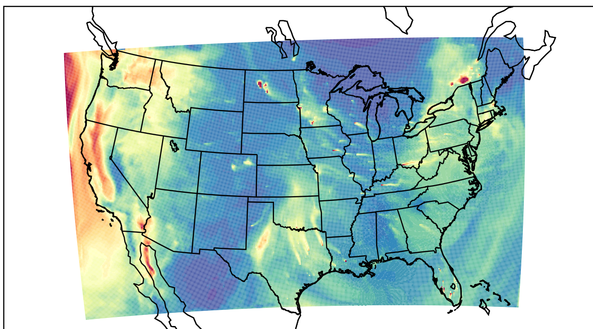
WRF 2023-01-06_20:00:00
