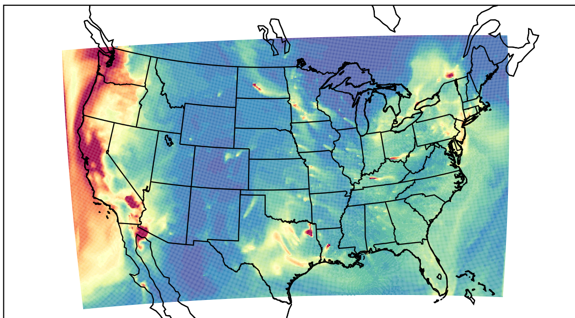
WRF 2023-01-06_10:00:00
