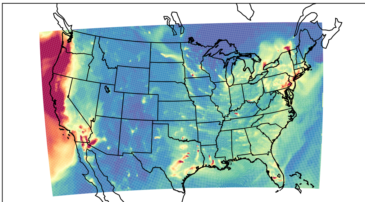
WRF 2023-01-06_03:00:00
