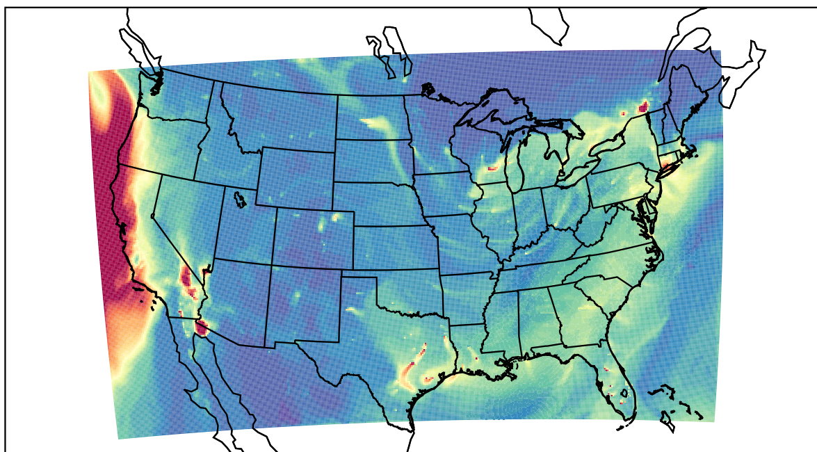
WRF 2023-01-05_20:00:00
