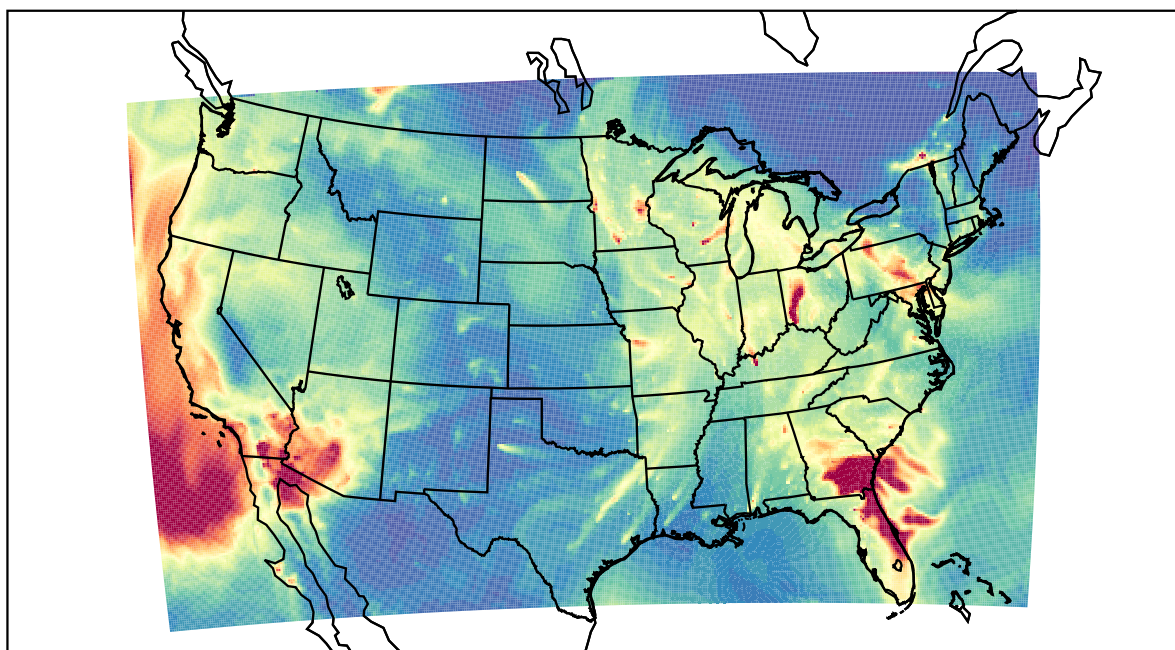
WRF 2023-01-11_12:00:00
