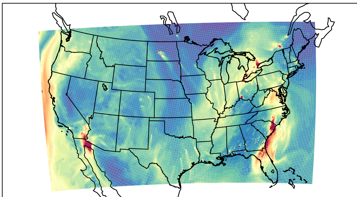
WRF 2023-01-12_18:00:00
