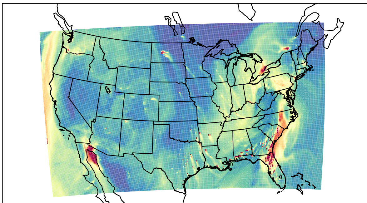
WRF 2023-01-12_23:00:00
