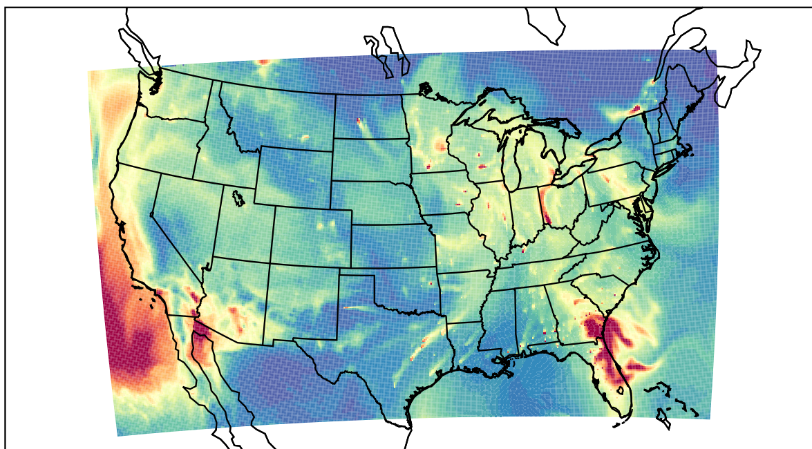
WRF 2023-01-11_17:00:00
