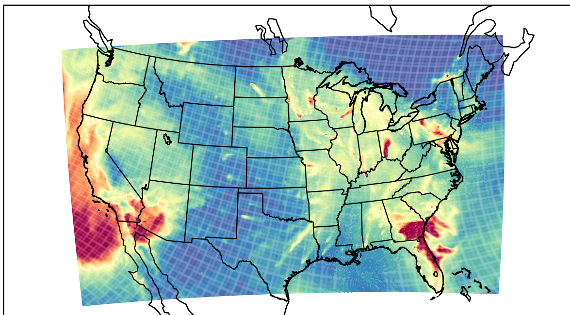
WRF 2023-01-11_11:00:00
