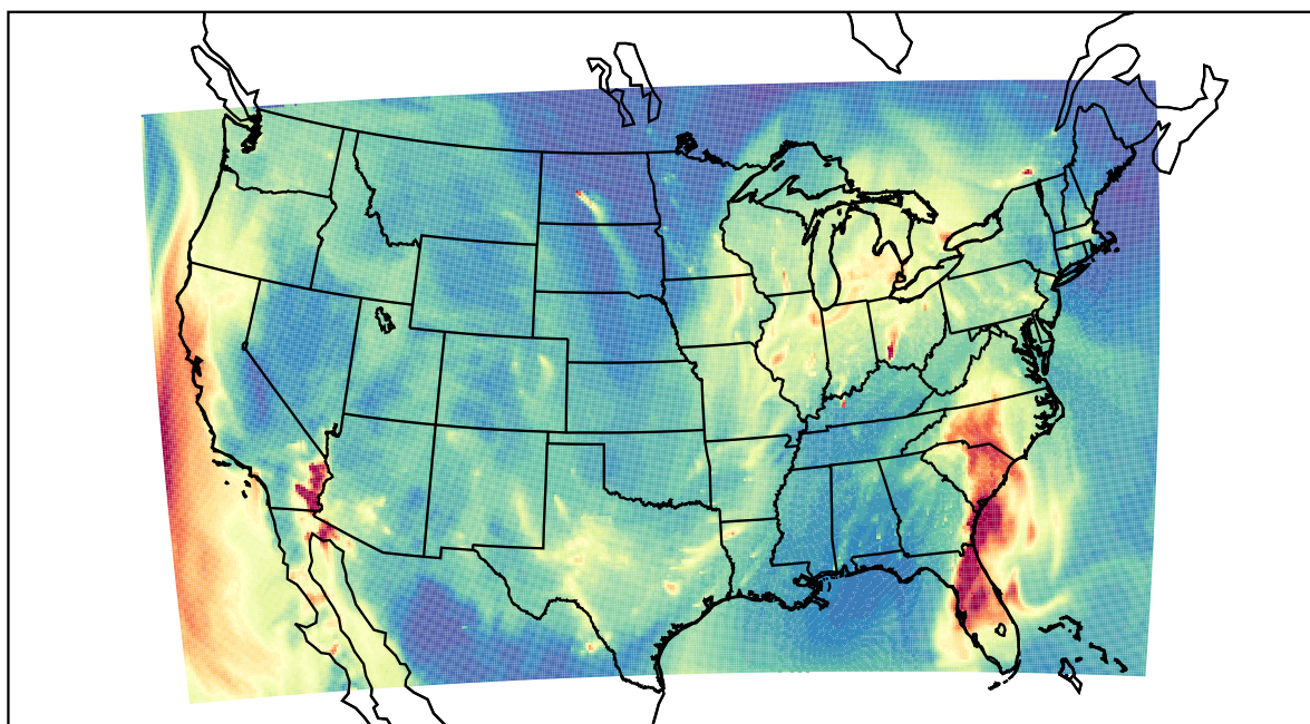
WRF 2023-01-12_10:00:00
