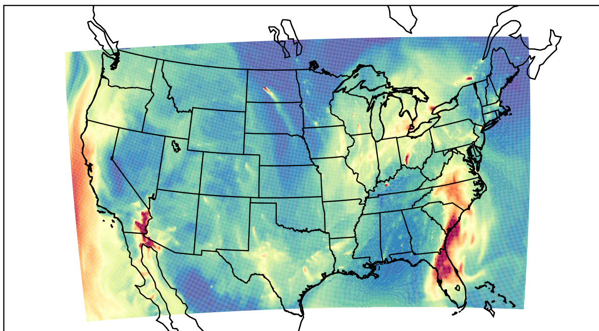
WRF 2023-01-12_13:00:00
