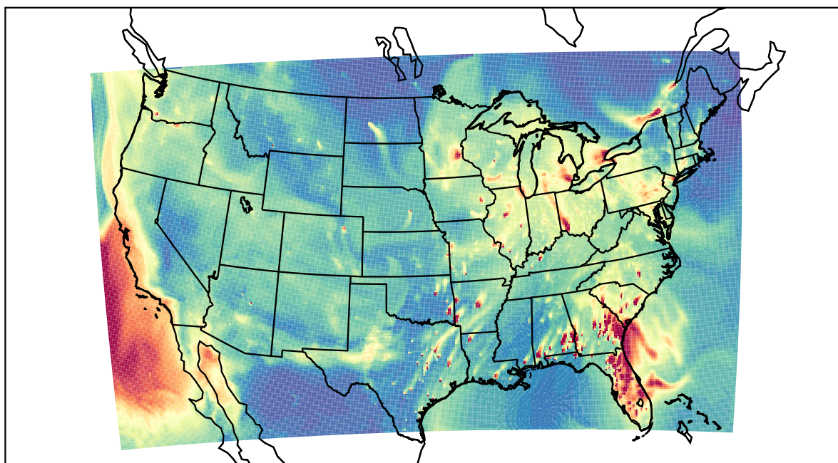
WRF 2023-01-11_23:00:00
