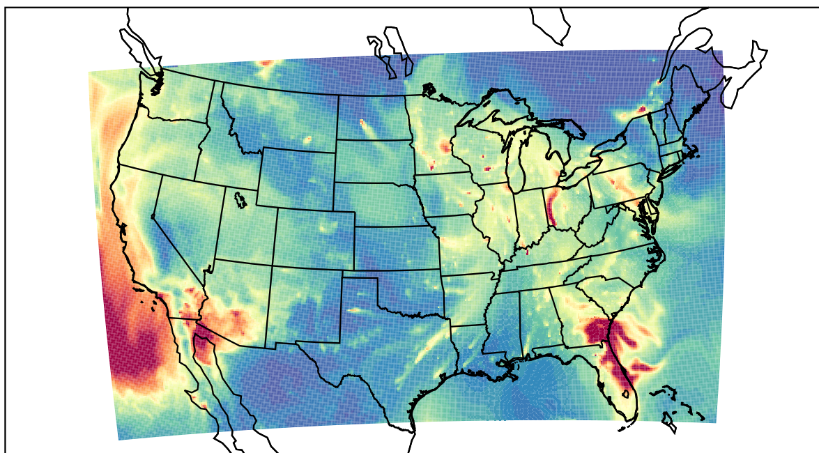
WRF 2023-01-11_15:00:00
