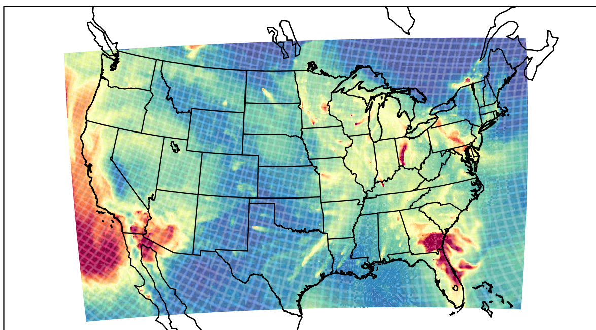
WRF 2023-01-11_13:00:00
