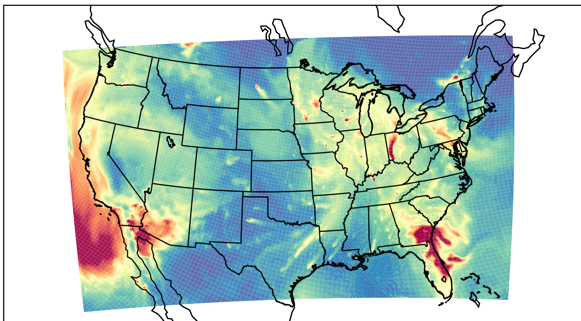
WRF 2023-01-11_14:00:00
