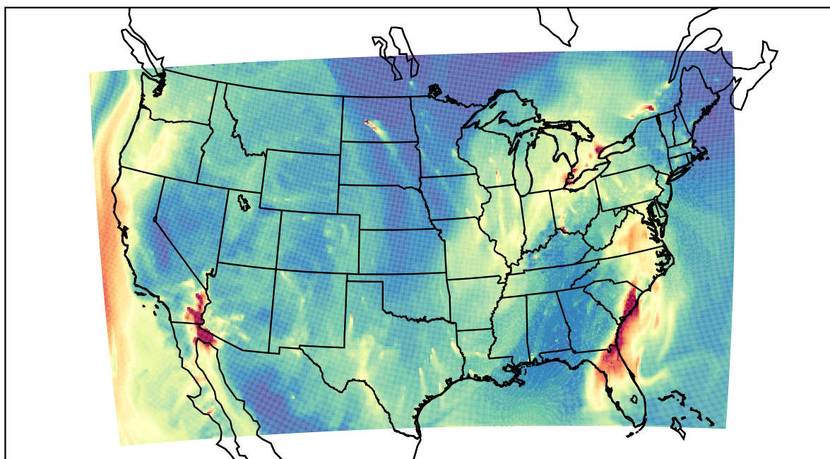
WRF 2023-01-12_16:00:00
