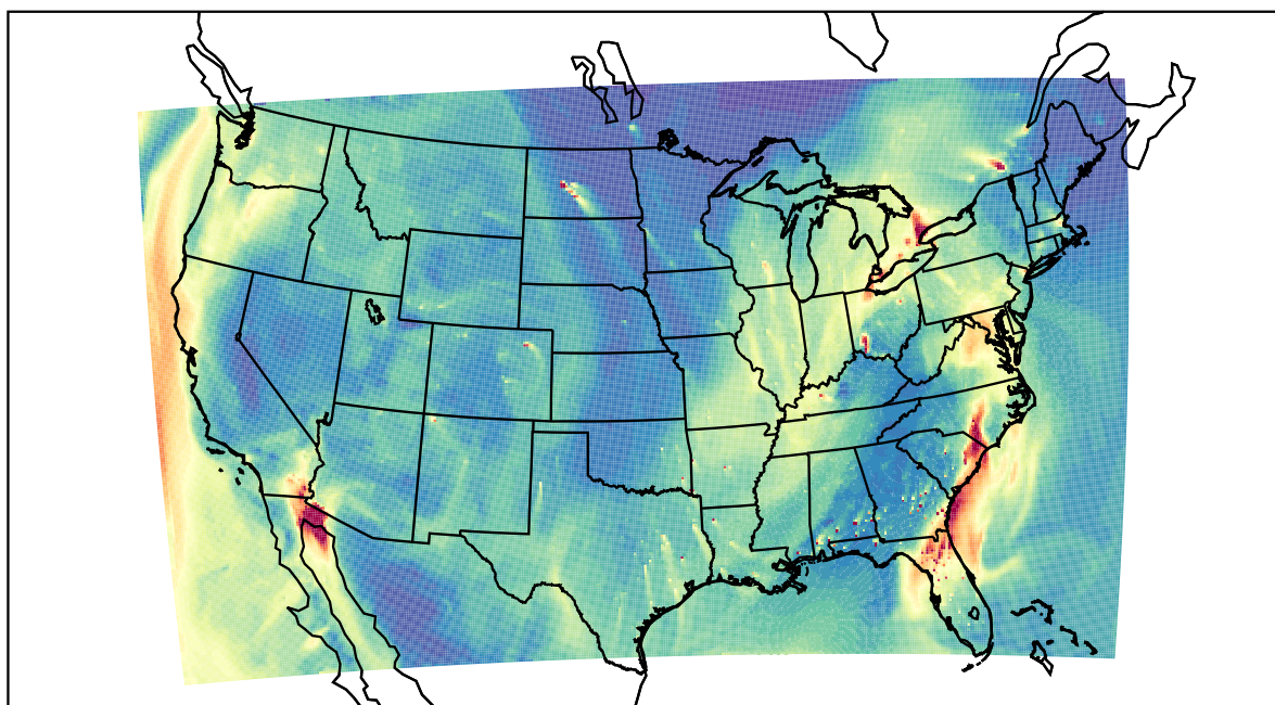
WRF 2023-01-12_19:00:00
