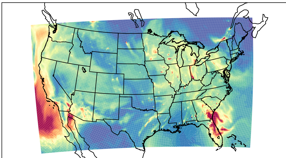
WRF 2023-01-11_18:00:00
