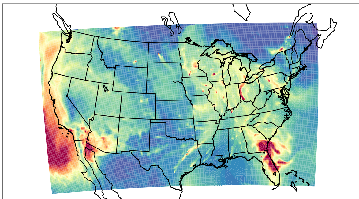
WRF 2023-01-11_16:00:00
