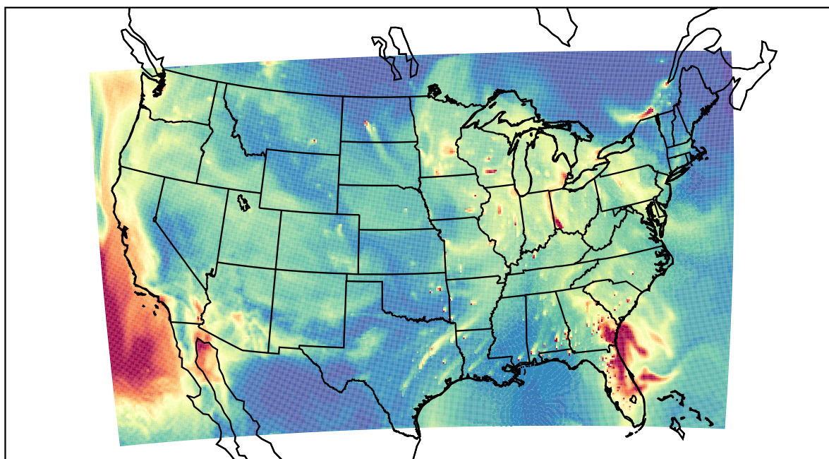
WRF 2023-01-11_19:00:00
