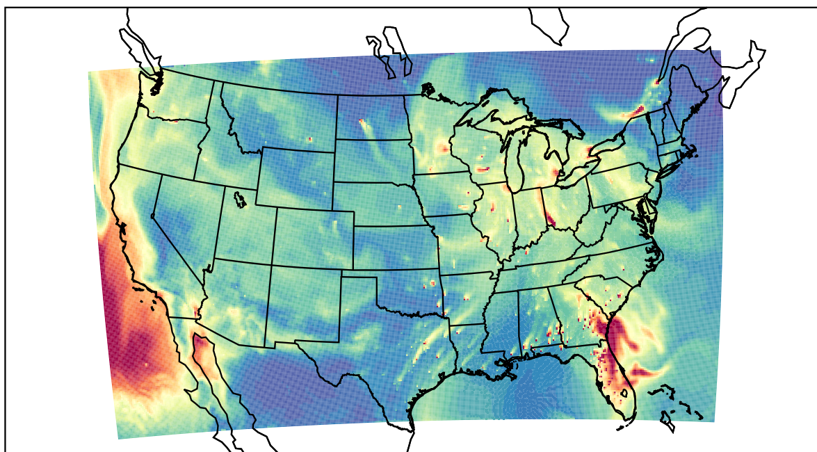
WRF 2023-01-11_20:00:00
