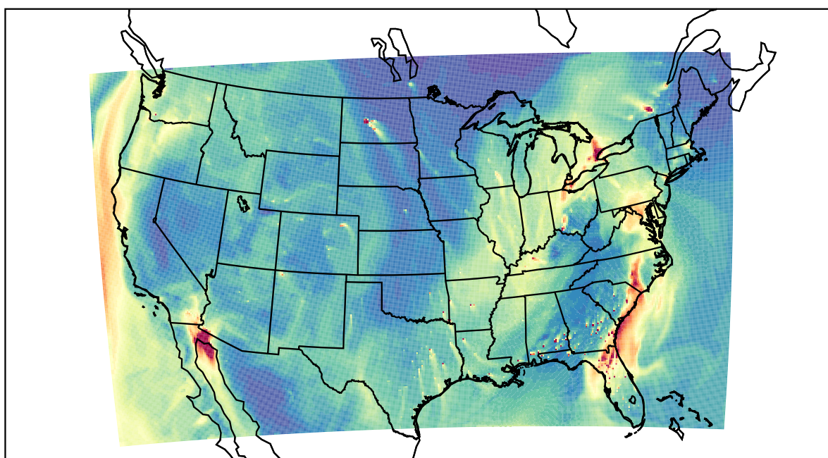
WRF 2023-01-12_20:00:00
