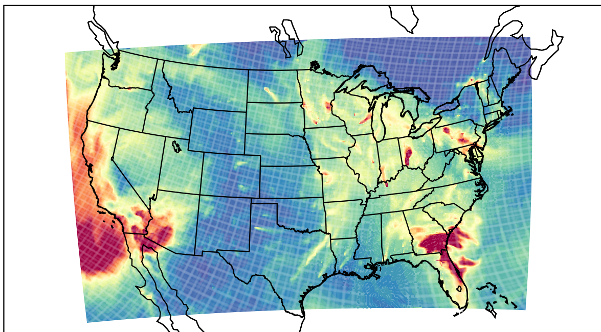
WRF 2023-01-11_10:00:00
