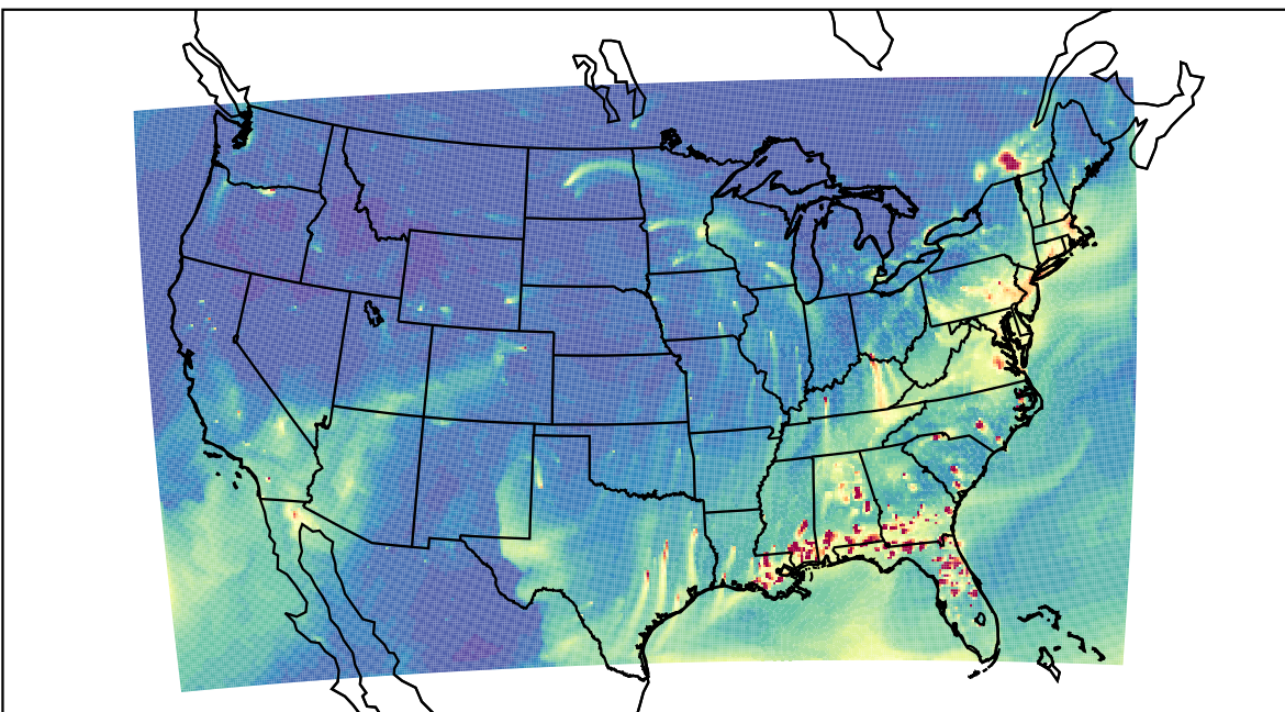
WRF 2023-01-30_23:00:00
