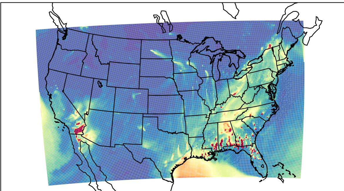
WRF 2023-01-29_22:00:00
