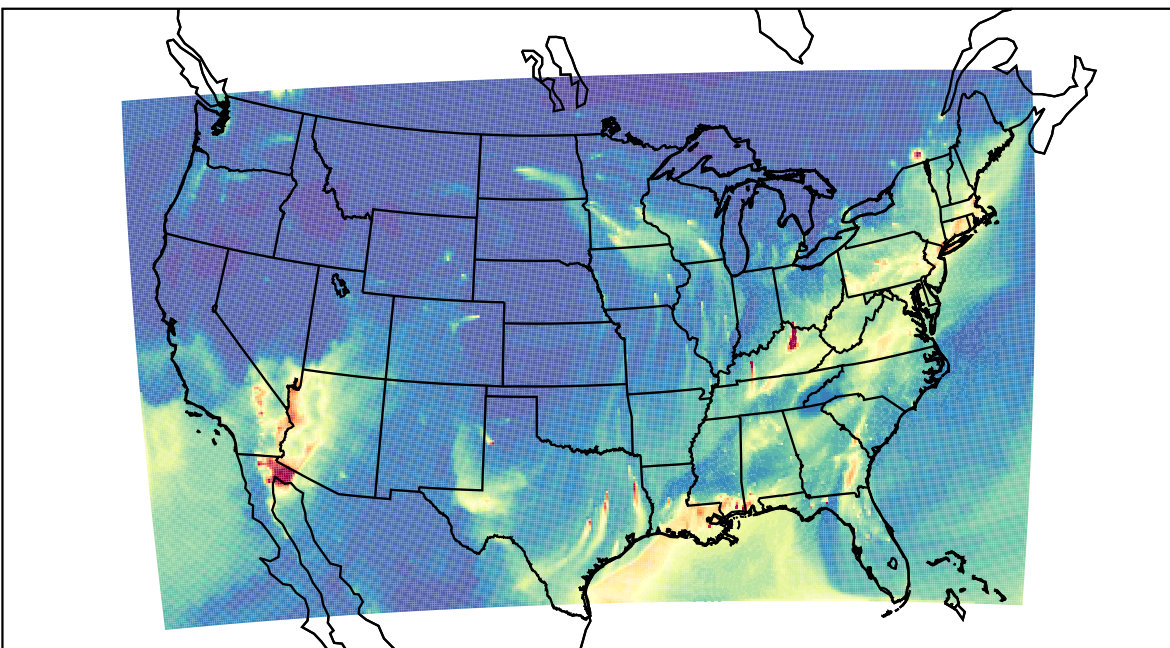
WRF 2023-01-30_10:00:00
