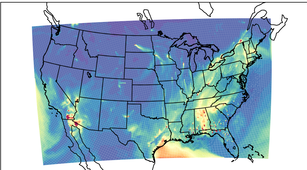
WRF 2023-01-29_18:00:00
