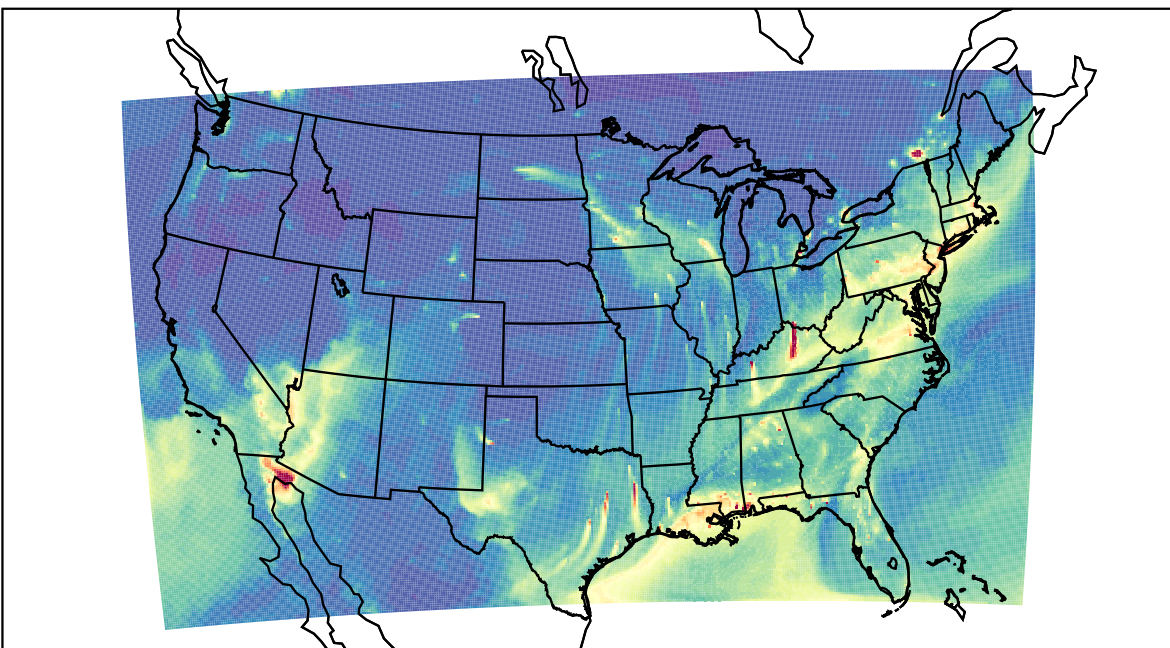
WRF 2023-01-30_13:00:00
