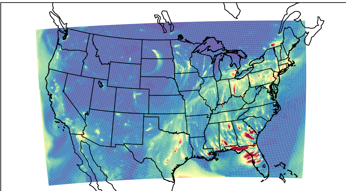
WRF 2023-01-29_03:00:00
