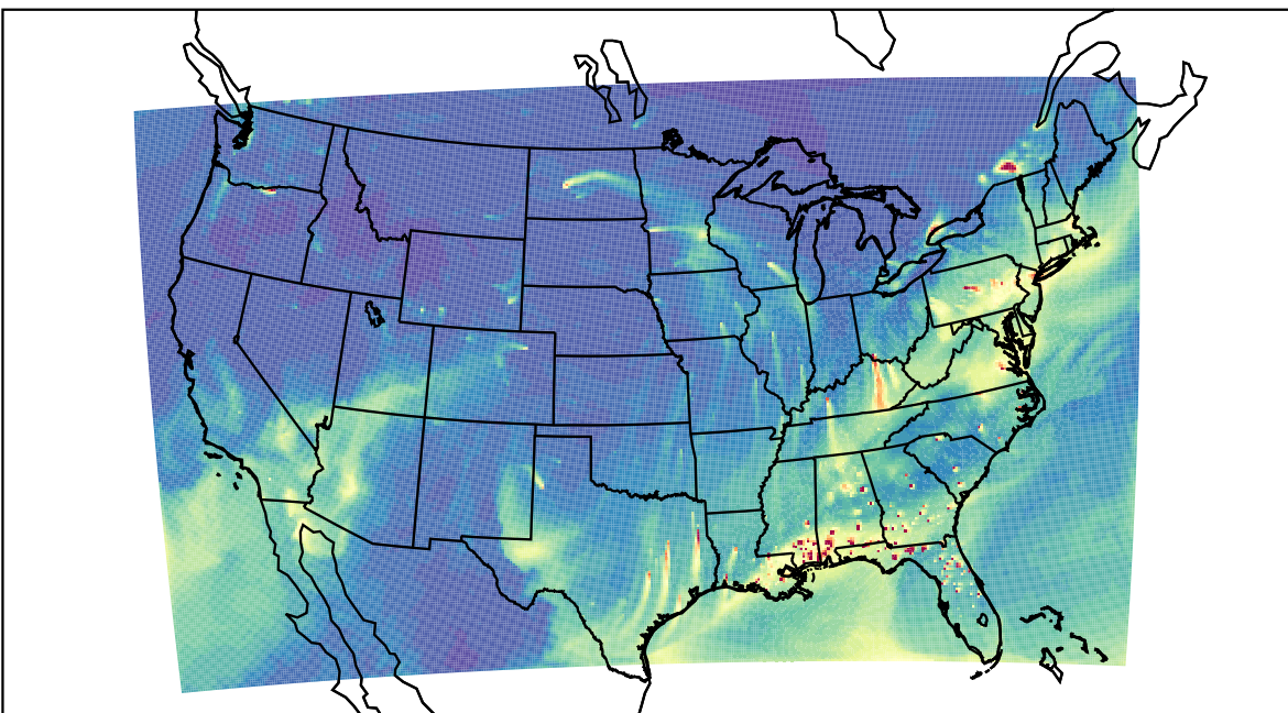
WRF 2023-01-30_19:00:00
