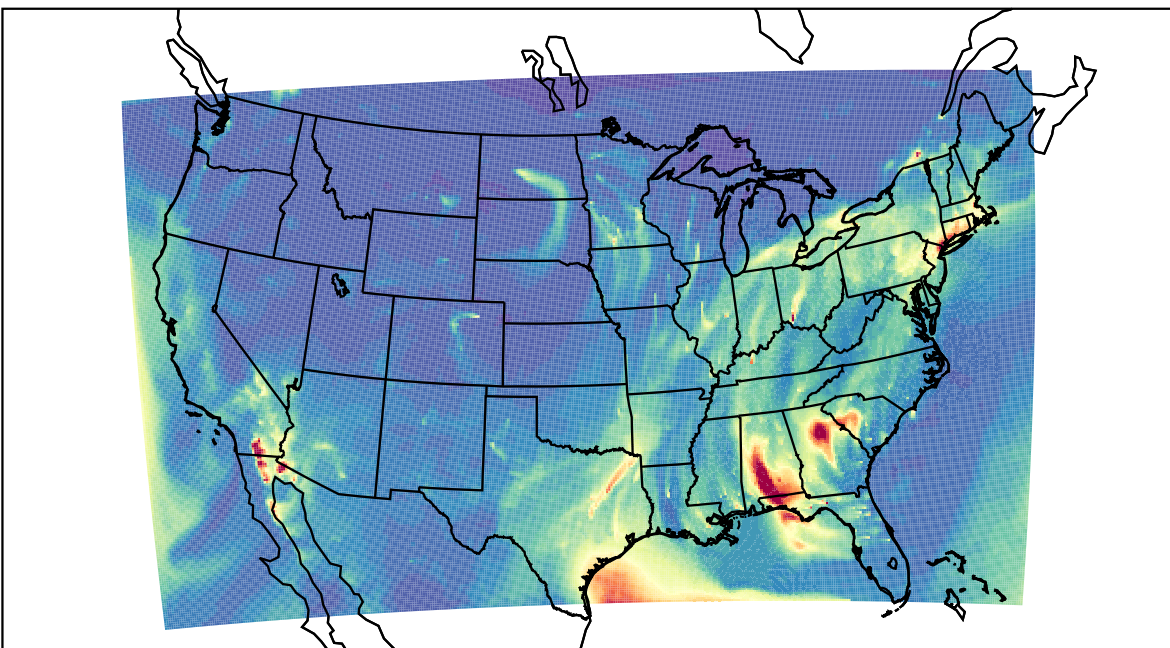
WRF 2023-01-29_10:00:00
