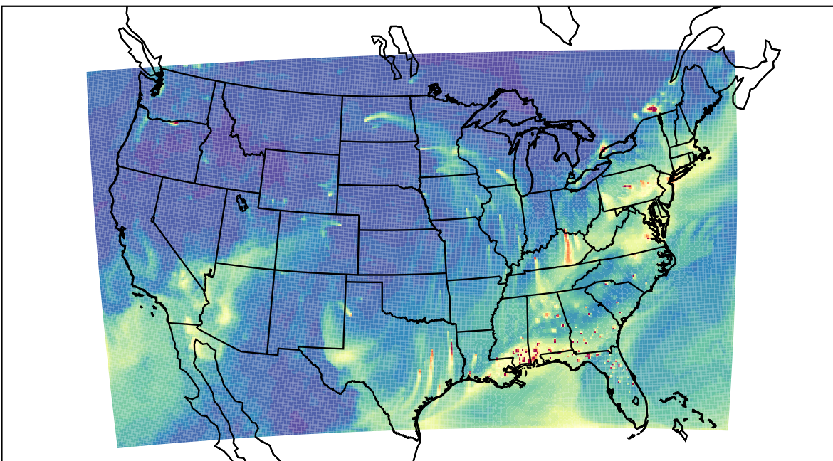
WRF 2023-01-30_18:00:00
