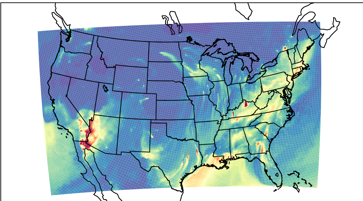
WRF 2023-01-30_08:00:00
