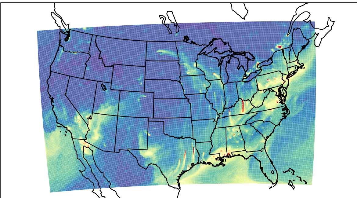
WRF 2023-01-30_16:00:00
