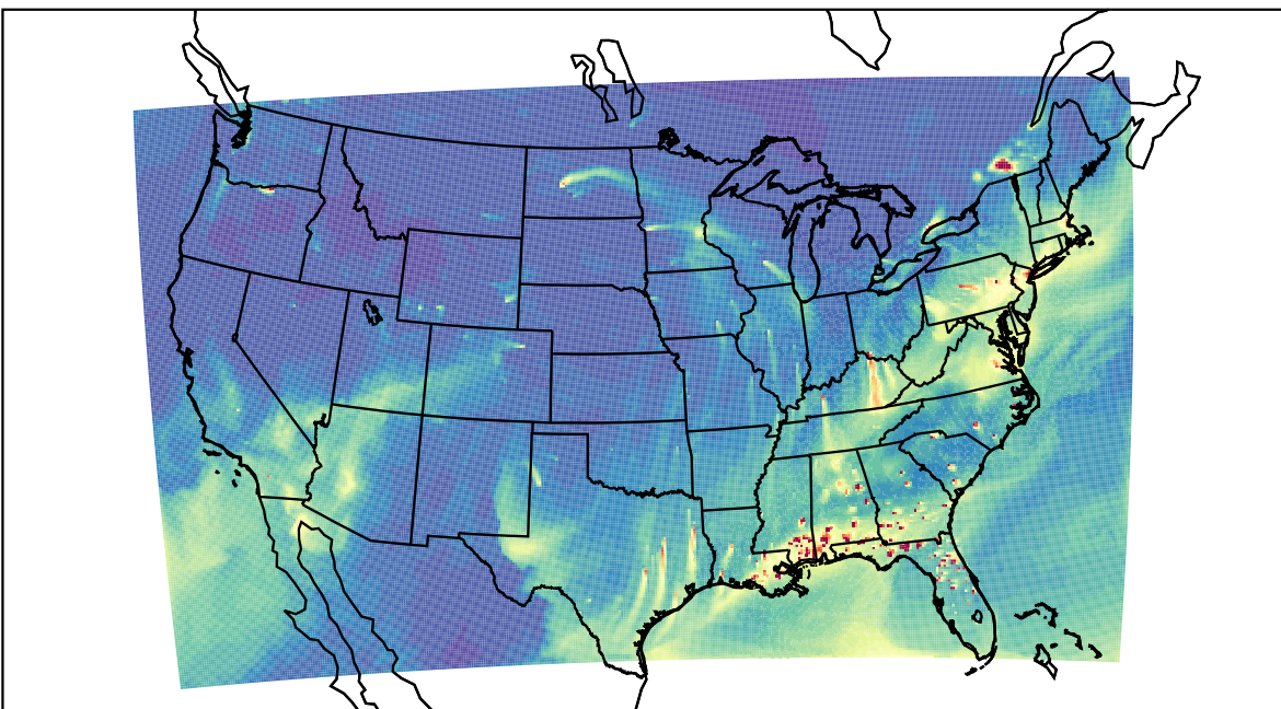
WRF 2023-01-30_20:00:00
