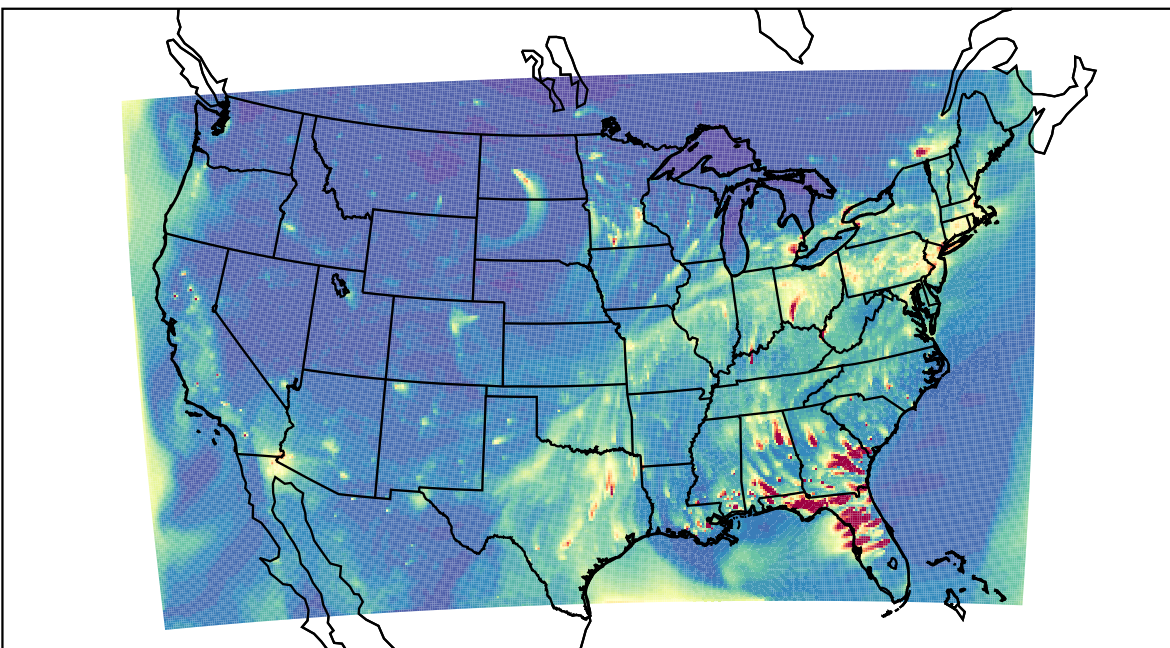
WRF 2023-01-29_01:00:00
