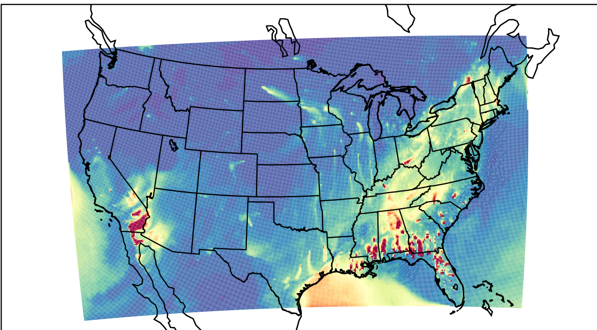
WRF 2023-01-29_23:00:00
