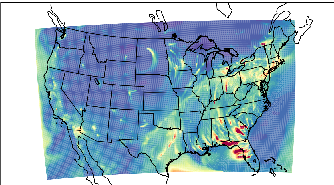
WRF 2023-01-29_04:00:00
