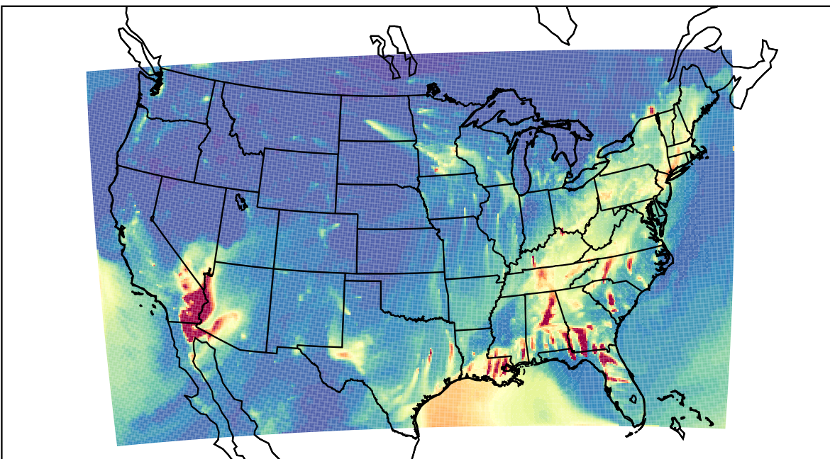
WRF 2023-01-30_03:00:00
