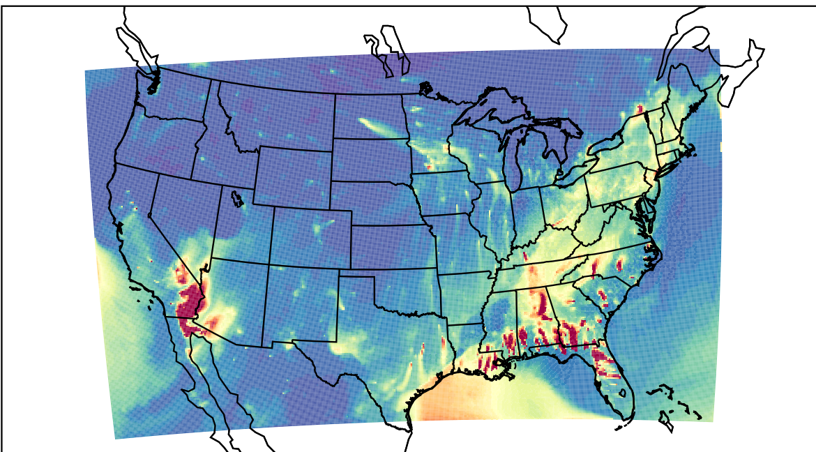
WRF 2023-01-30_01:00:00
