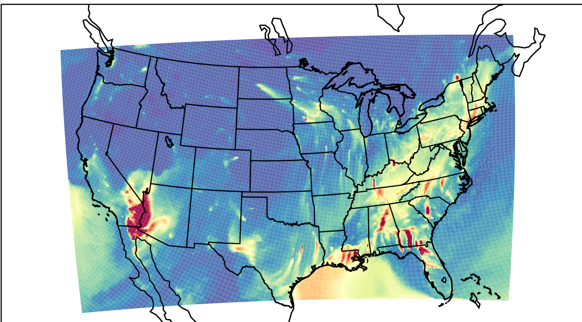
WRF 2023-01-30_04:00:00
