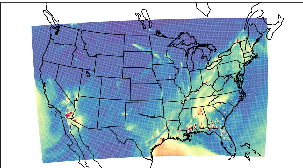
WRF 2023-01-29_20:00:00
