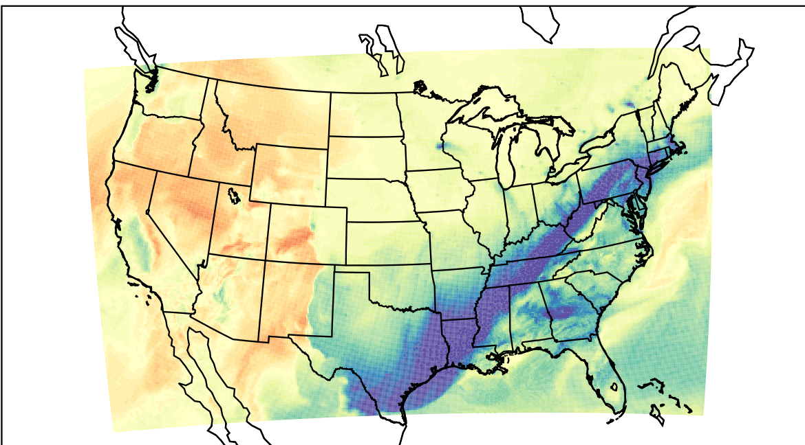
WRF (2023-01-30_22:00:00)
