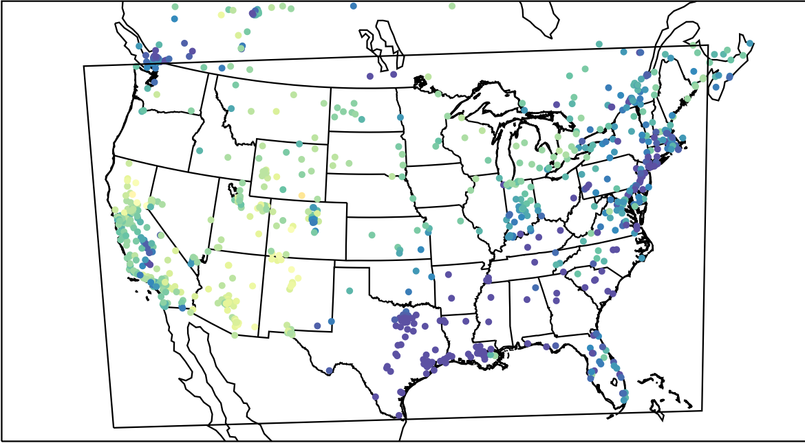
AirNOW (2023-01-30_23:00:00)
