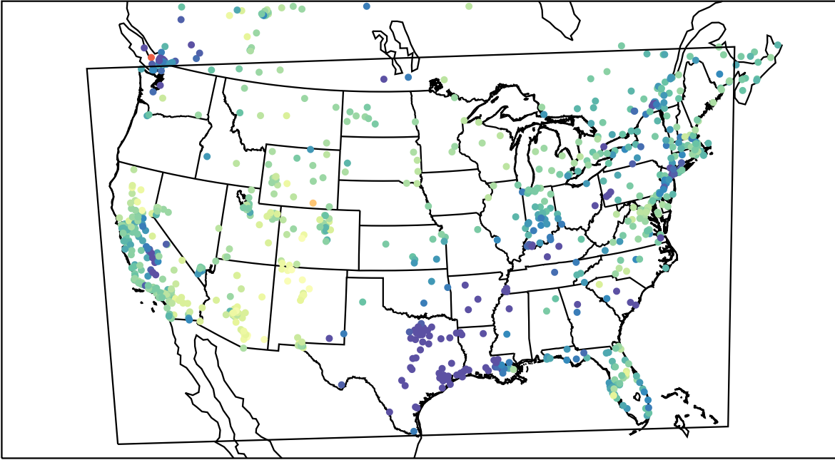
AirNOW (2023-01-30_20:00:00)
