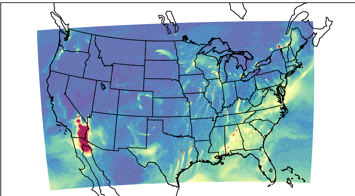
WRF 2023-01-31_14:00:00
