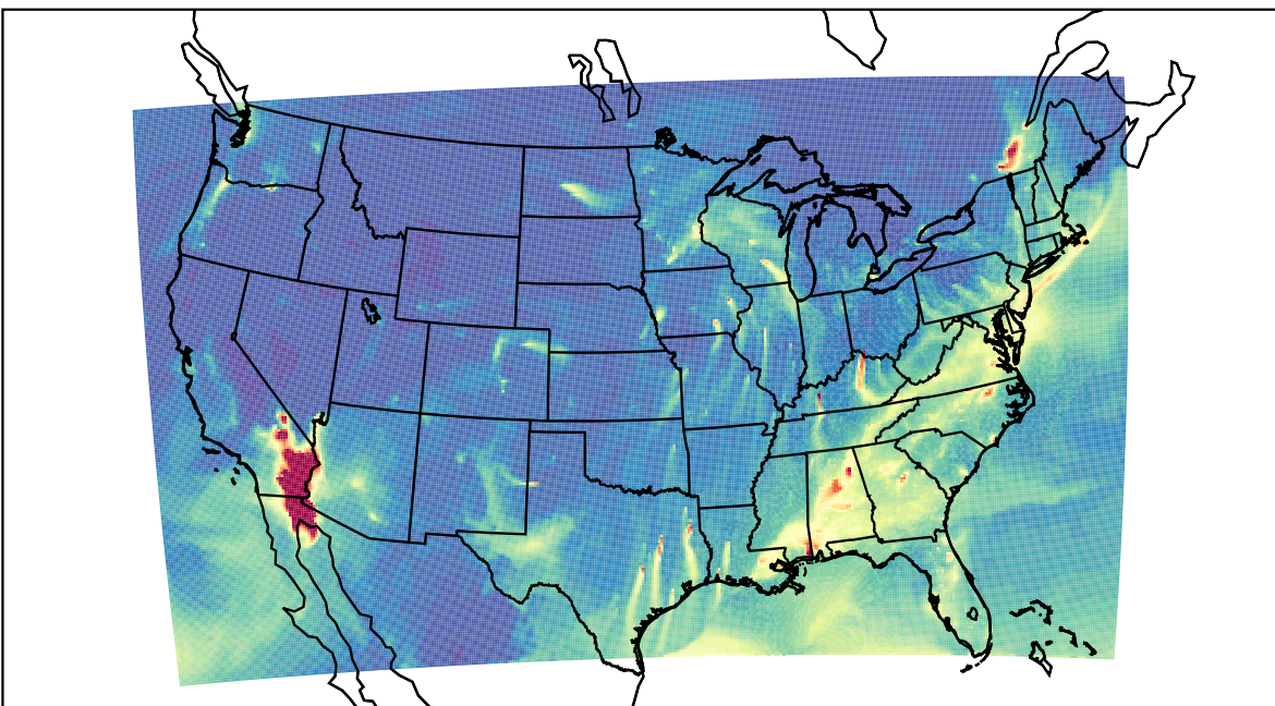
WRF 2023-01-31_10:00:00
