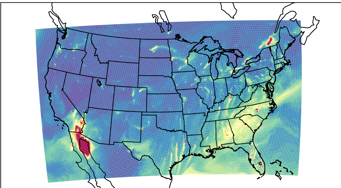
WRF 2023-01-31_23:00:00
