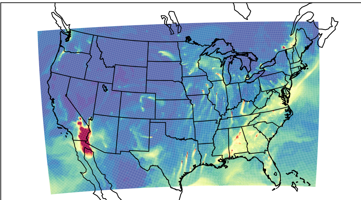
WRF 2023-01-31_13:00:00
