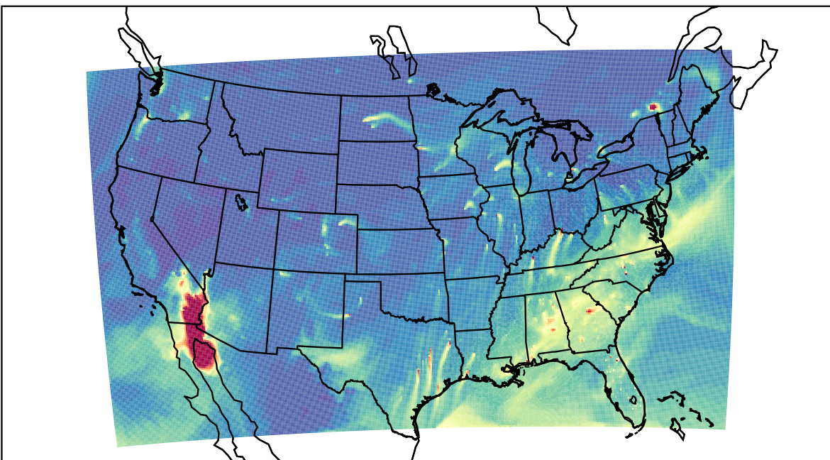
WRF 2023-01-31_18:00:00
