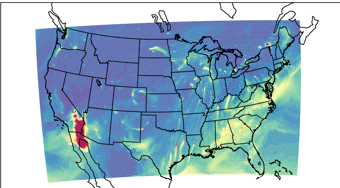
WRF 2023-01-31_16:00:00
