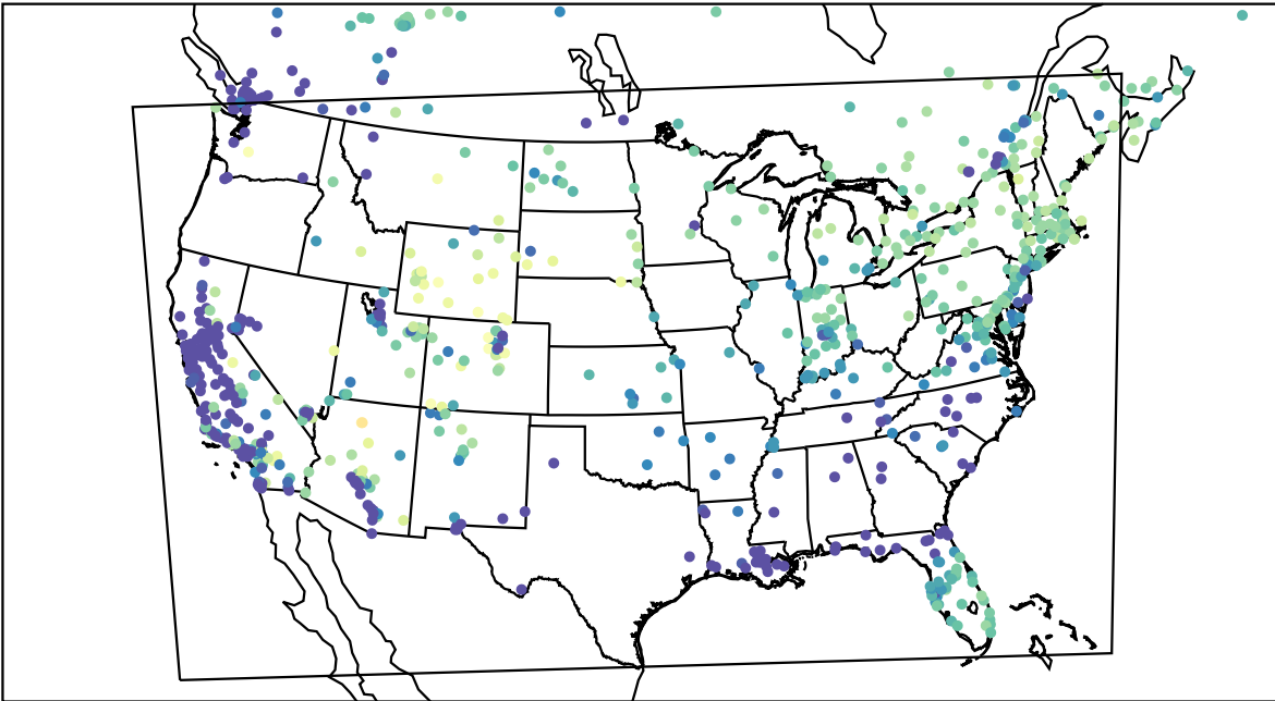
AirNOW (2023-02-01_16:00:00)
