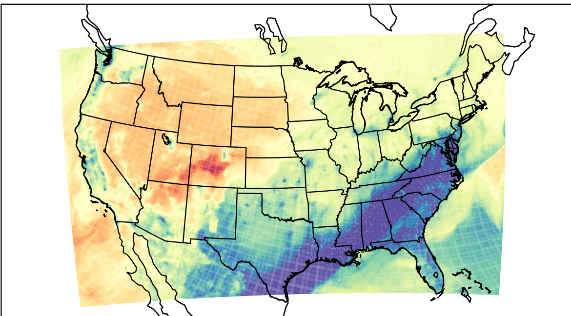
WRF (2023-02-01_04:00:00)
