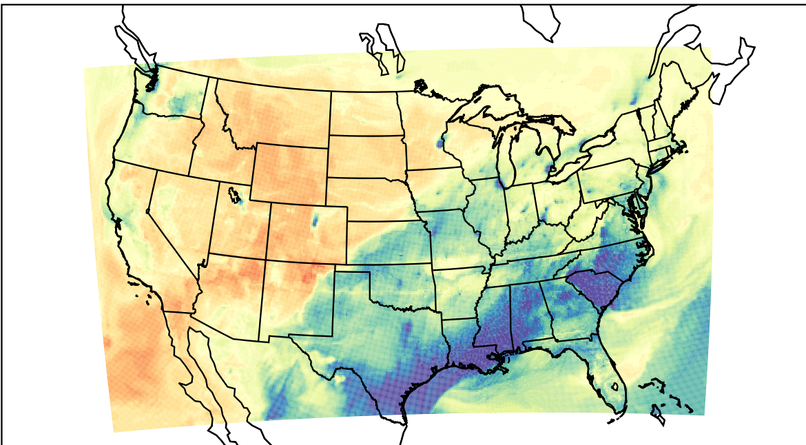
WRF (2023-02-01_23:00:00)
