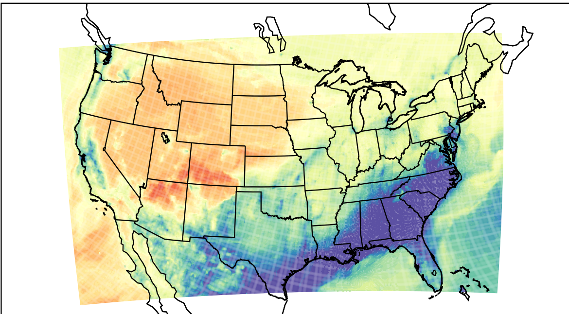
WRF (2023-02-01_12:00:00)
