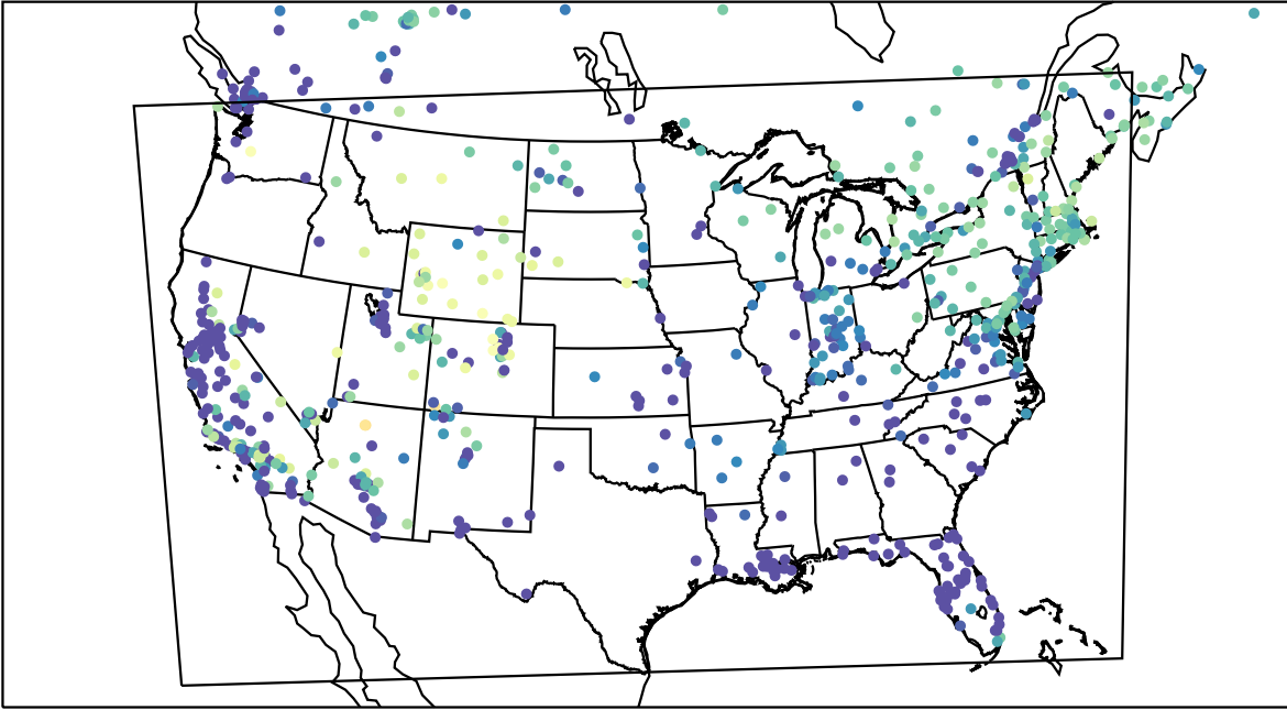
AirNOW (2023-02-01_14:00:00)
