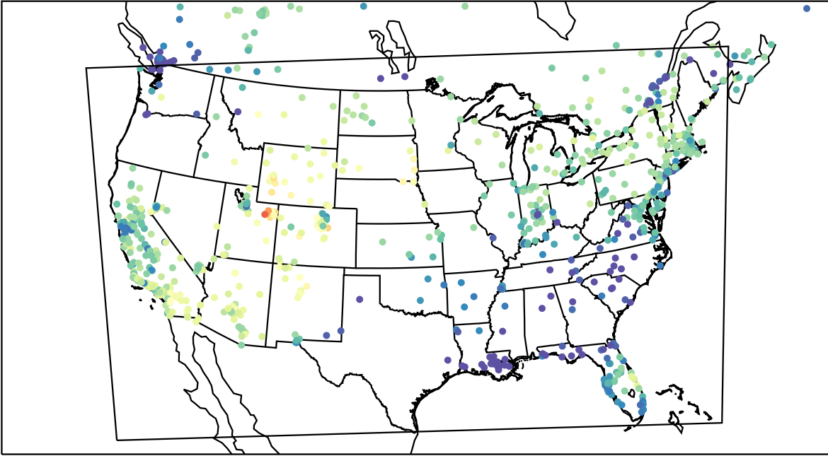
AirNOW (2023-02-01_22:00:00)
