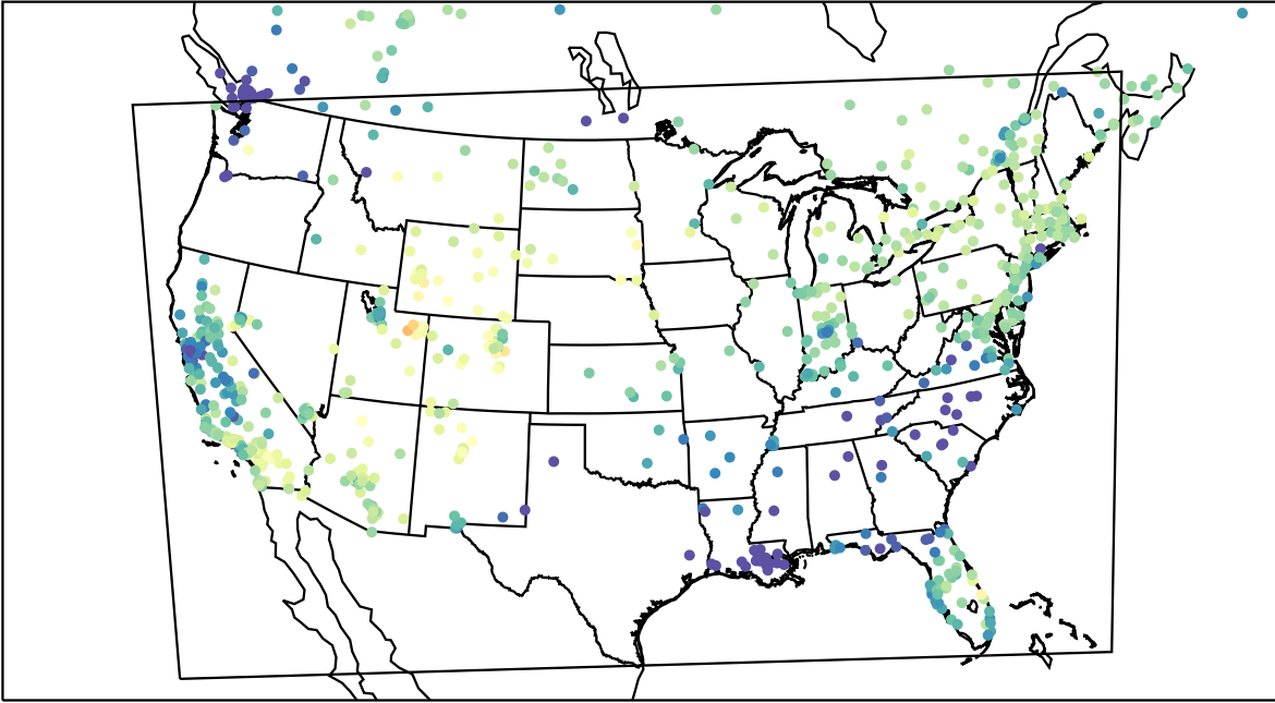
AirNOW (2023-02-01_20:00:00)
