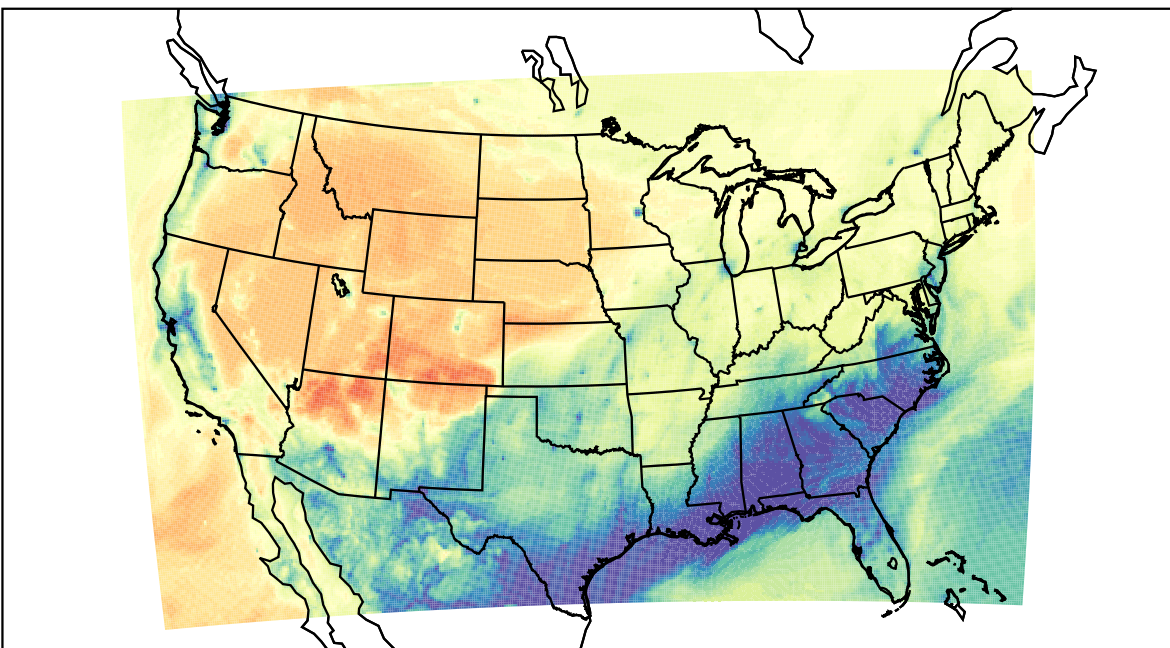
WRF (2023-02-01_15:00:00)
