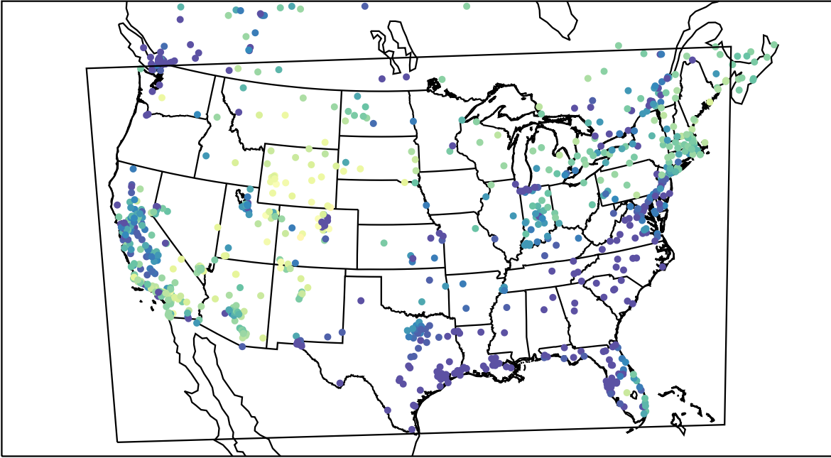
AirNOW (2023-02-01_01:00:00)
