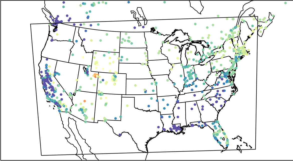
AirNOW (2023-02-02_18:00:00)
