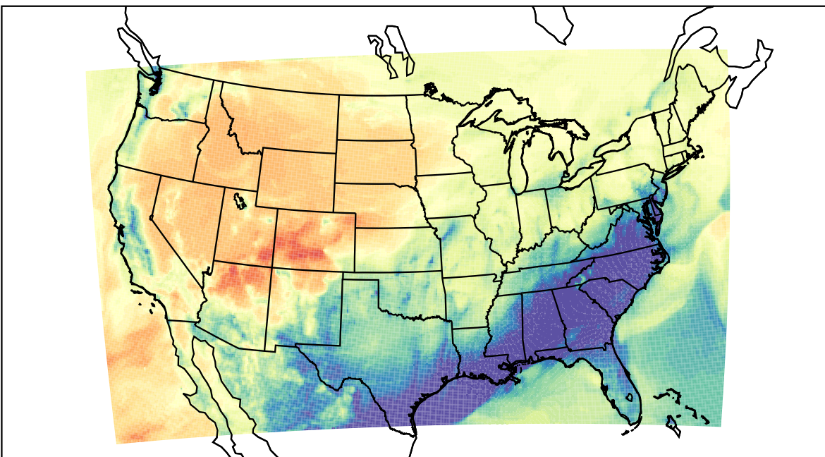
WRF (2023-02-01_08:00:00)
