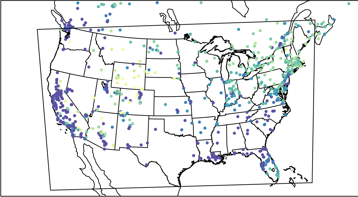
AirNOW (2023-02-01_15:00:00)
