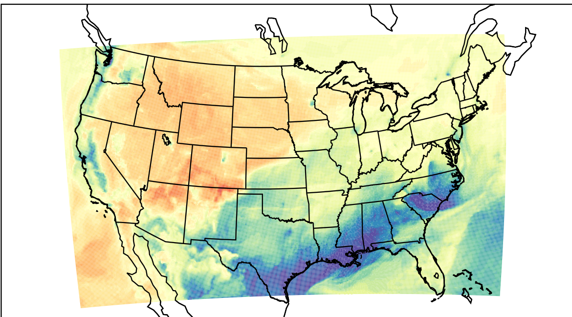
WRF (2023-02-01_18:00:00)
