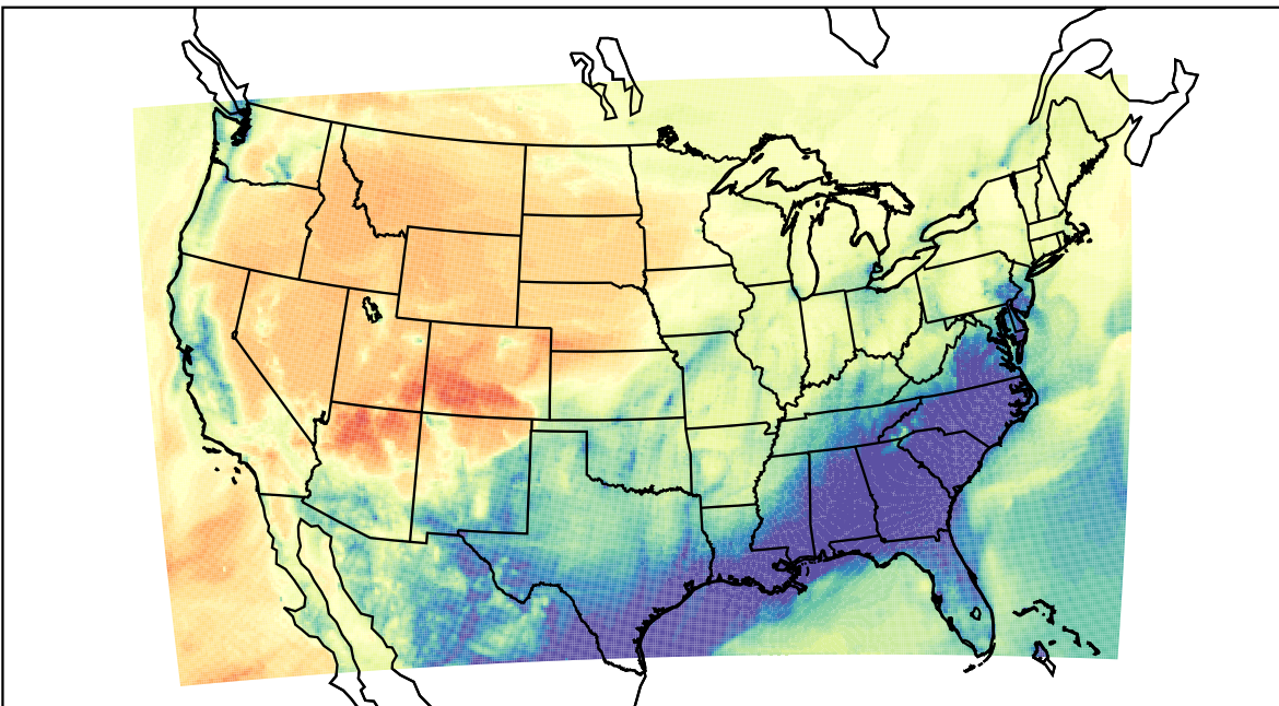
WRF (2023-02-01_11:00:00)
