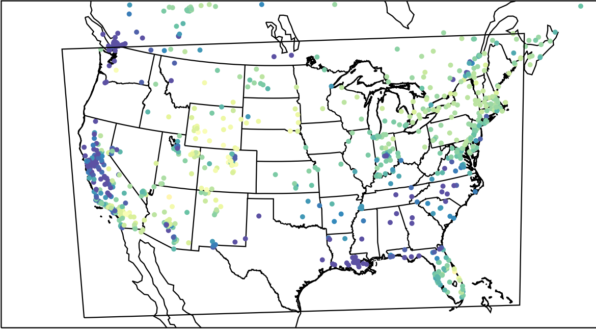
AirNOW (2023-02-01_18:00:00)
