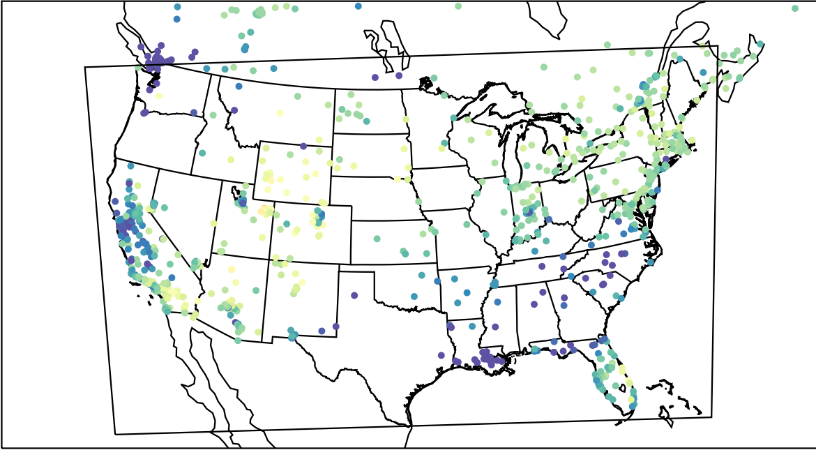
AirNOW (2023-02-01_19:00:00)
