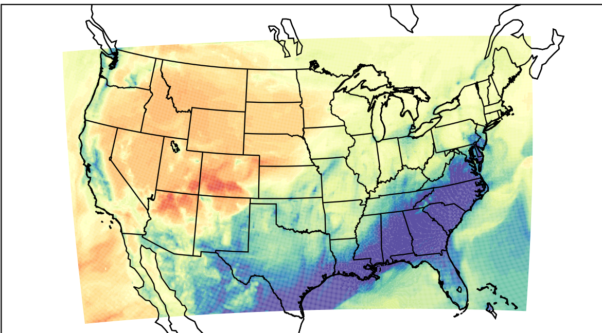
WRF (2023-02-01_10:00:00)
