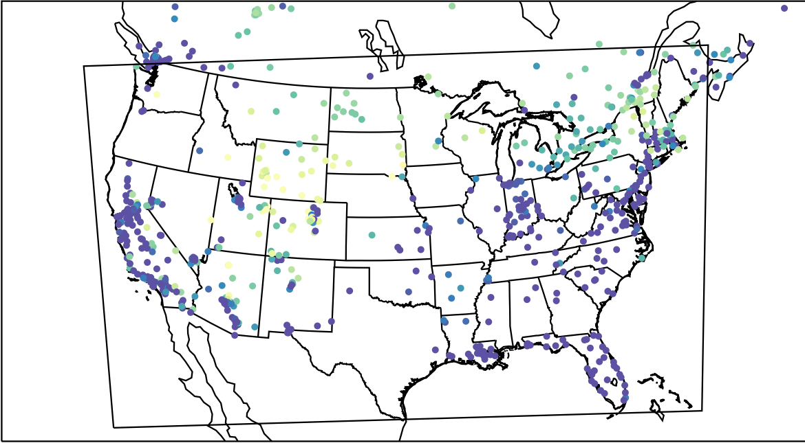
AirNOW (2023-02-02_10:00:00)
