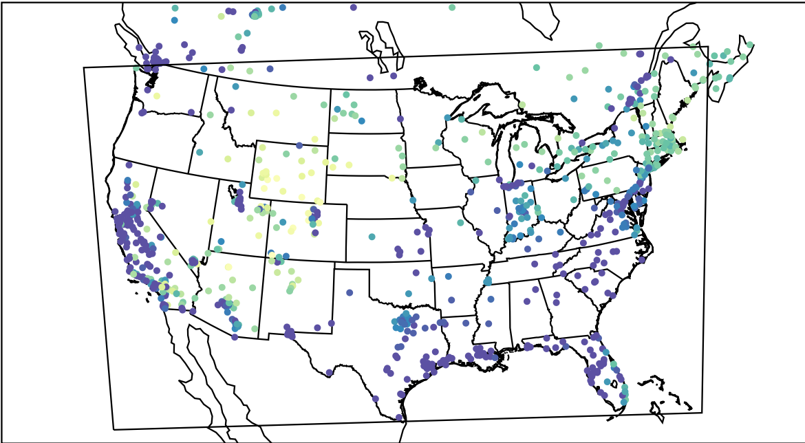
AirNOW (2023-02-01_04:00:00)
