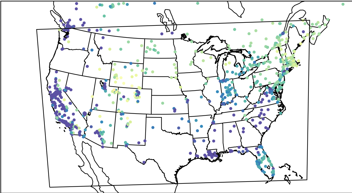
AirNOW (2023-02-02_16:00:00)
