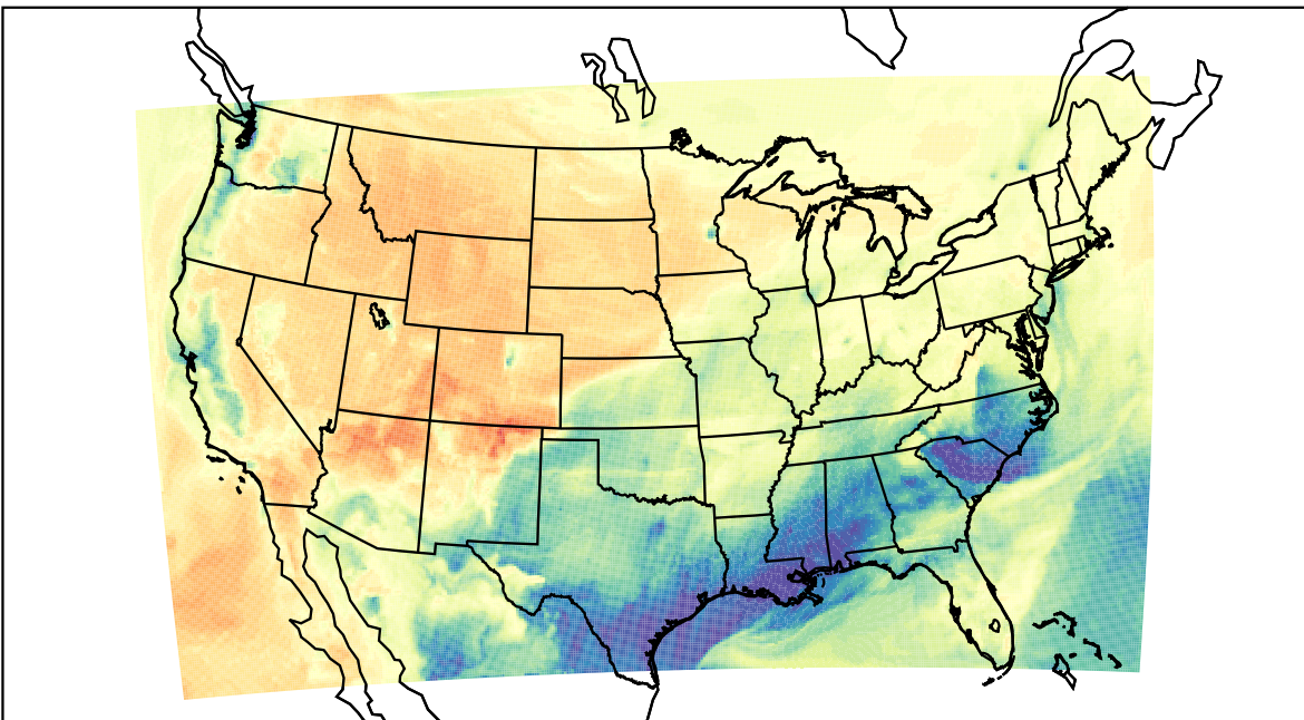
WRF (2023-02-01_19:00:00)
