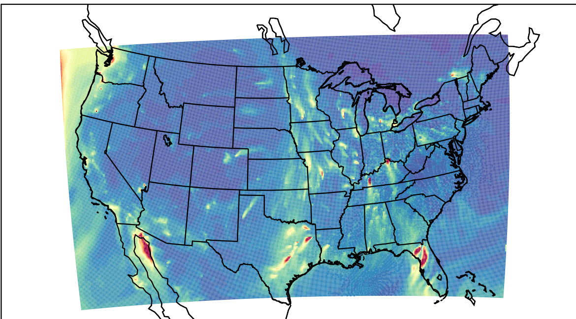
WRF 2023-02-04_04:00:00
