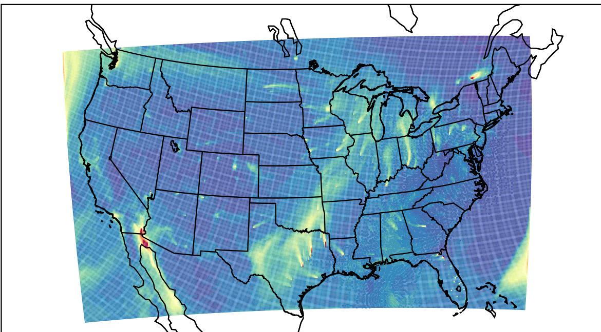
WRF 2023-02-04_18:00:00
