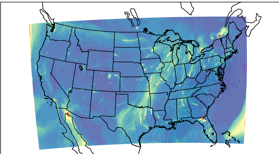
WRF 2023-02-04_22:00:00
