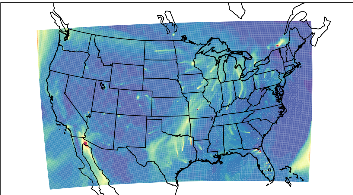
WRF 2023-02-04_20:00:00
