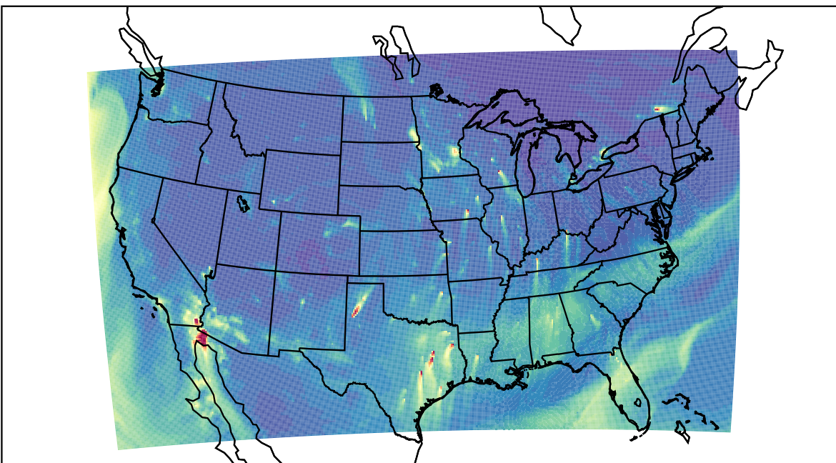
WRF 2023-02-03_16:00:00
