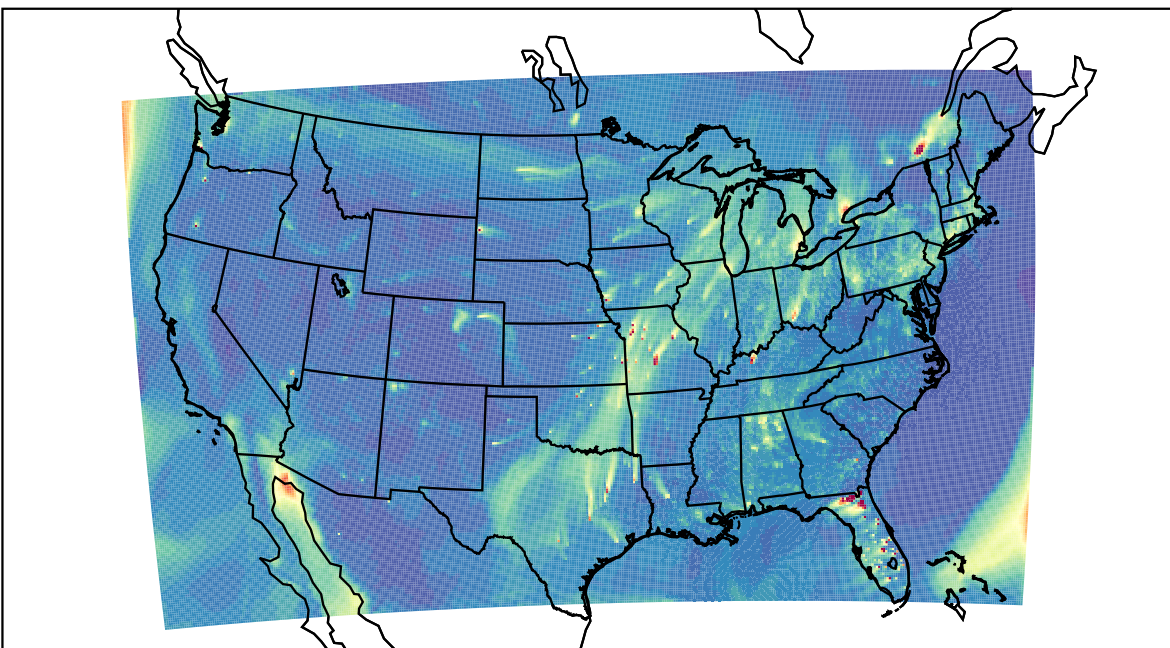
WRF 2023-02-04_23:00:00
