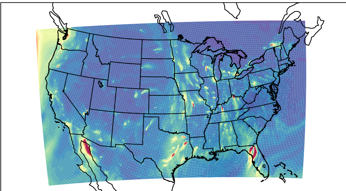
WRF 2023-02-04_03:00:00
