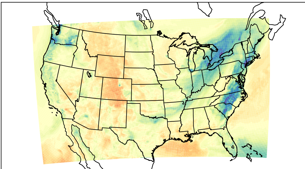
WRF (2023-02-05_20:00:00)
