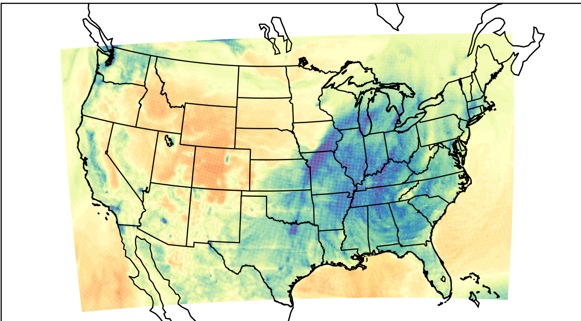
WRF (2023-02-05_03:00:00)
