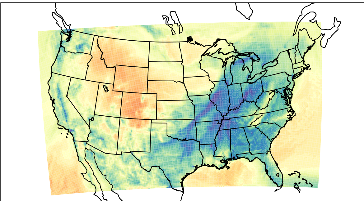
WRF (2023-02-05_10:00:00)
