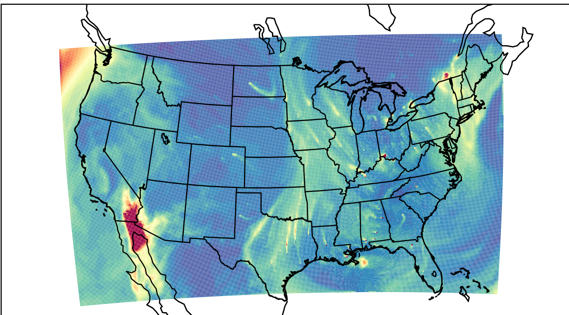
WRF 2023-02-06_20:00:00
