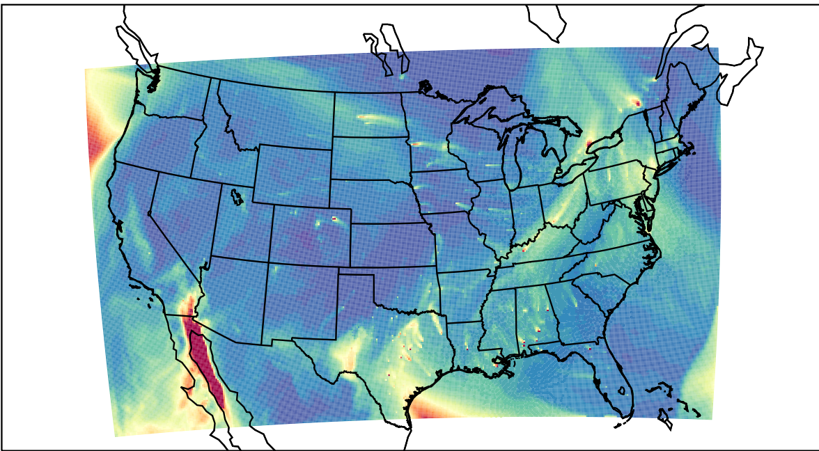
WRF 2023-02-07_20:00:00
