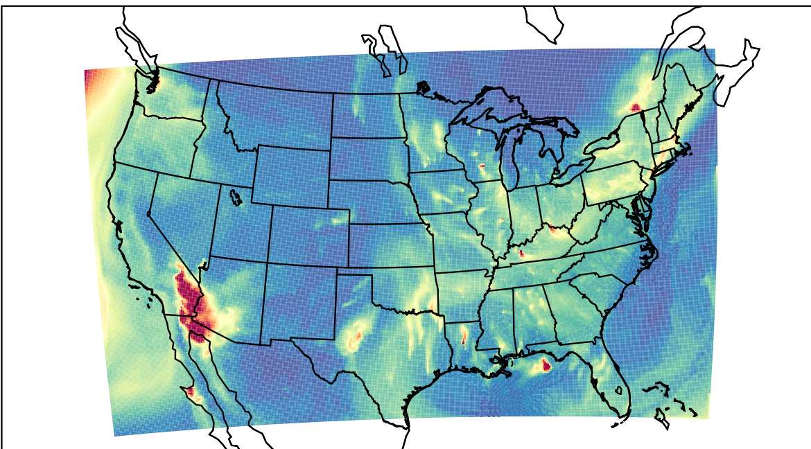
WRF 2023-02-06_10:00:00
