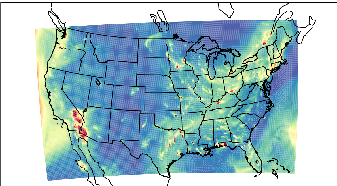
WRF 2023-02-06_03:00:00
