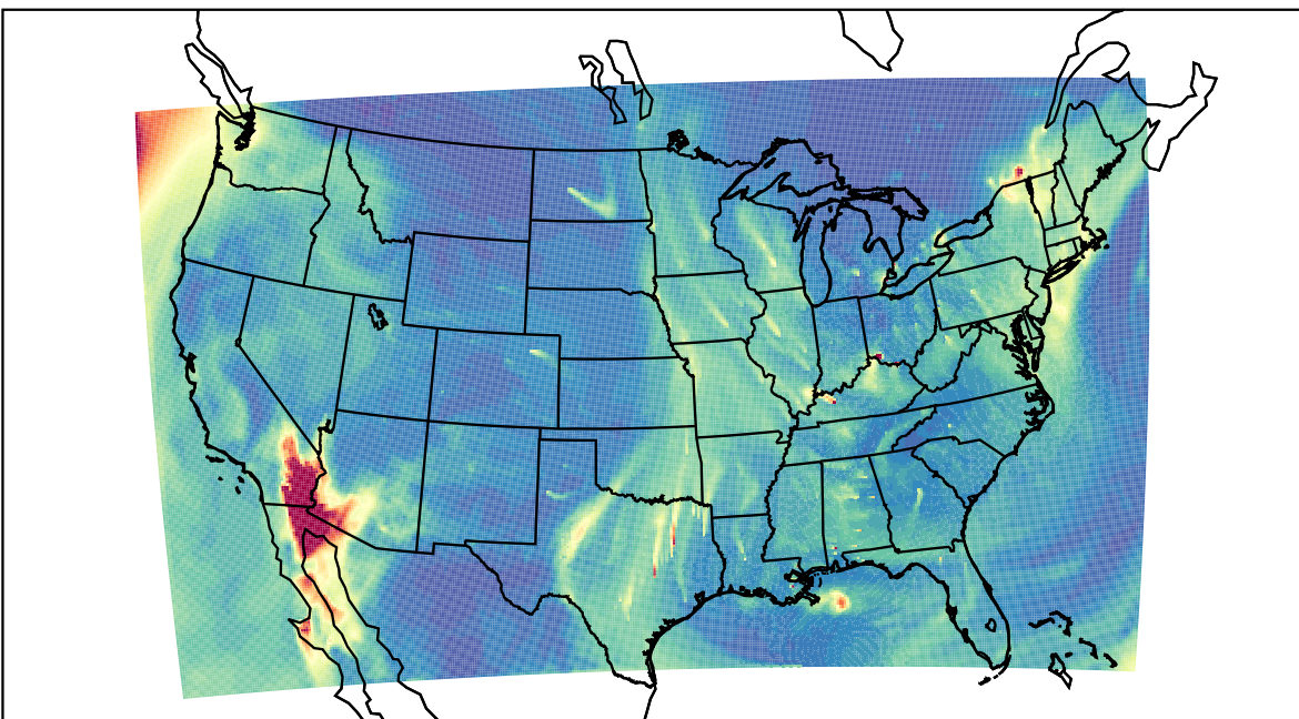
WRF 2023-02-06_18:00:00
