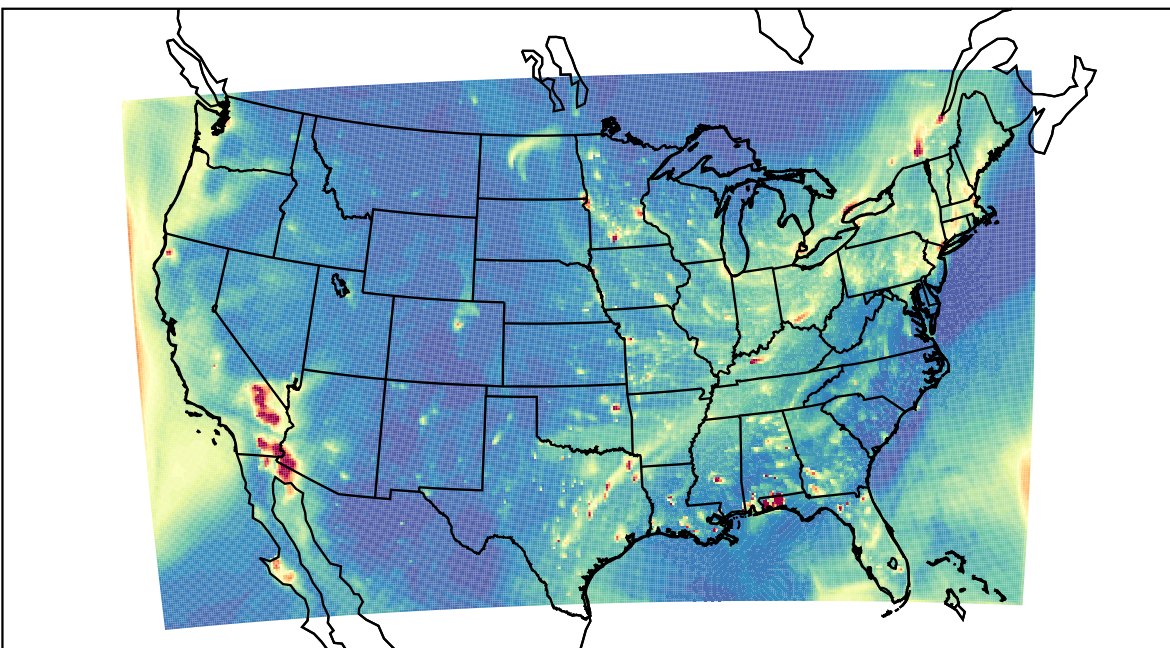
WRF 2023-02-06_01:00:00
