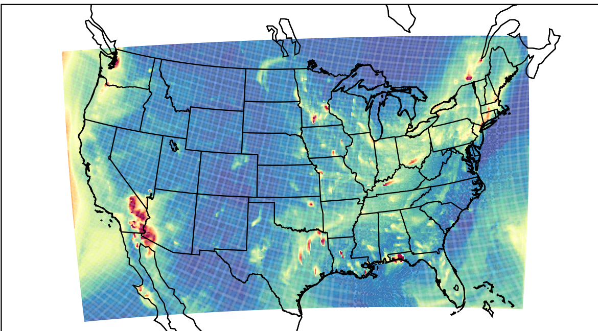
WRF 2023-02-06_04:00:00
