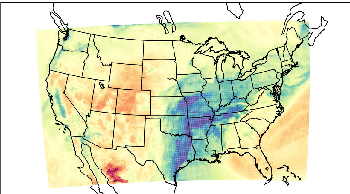
WRF (2023-02-08_18:00:00)
