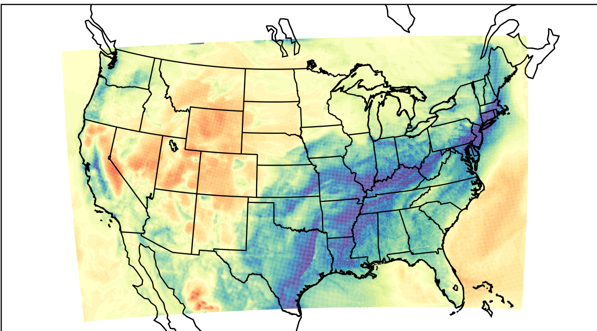
WRF (2023-02-08_10:00:00)
