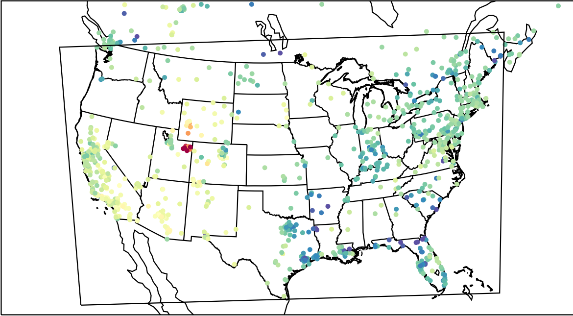
AirNOW (2023-02-10_23:00:00)
