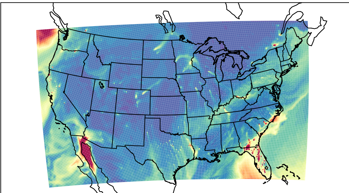
WRF 2023-02-10_22:00:00
