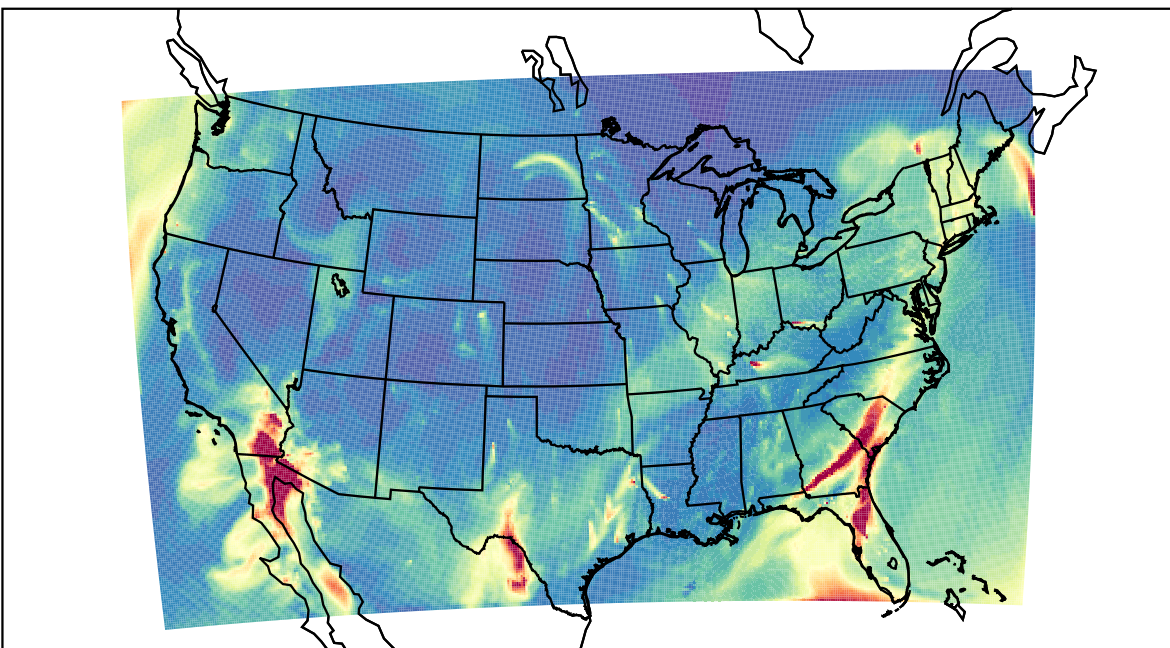
WRF 2023-02-10_10:00:00
