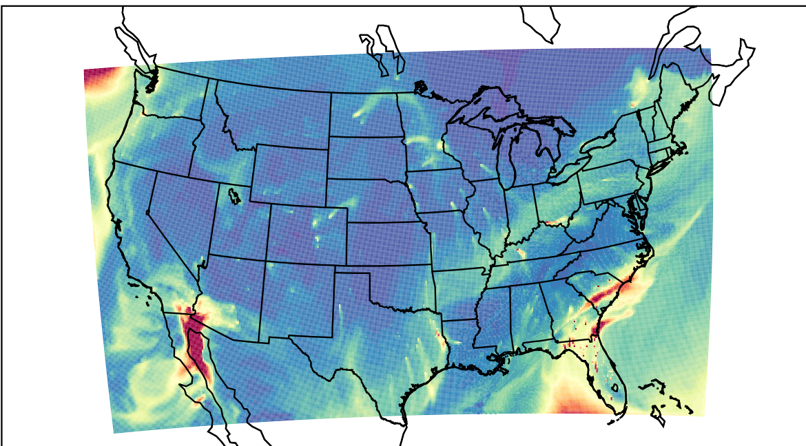
WRF 2023-02-10_18:00:00
