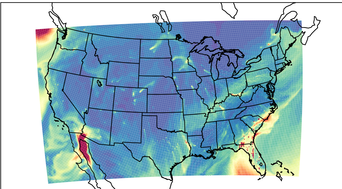
WRF 2023-02-10_20:00:00
