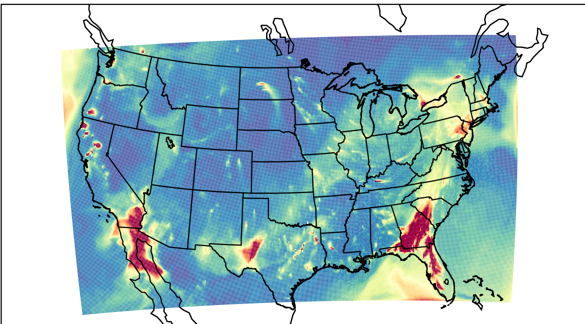
WRF 2023-02-10_03:00:00
