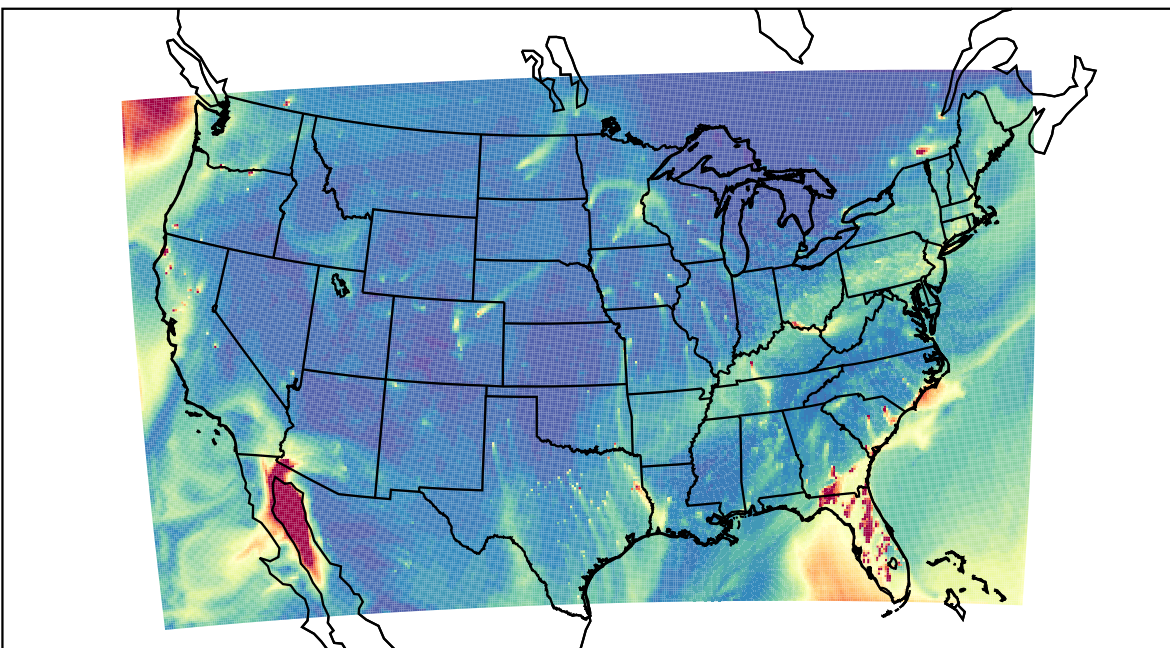
WRF 2023-02-10_23:00:00
