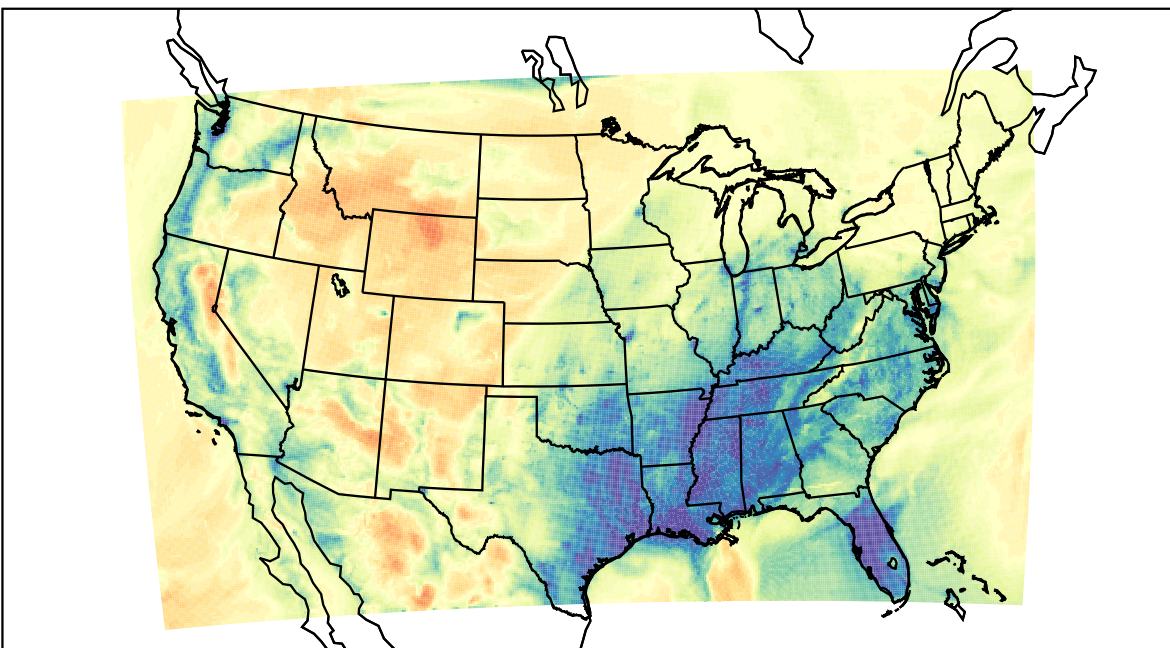
WRF (2023-02-11_13:00:00)
