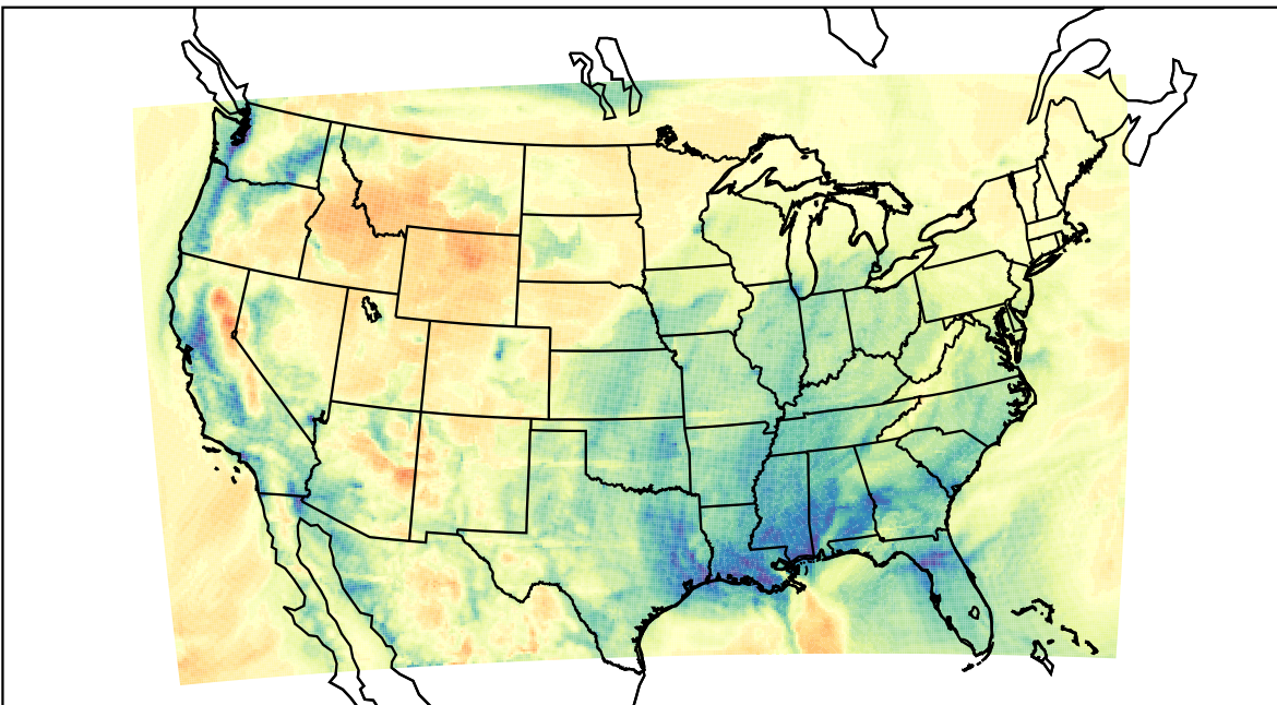
WRF (2023-02-11_16:00:00)
