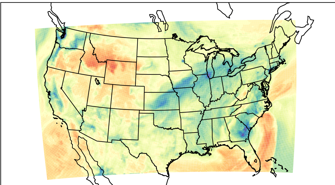
WRF (2023-02-12_18:00:00)
