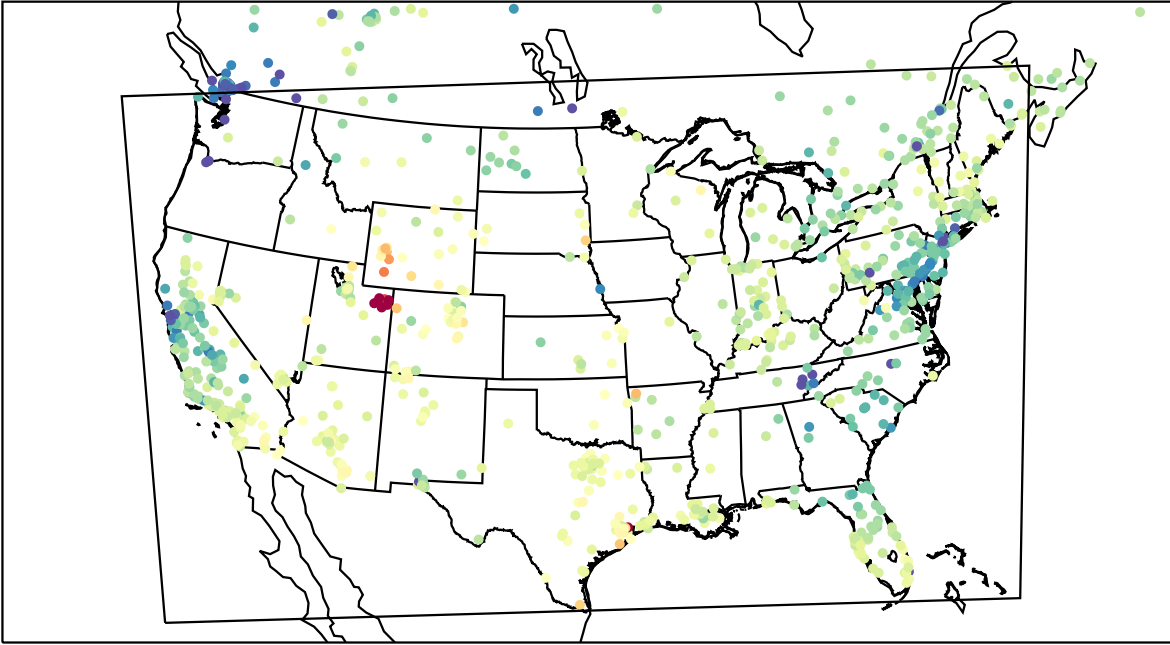
AirNOW (2023-02-12_20:00:00)
