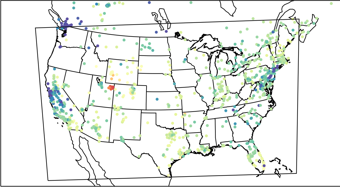
AirNOW (2023-02-12_18:00:00)
