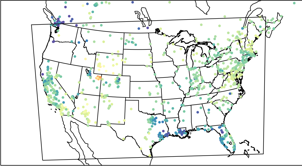
AirNOW (2023-02-11_18:00:00)
