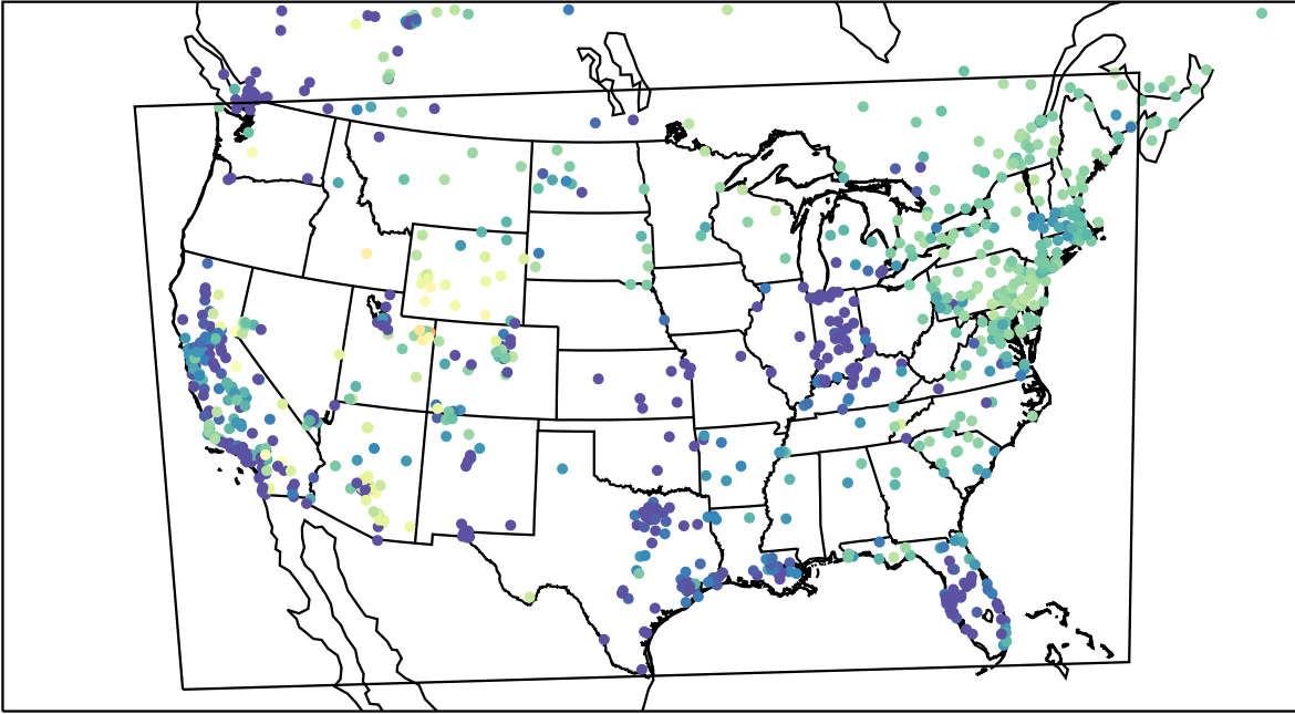
AirNOW (2023-02-11_13:00:00)
