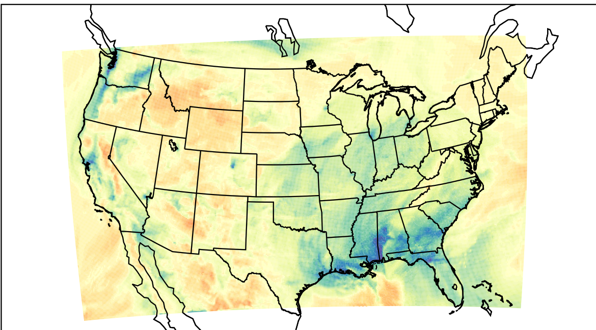
WRF (2023-02-11_18:00:00)
