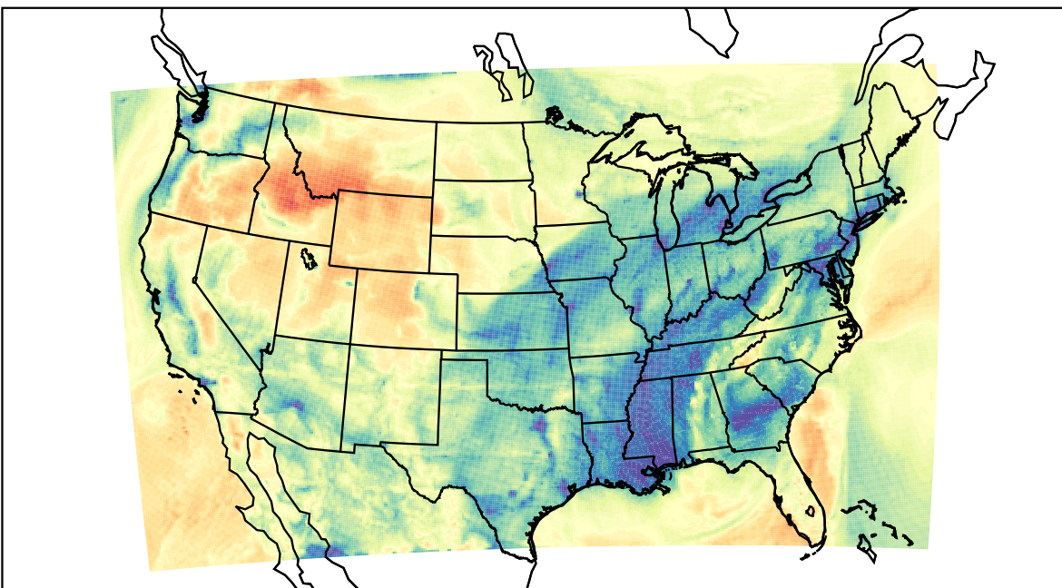
WRF (2023-02-12_13:00:00)
