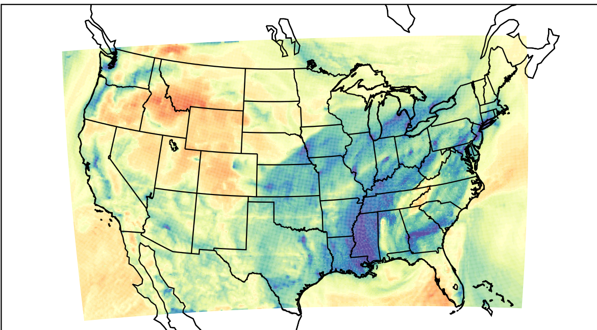
WRF (2023-02-12_10:00:00)
