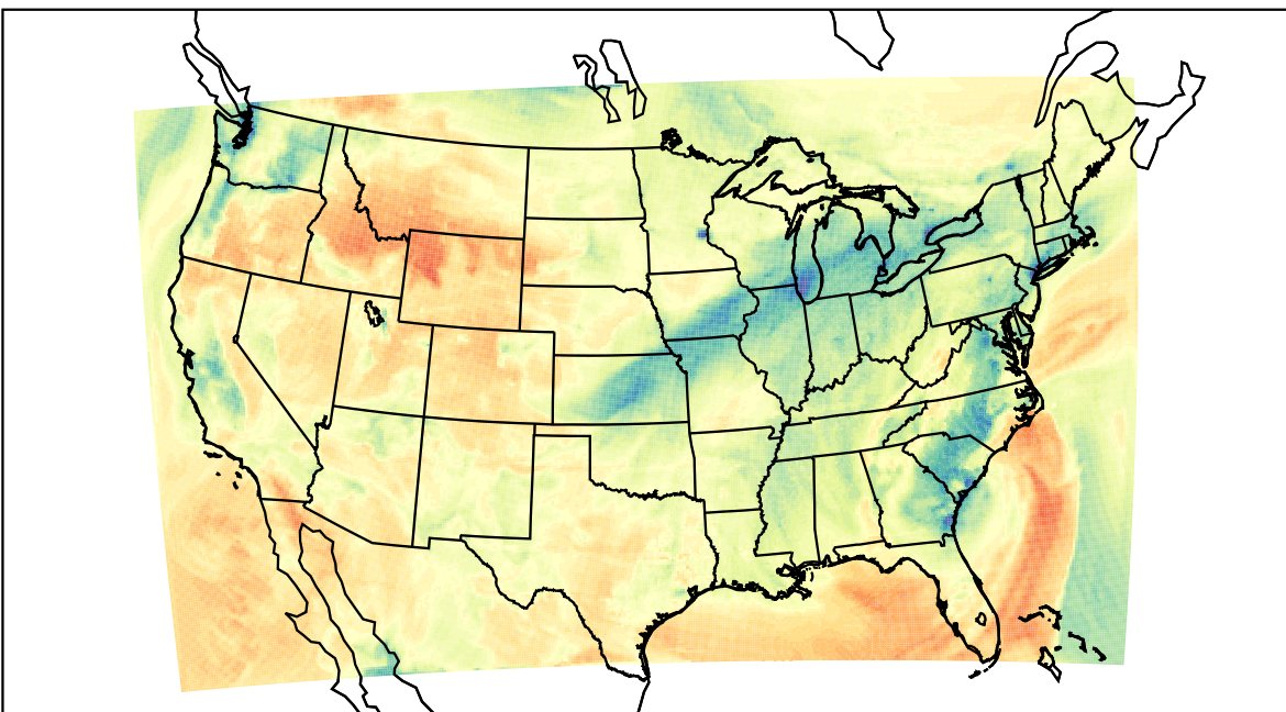
WRF (2023-02-12_20:00:00)
