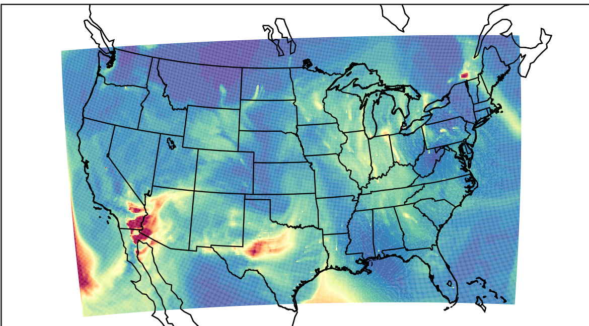
WRF 2023-02-14_20:00:00
