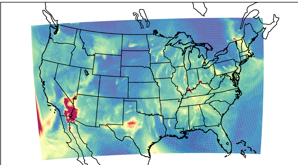
WRF 2023-02-14_10:00:00
