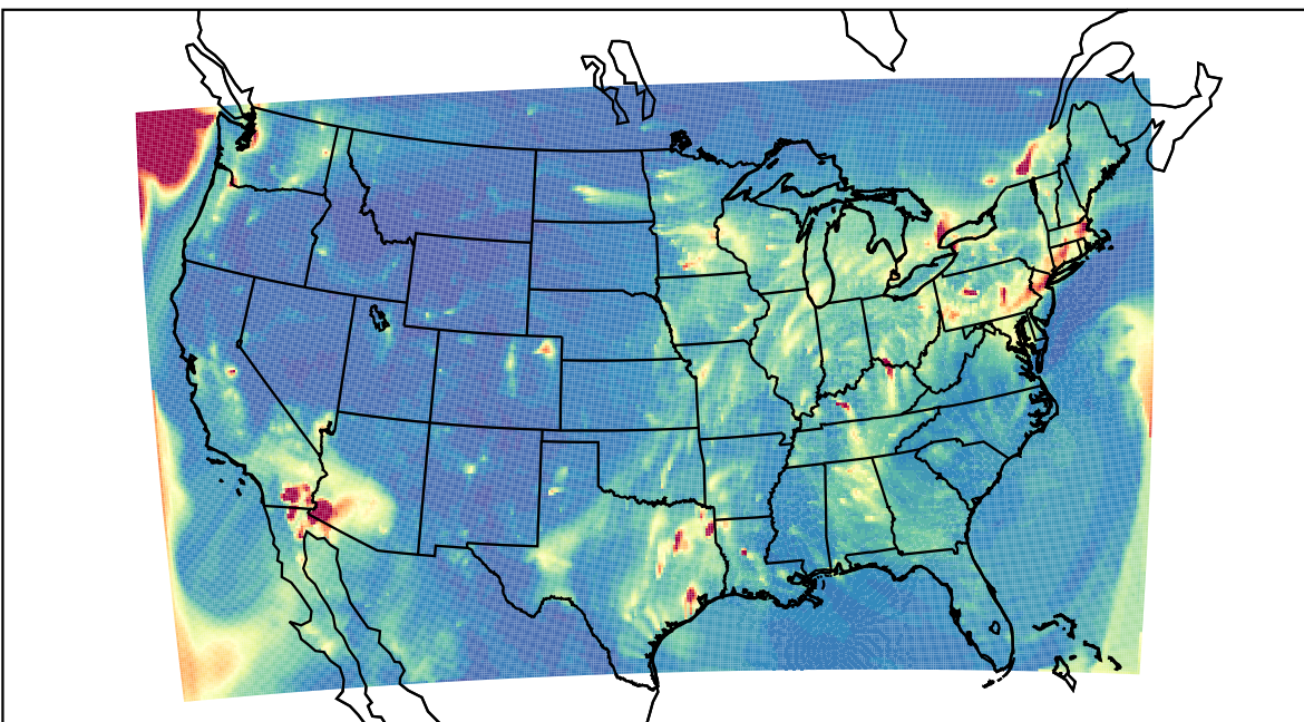
WRF 2023-02-13_03:00:00
