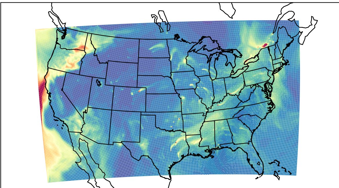
WRF 2023-02-13_20:00:00
