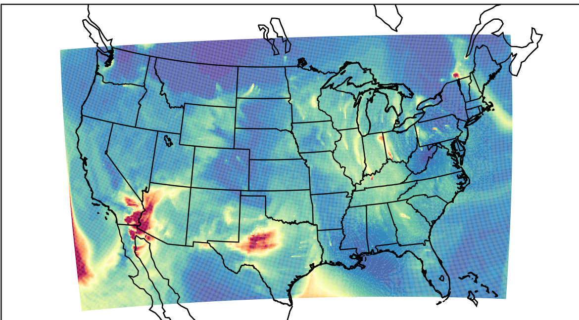
WRF 2023-02-14_18:00:00
