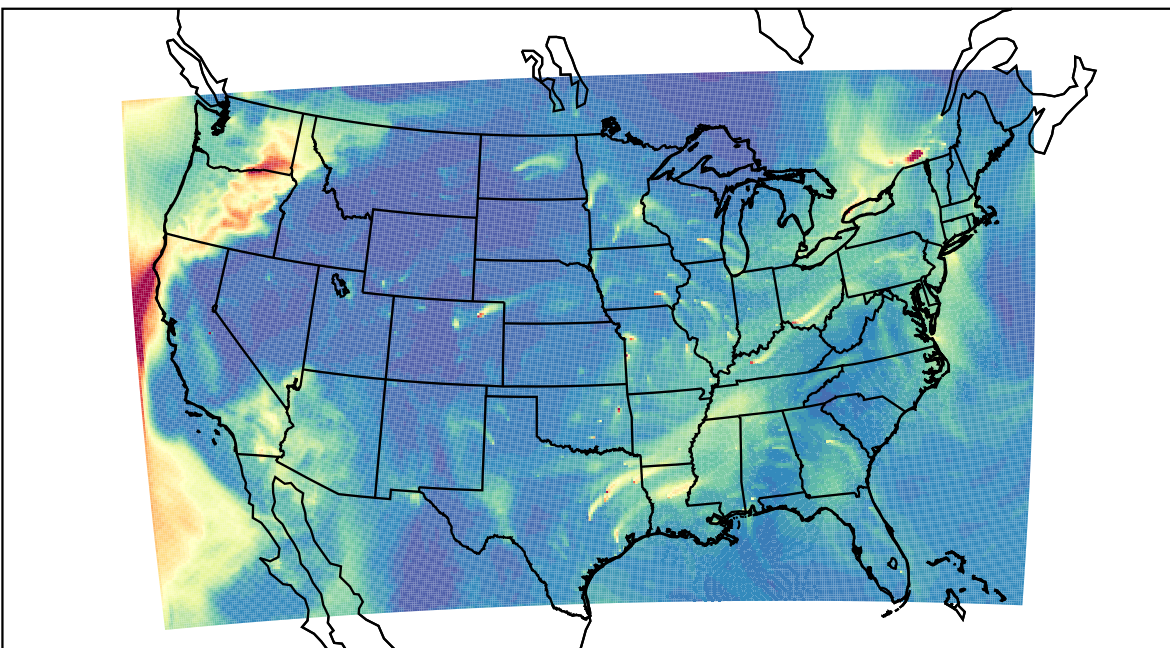
WRF 2023-02-13_19:00:00
