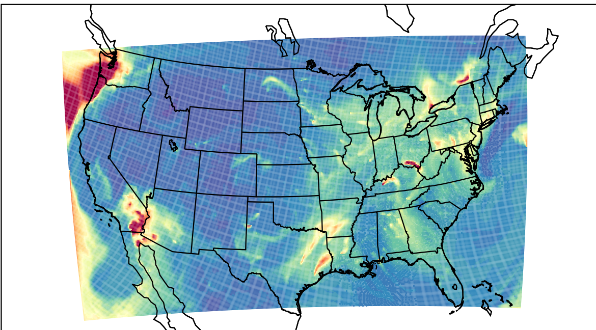
WRF 2023-02-13_10:00:00
