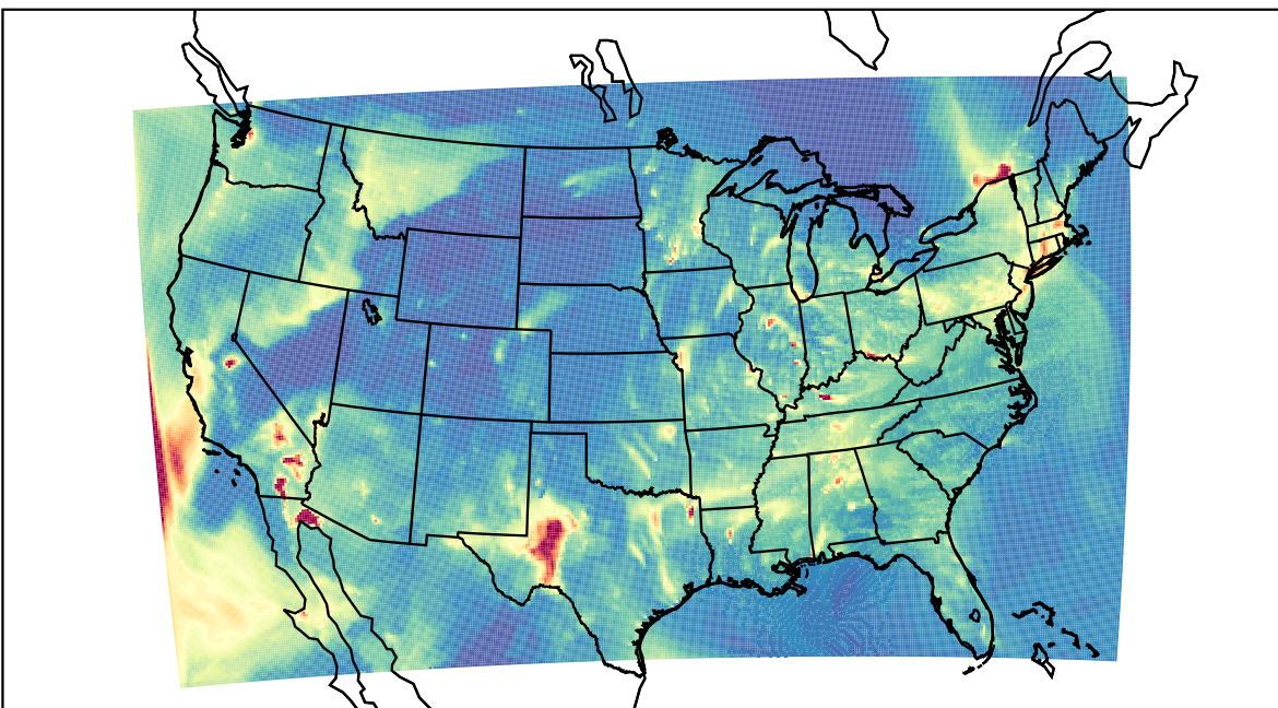
WRF 2023-02-14_03:00:00
