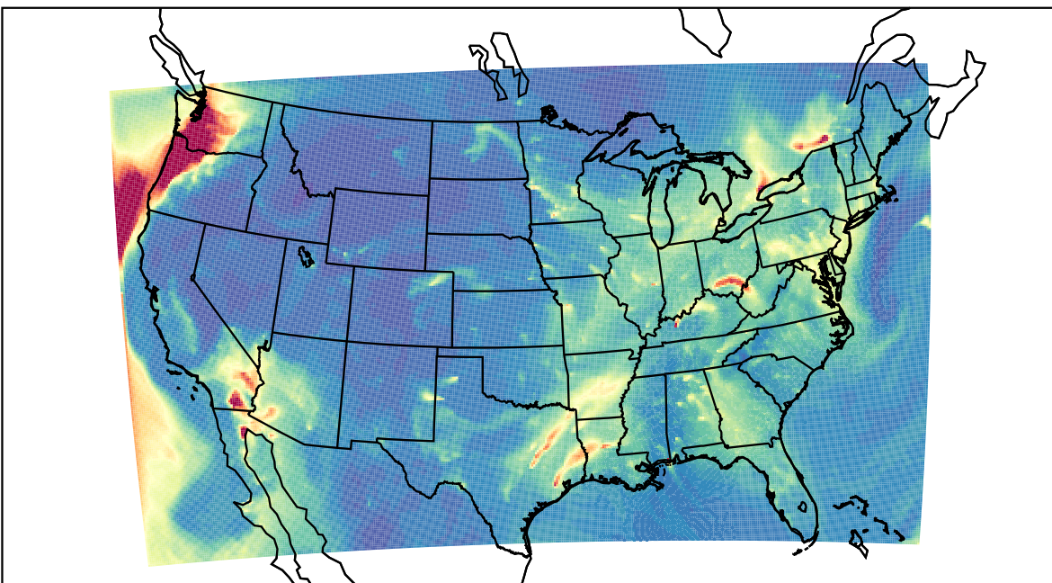
WRF 2023-02-13_13:00:00
