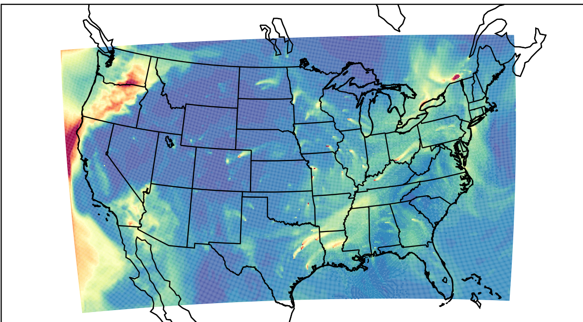
WRF 2023-02-13_18:00:00
