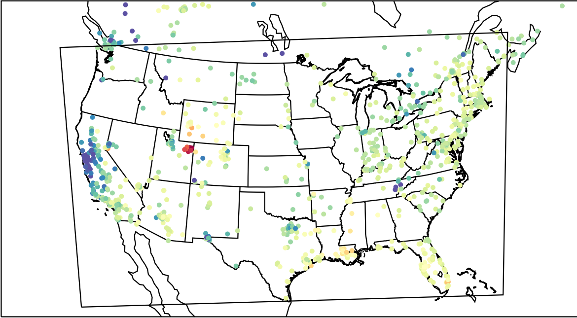
AirNOW (2023-02-13_18:00:00)
