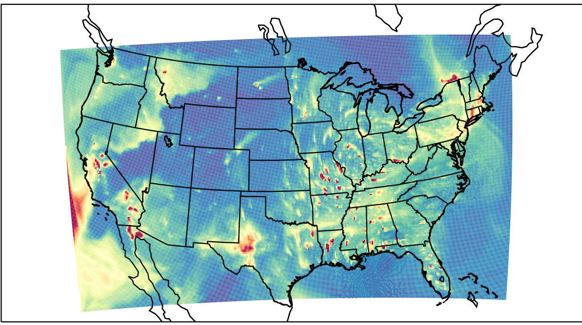
WRF 2023-02-14_03:00:00
