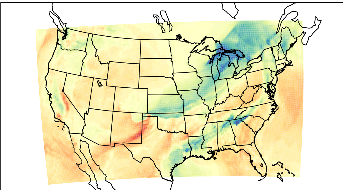
WRF (2023-02-15_20:00:00)
