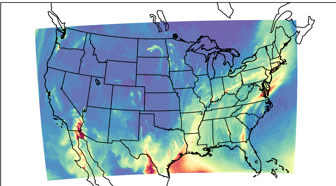
WRF 2023-02-16_10:00:00
