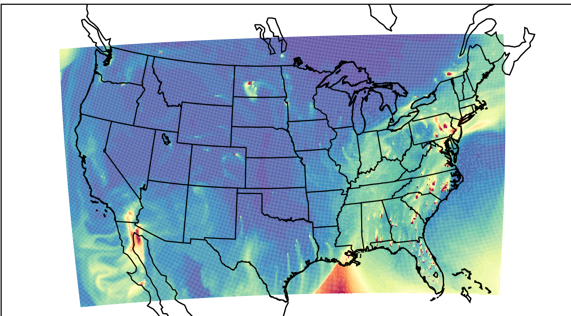
WRF 2023-02-16_20:00:00
