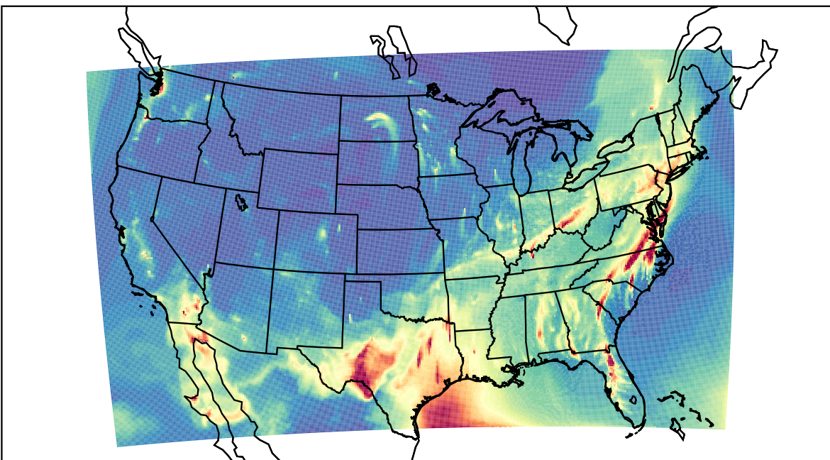
WRF 2023-02-16_04:00:00
