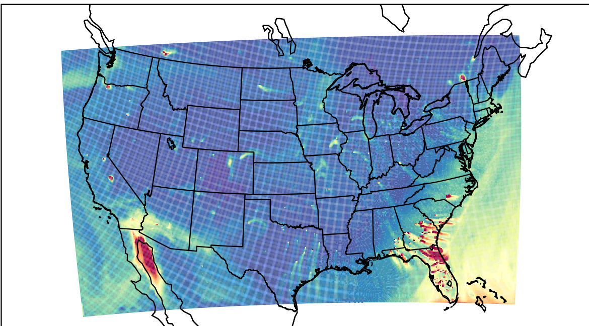
WRF 2023-02-17_23:00:00
