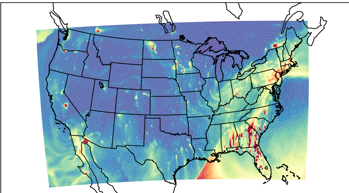
WRF 2023-02-17_01:00:00
