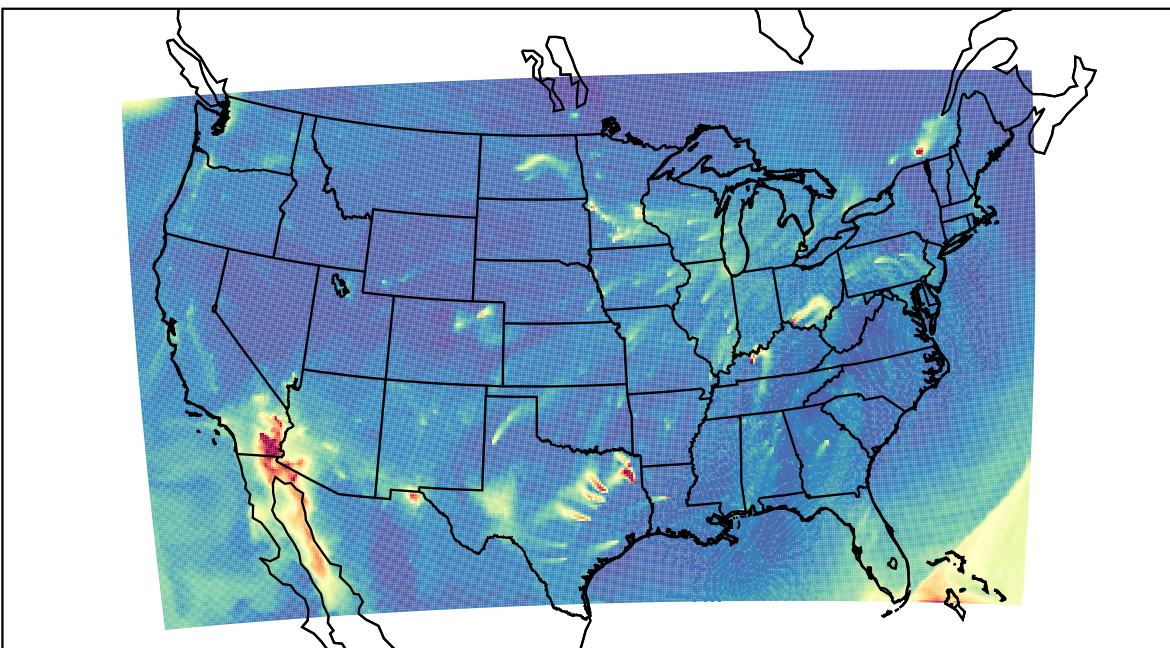
WRF 2023-02-18_15:00:00
