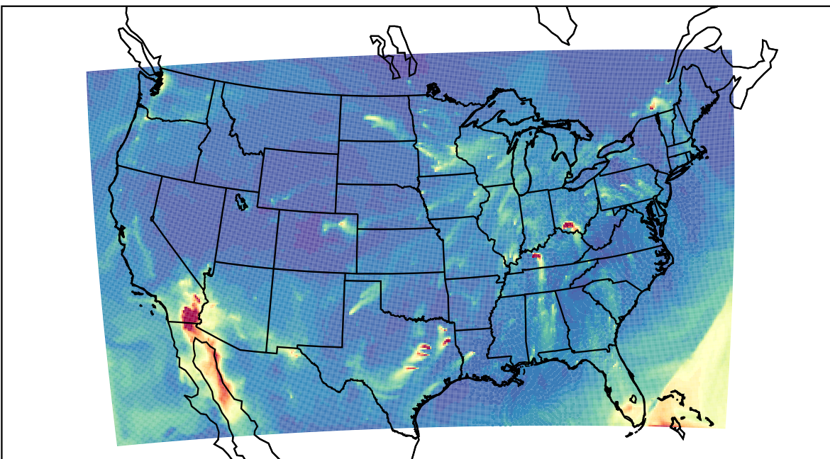
WRF 2023-02-18_11:00:00
