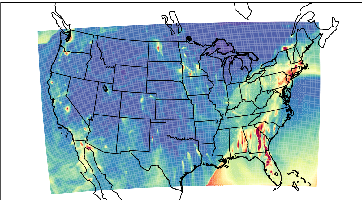
WRF 2023-02-17_03:00:00
