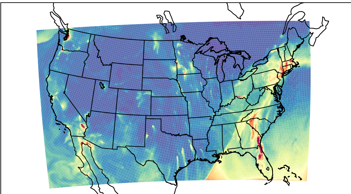
WRF 2023-02-17_06:00:00
