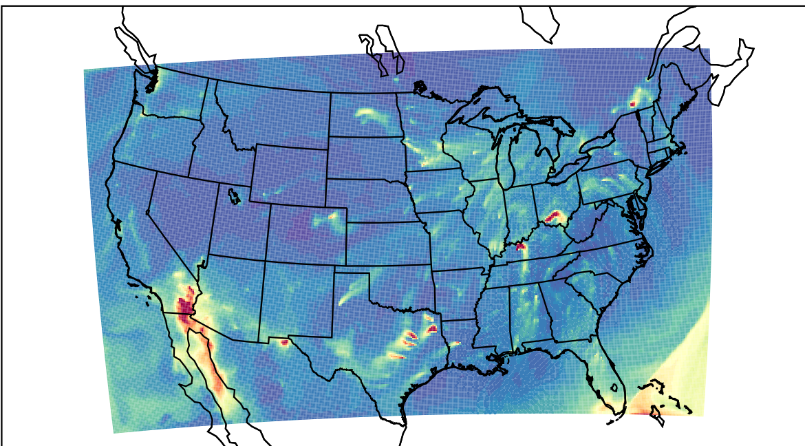
WRF 2023-02-18_13:00:00
