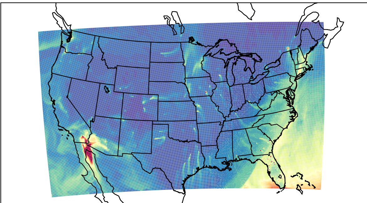
WRF 2023-02-17_18:00:00
