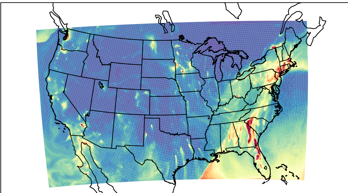
WRF 2023-02-17_04:00:00
