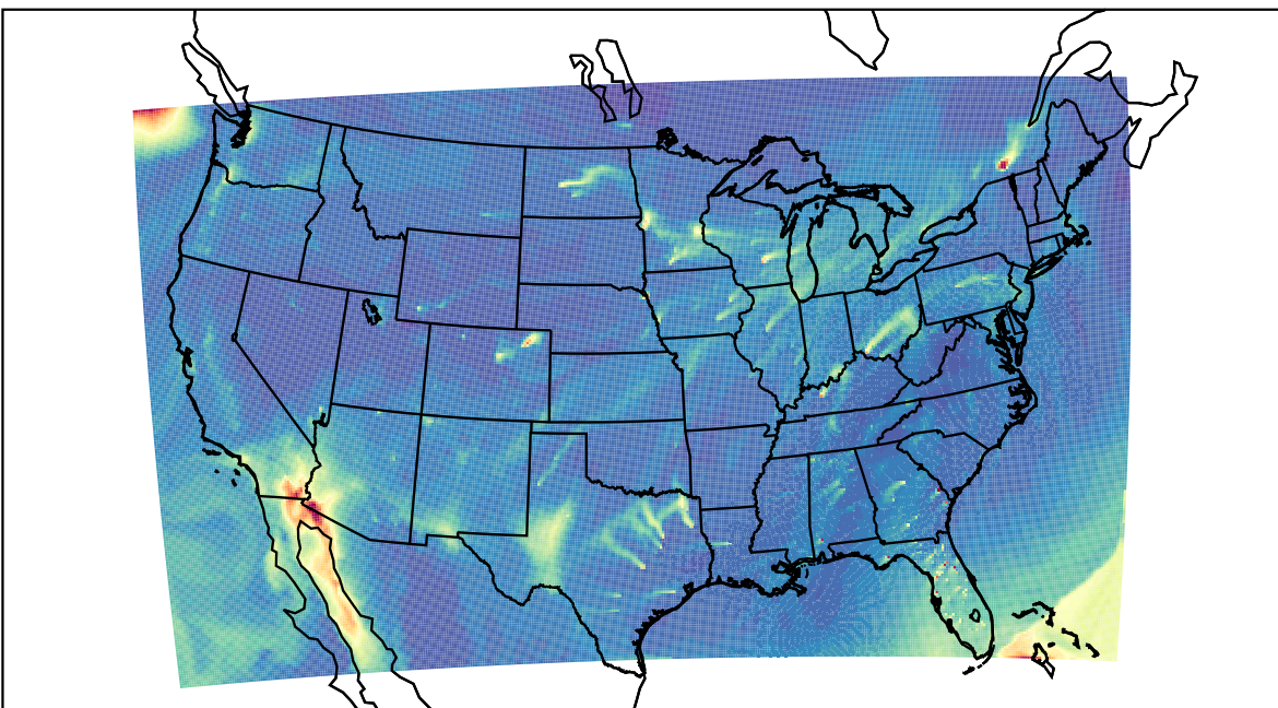
WRF 2023-02-18_18:00:00
