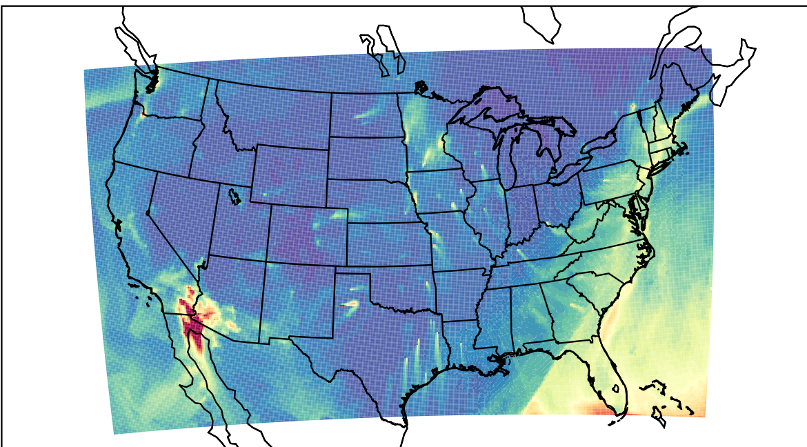
WRF 2023-02-17_16:00:00
