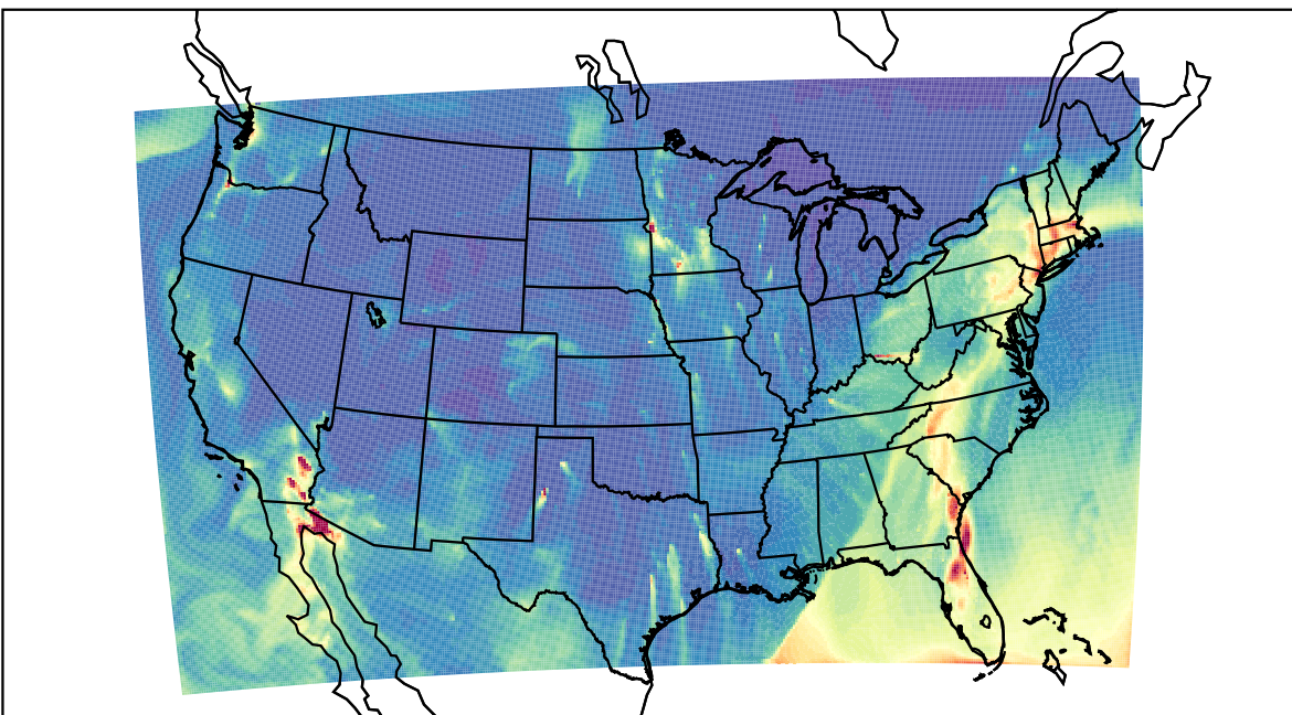
WRF 2023-02-17_08:00:00
