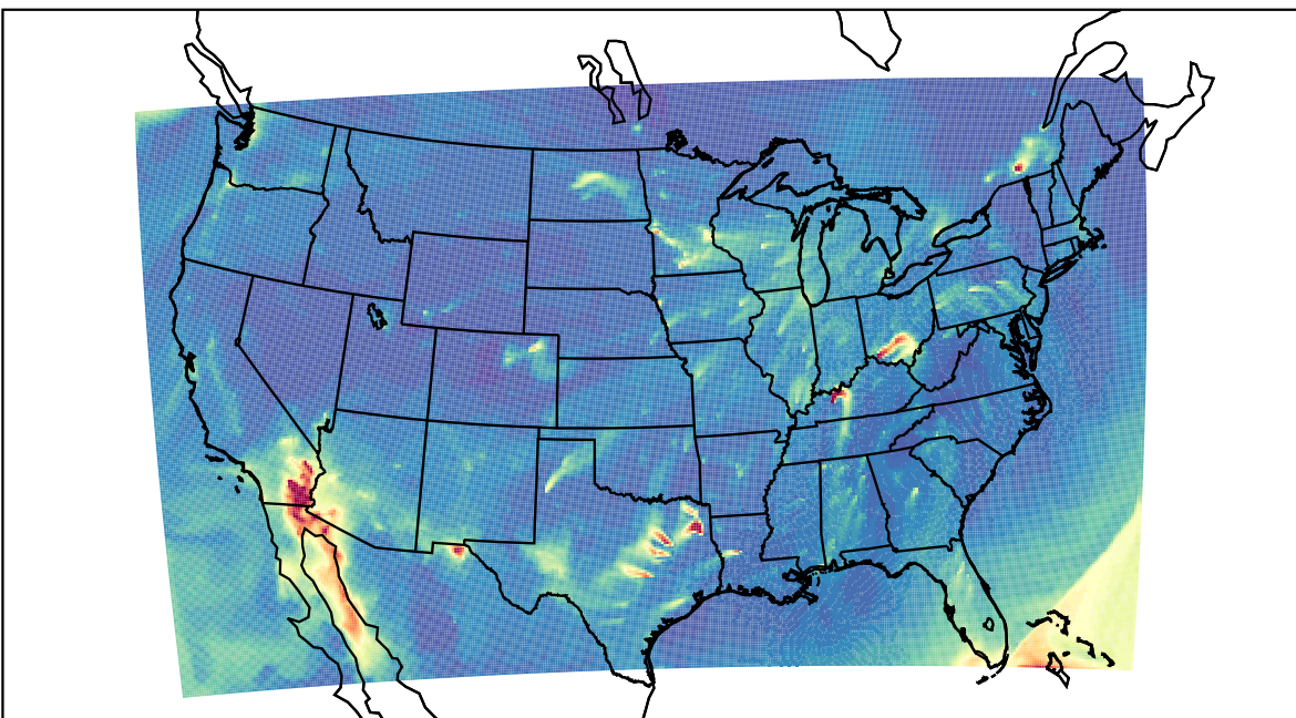
WRF 2023-02-18_14:00:00
