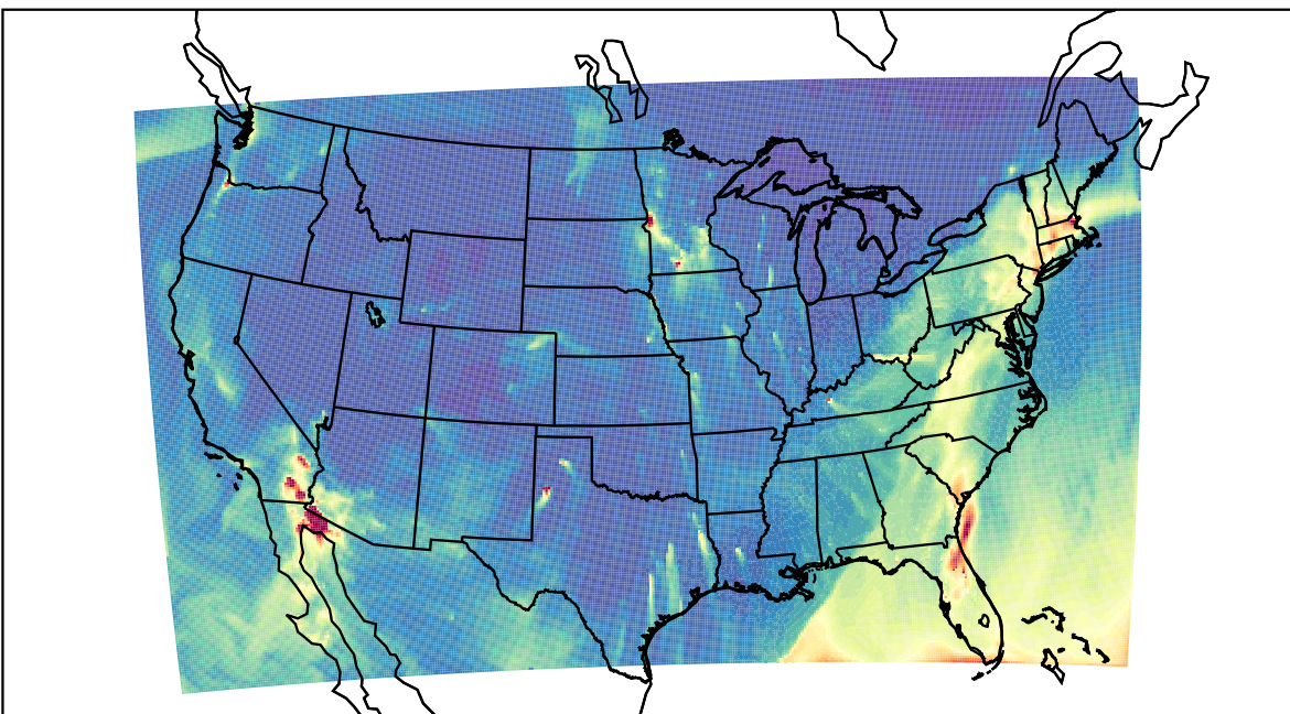
WRF 2023-02-17_10:00:00
