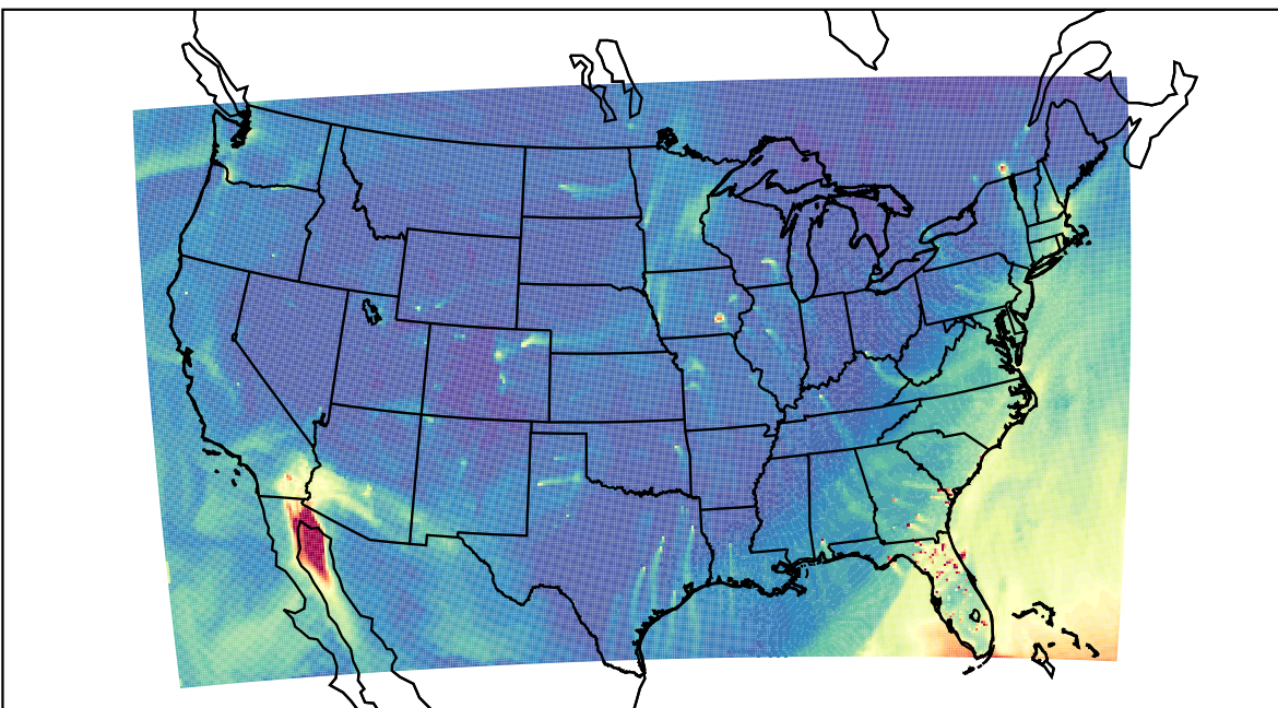
WRF 2023-02-17_20:00:00
