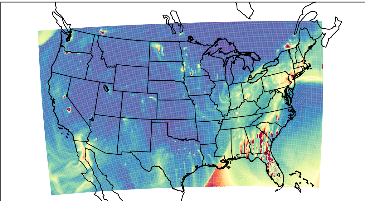
WRF 2023-02-17_00:00:00
