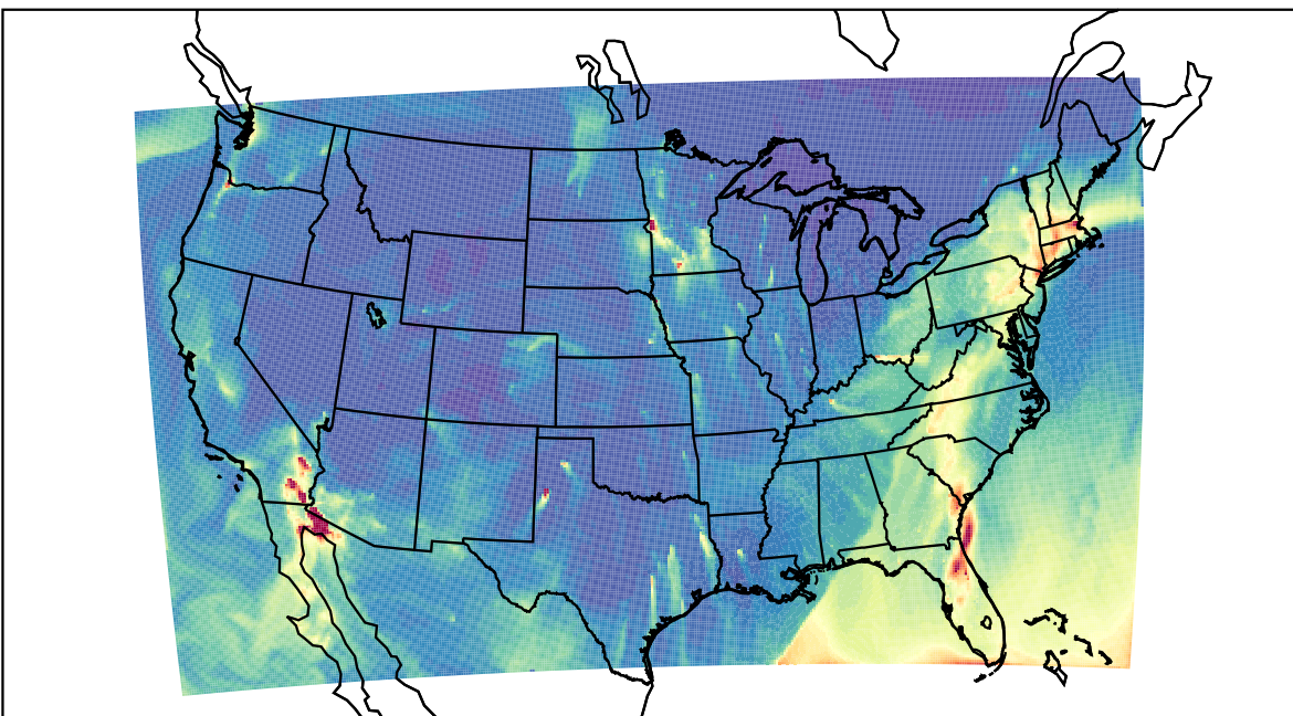
WRF 2023-02-17_09:00:00
