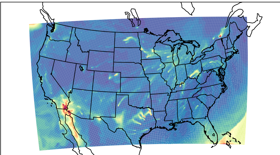
WRF 2023-02-18_16:00:00
