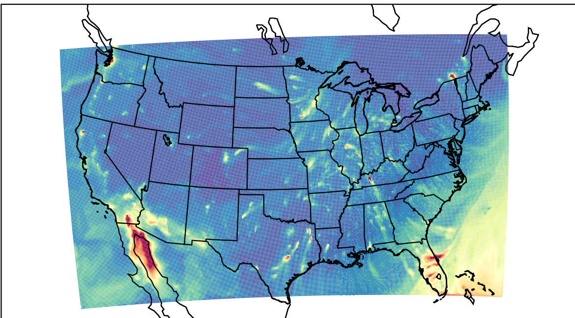
WRF 2023-02-18_03:00:00
