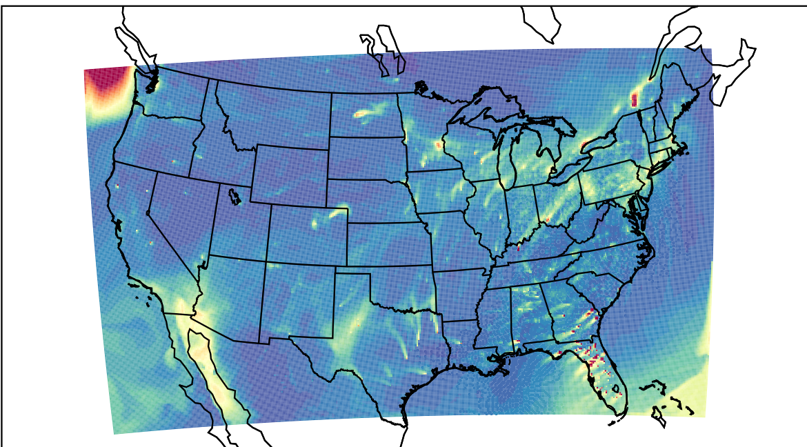
WRF 2023-02-18_23:00:00
