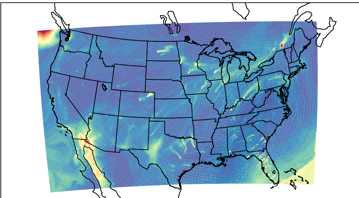
WRF 2023-02-18_20:00:00
