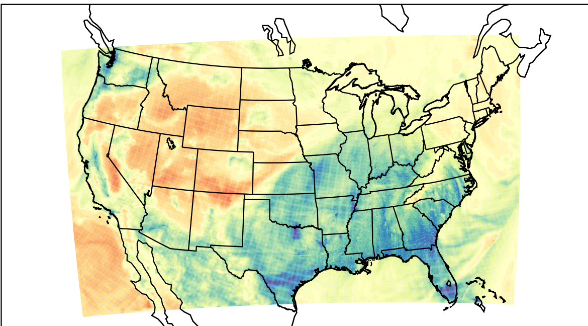
WRF (2023-02-18_10:00:00)
