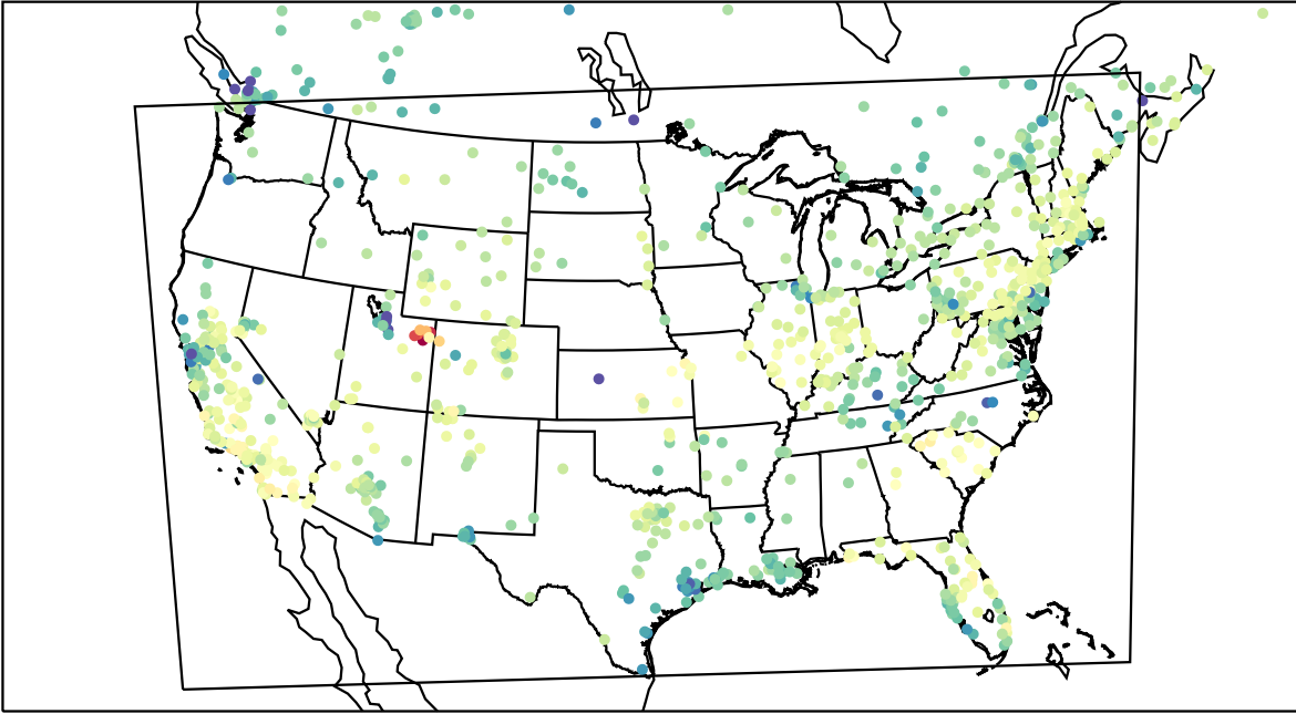
AirNOW (2023-02-20_20:00:00)
