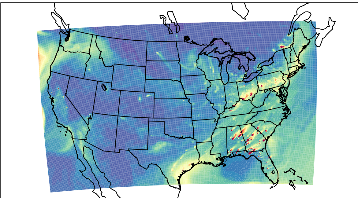
WRF 2023-02-20_23:00:00
