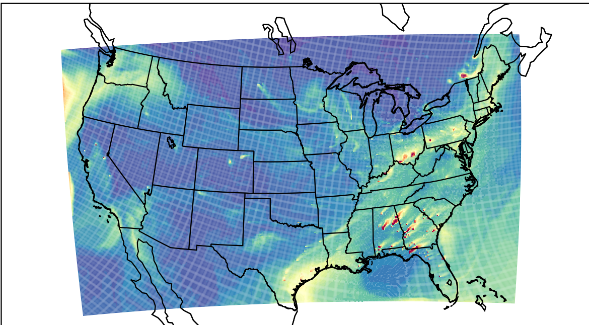
WRF 2023-02-20_22:00:00
