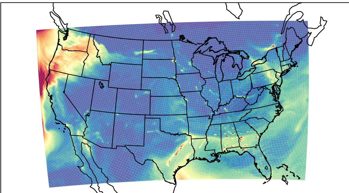
WRF 2023-02-21_18:00:00
