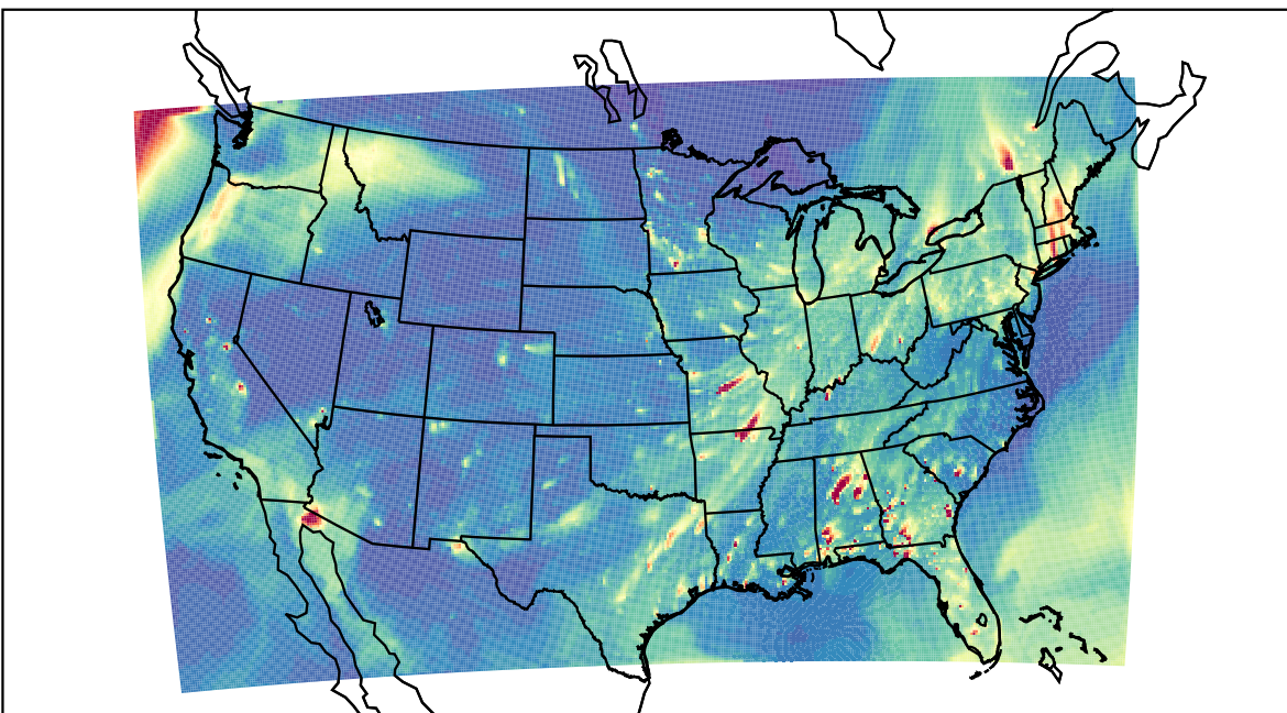
WRF 2023-02-20_01:00:00
