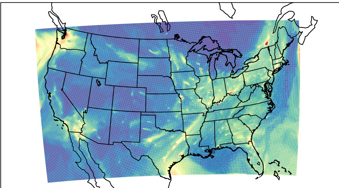
WRF 2023-02-20_14:00:00
