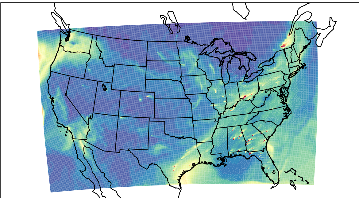
WRF 2023-02-20_19:00:00
