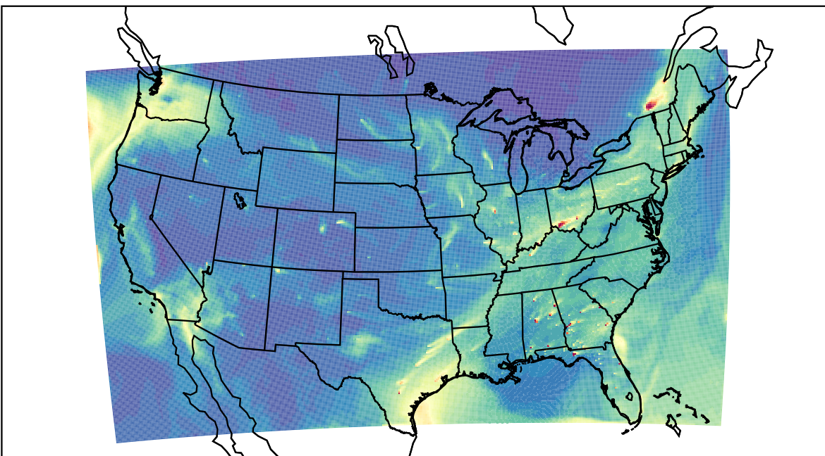
WRF 2023-02-20_18:00:00
