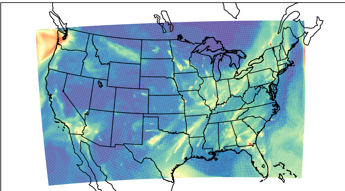
WRF 2023-02-20_10:00:00
