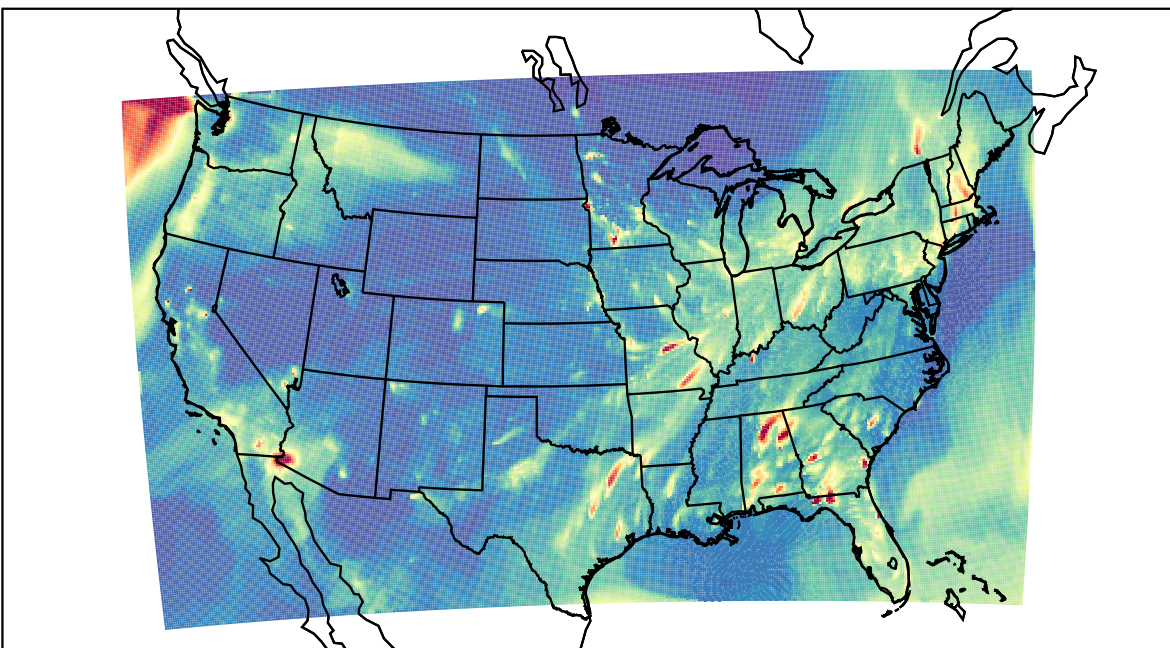
WRF 2023-02-20_04:00:00
