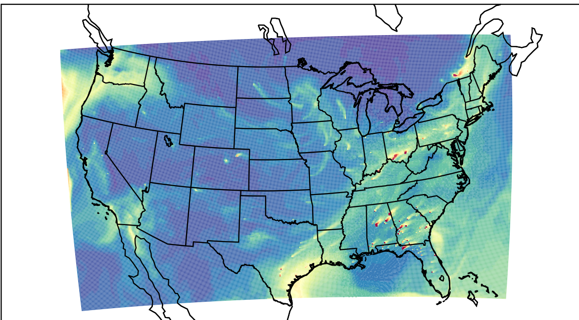
WRF 2023-02-20_20:00:00
