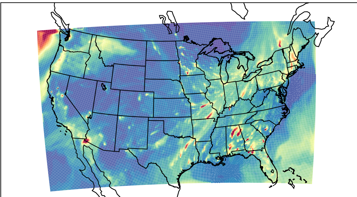
WRF 2023-02-20_03:00:00
