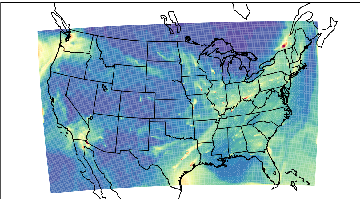
WRF 2023-02-20_16:00:00
