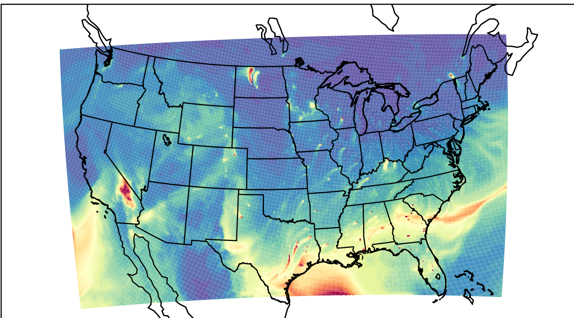
WRF 2023-02-24_18:00:00
