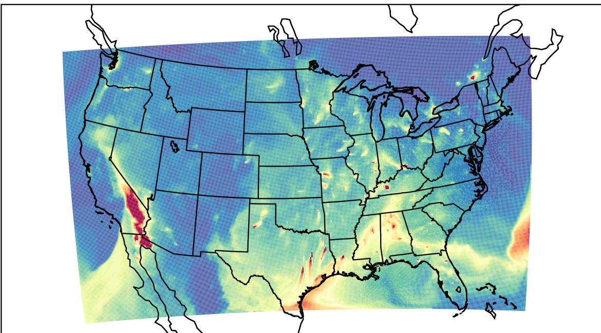
WRF 2023-02-25_13:00:00
