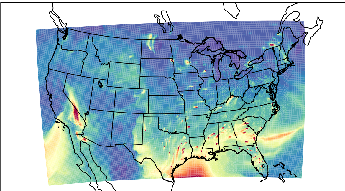
WRF 2023-02-24_23:00:00
