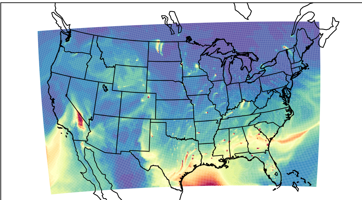
WRF 2023-02-24_20:00:00
