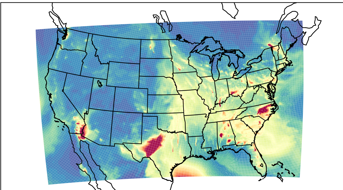
WRF 2023-02-27_04:00:00
