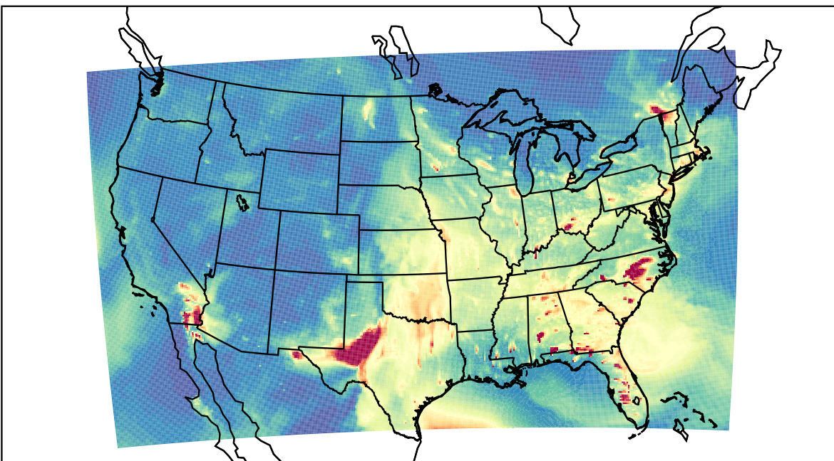
WRF 2023-02-27_01:00:00
