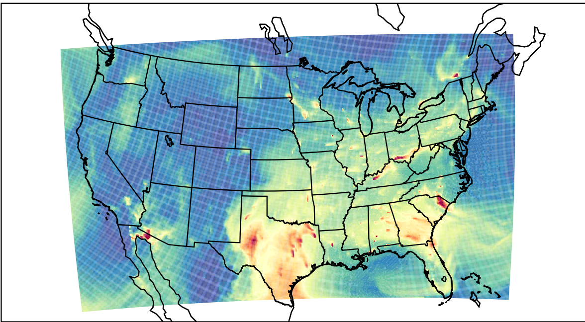
WRF 2023-02-26_14:00:00
