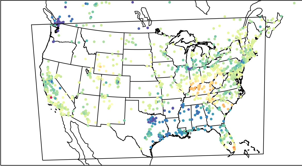
AirNOW (2023-03-01_18:00:00)
