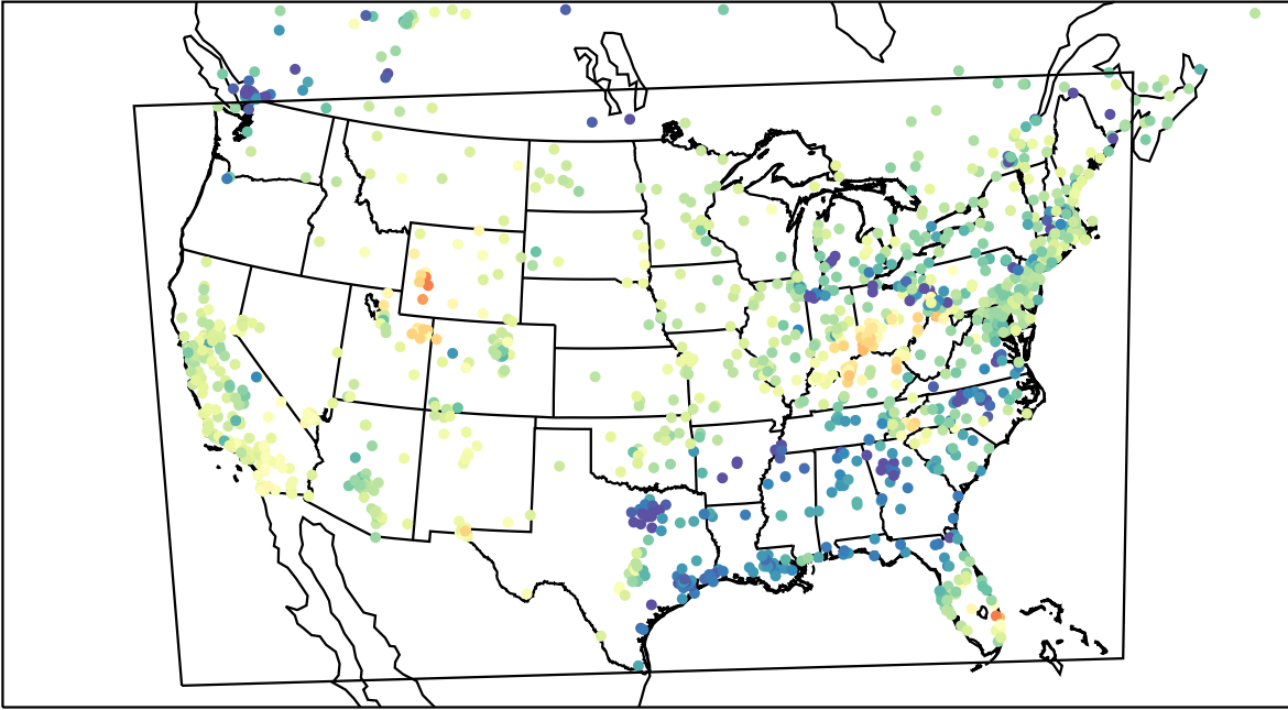
AirNOW (2023-03-01_23:00:00)
