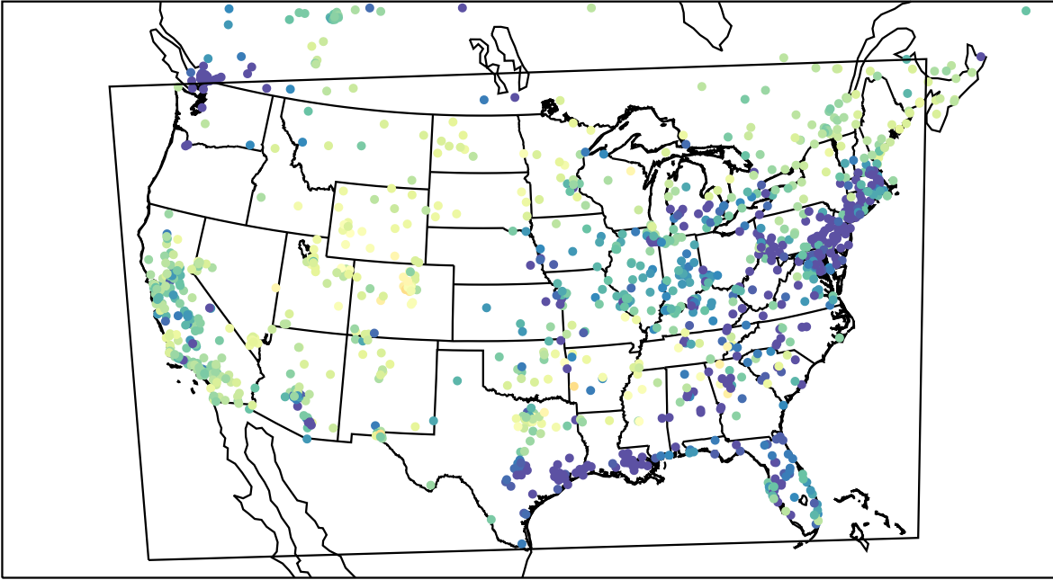
AirNOW (2023-03-01_03:00:00)
