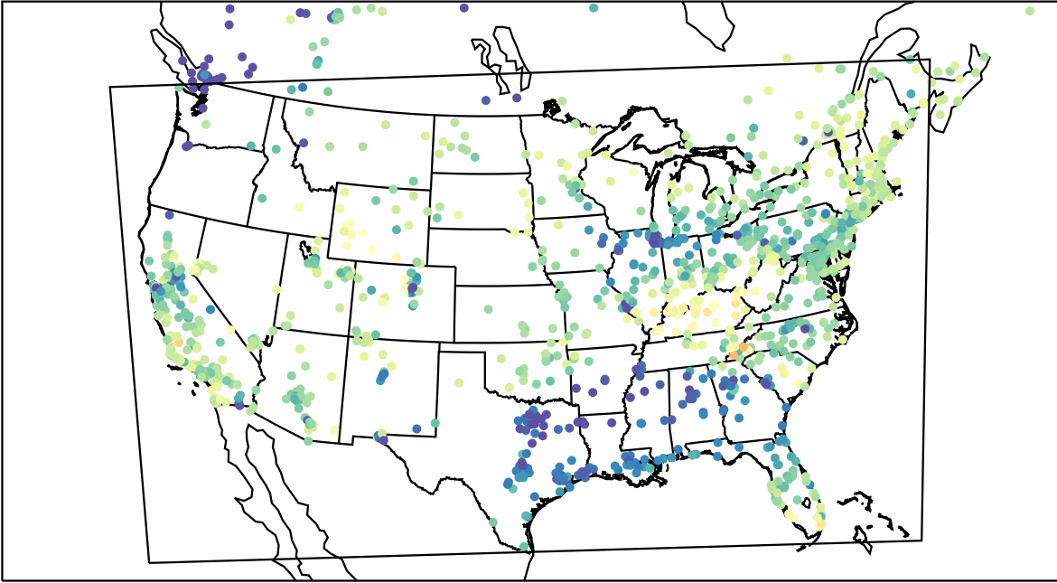
AirNOW (2023-03-01_16:00:00)
