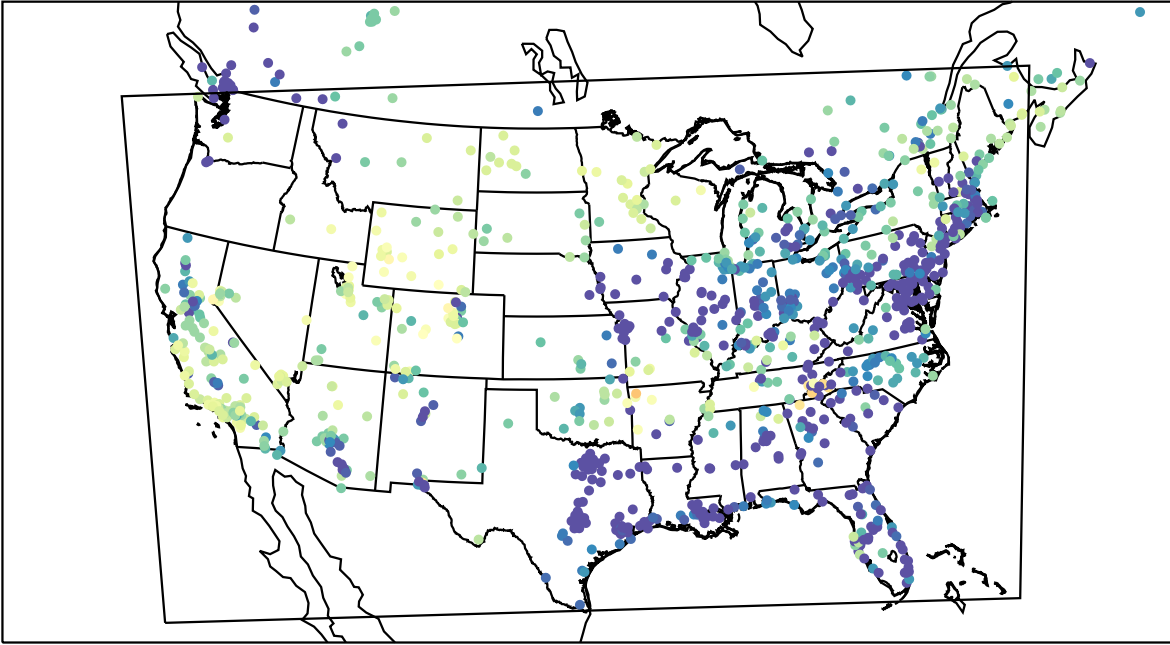
AirNOW (2023-03-01_10:00:00)
