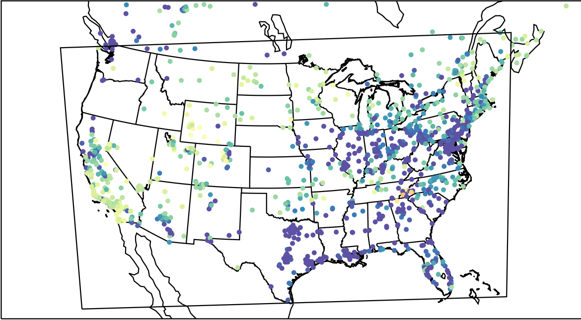
AirNOW (2023-03-01_13:00:00)
