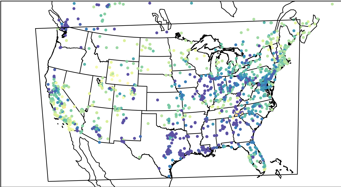
AirNOW (2023-03-01_14:00:00)
