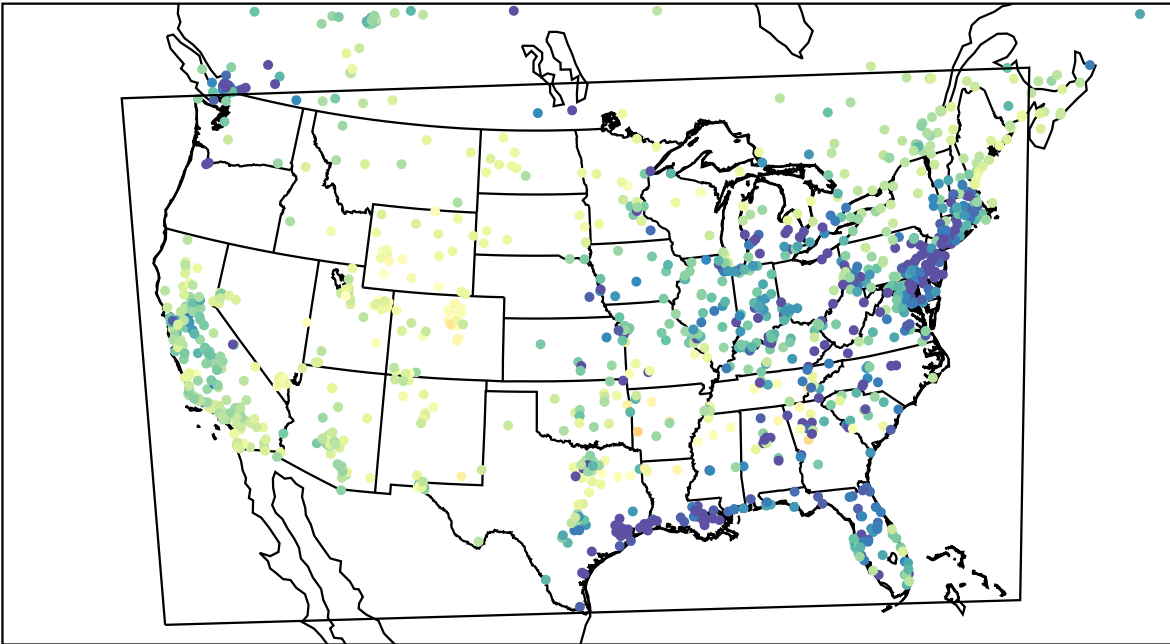
AirNOW (2023-03-01_01:00:00)
