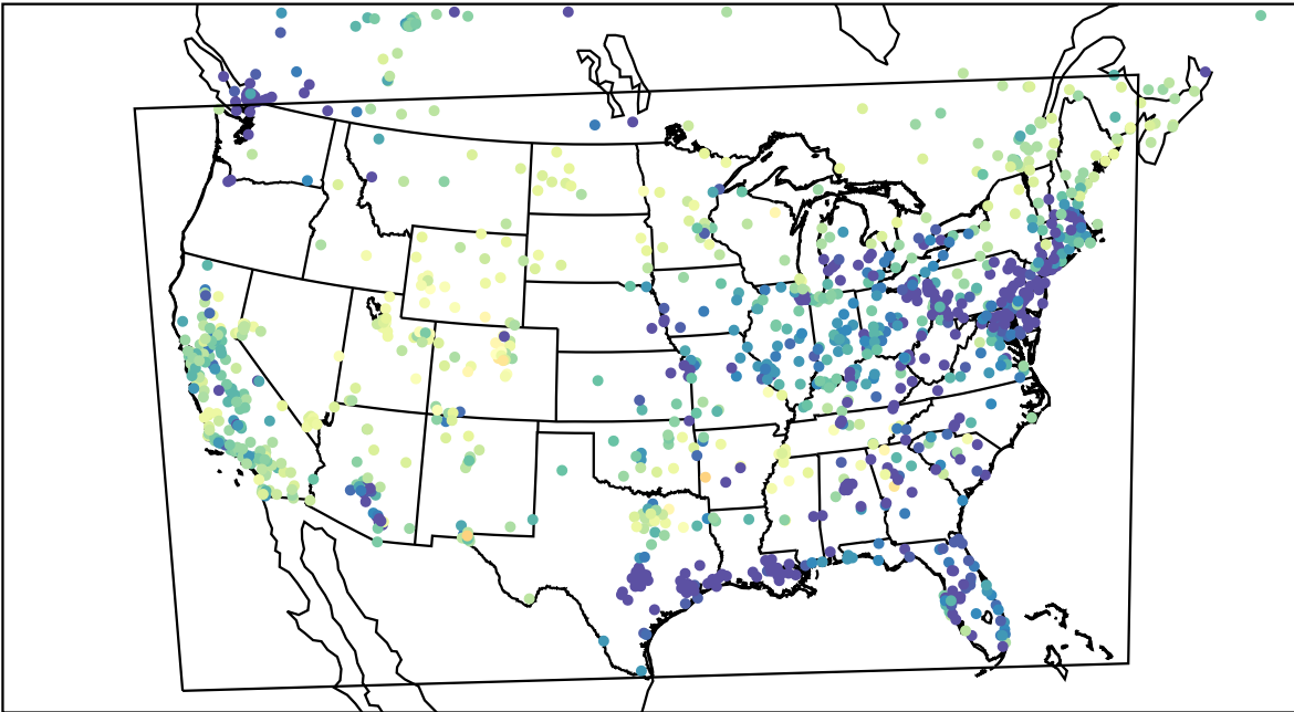
AirNOW (2023-03-01_04:00:00)
