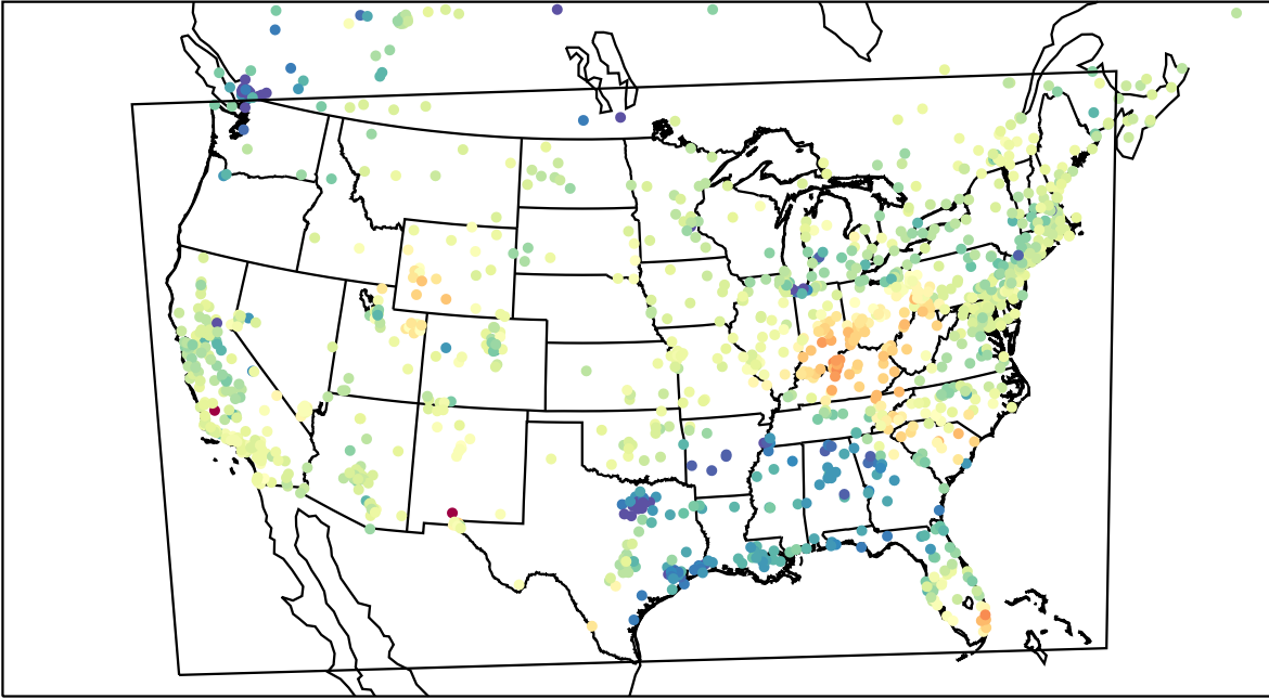
AirNOW (2023-03-01_20:00:00)
