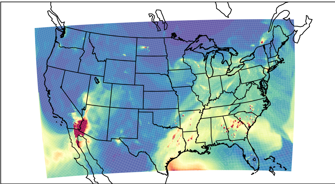
WRF 2023-03-01_20:00:00
