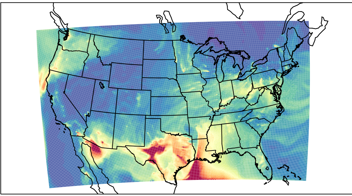
WRF 2023-03-03_06:00:00
