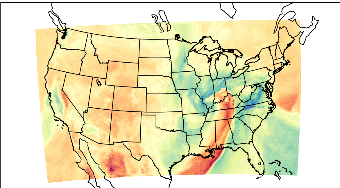
WRF (2023-03-03_19:00:00)
