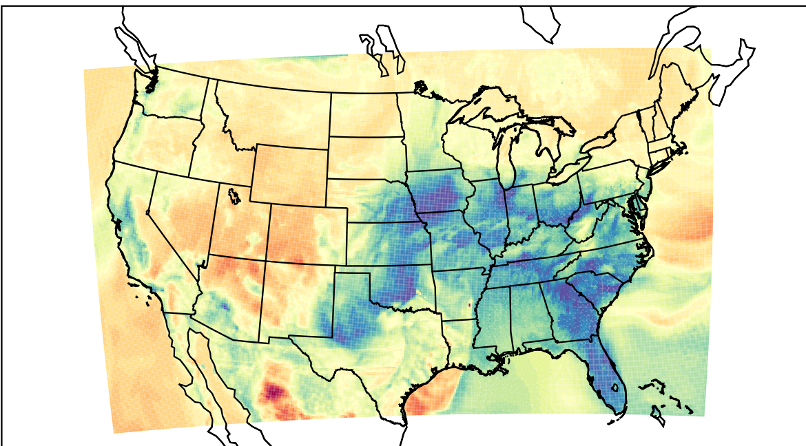
WRF (2023-03-03_08:00:00)
