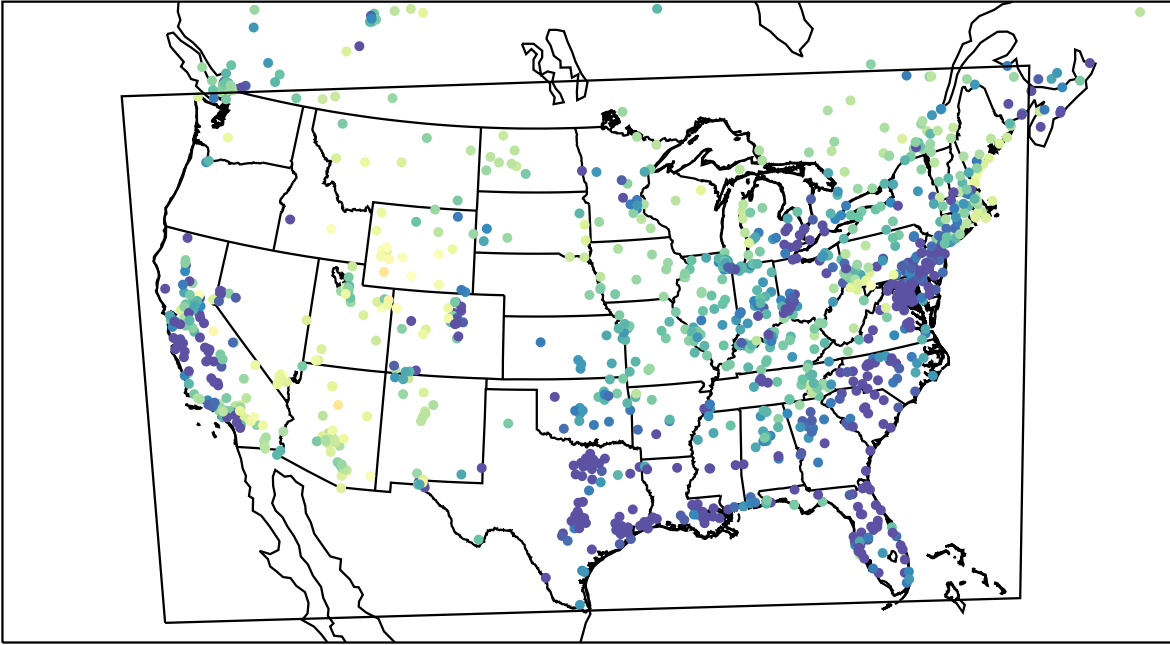
AirNOW (2023-03-02_10:00:00)
