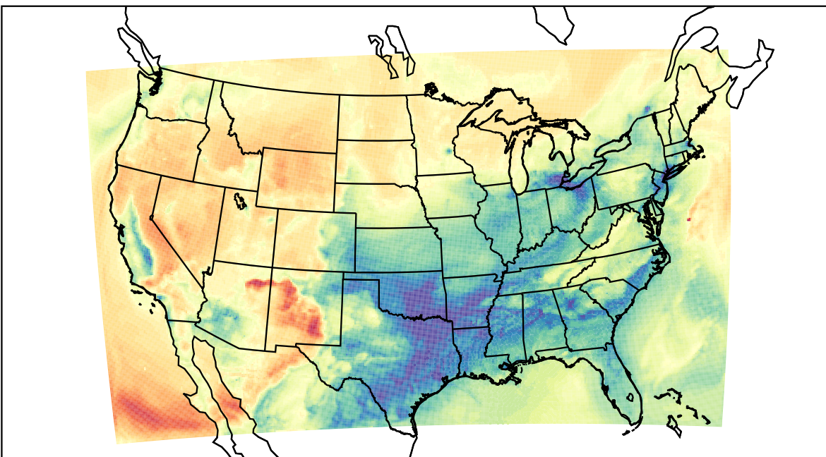
WRF (2023-03-02_15:00:00)
