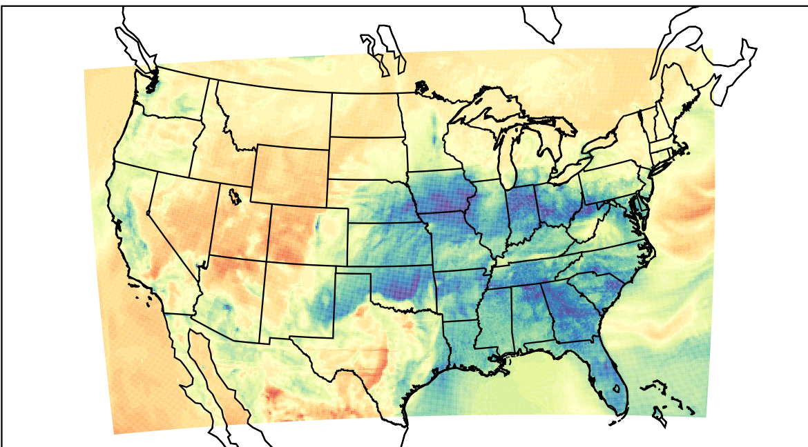
WRF (2023-03-03_04:00:00)
