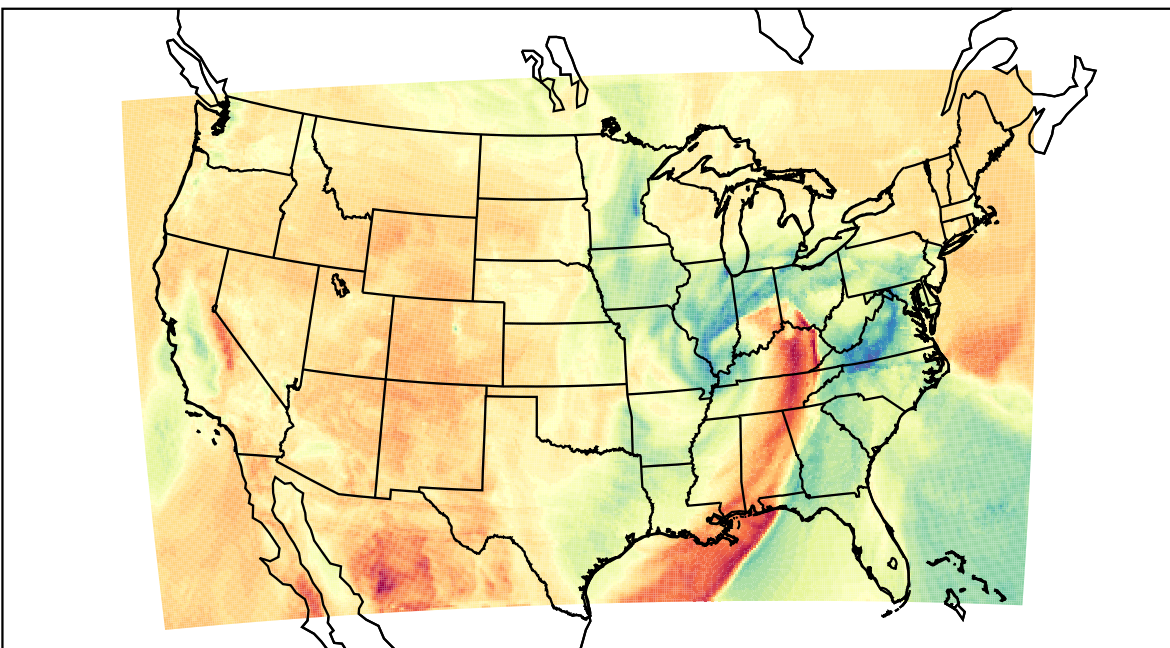
WRF (2023-03-03_20:00:00)
