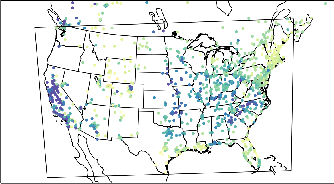
AirNOW (2023-03-03_16:00:00)
