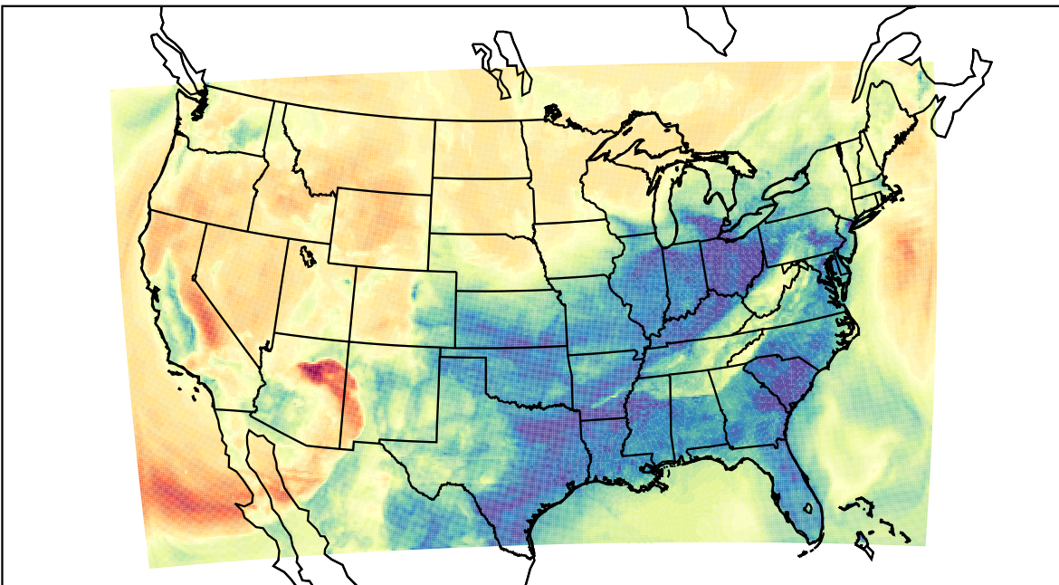
WRF (2023-03-02_10:00:00)
