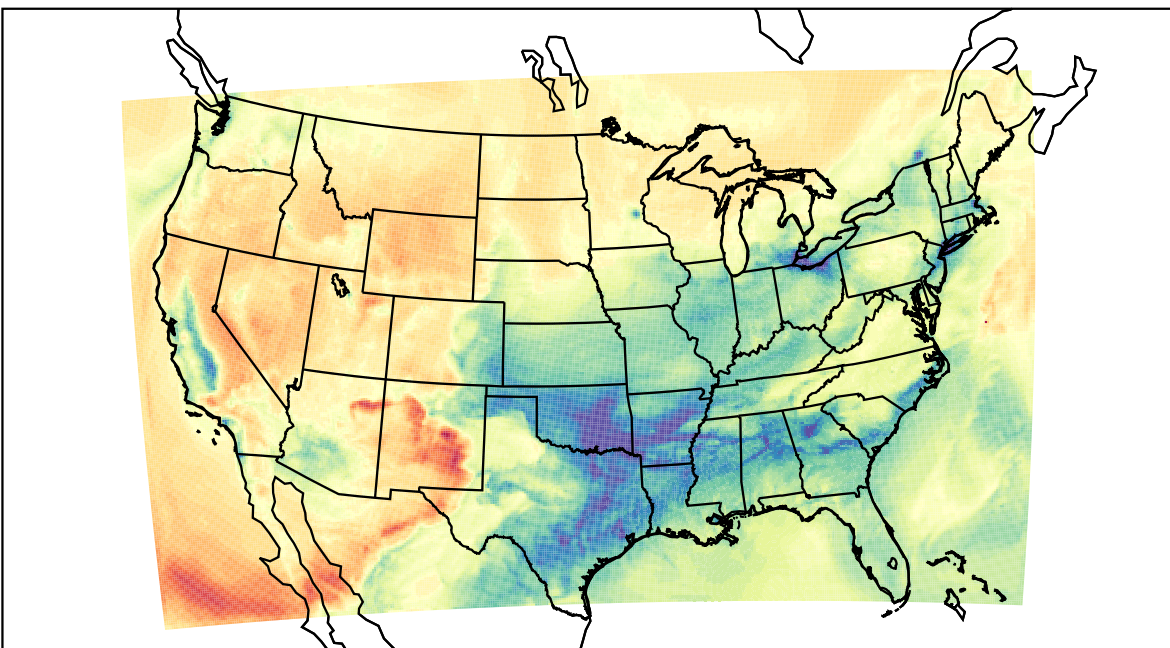
WRF (2023-03-02_16:00:00)
