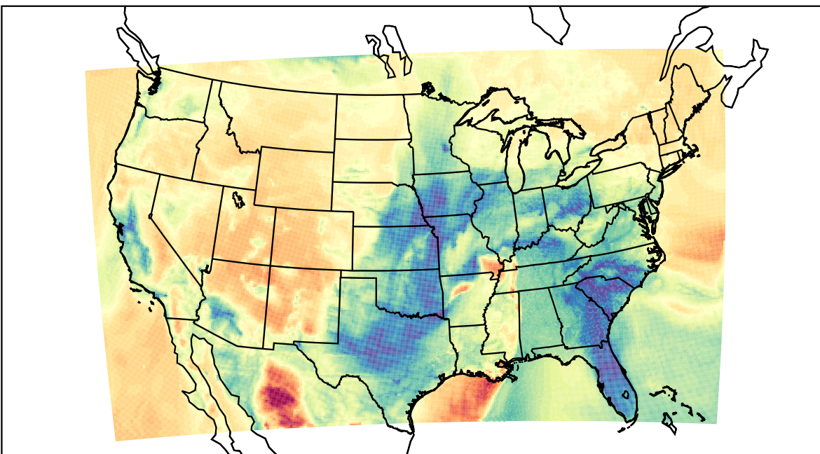
WRF (2023-03-03_13:00:00)
