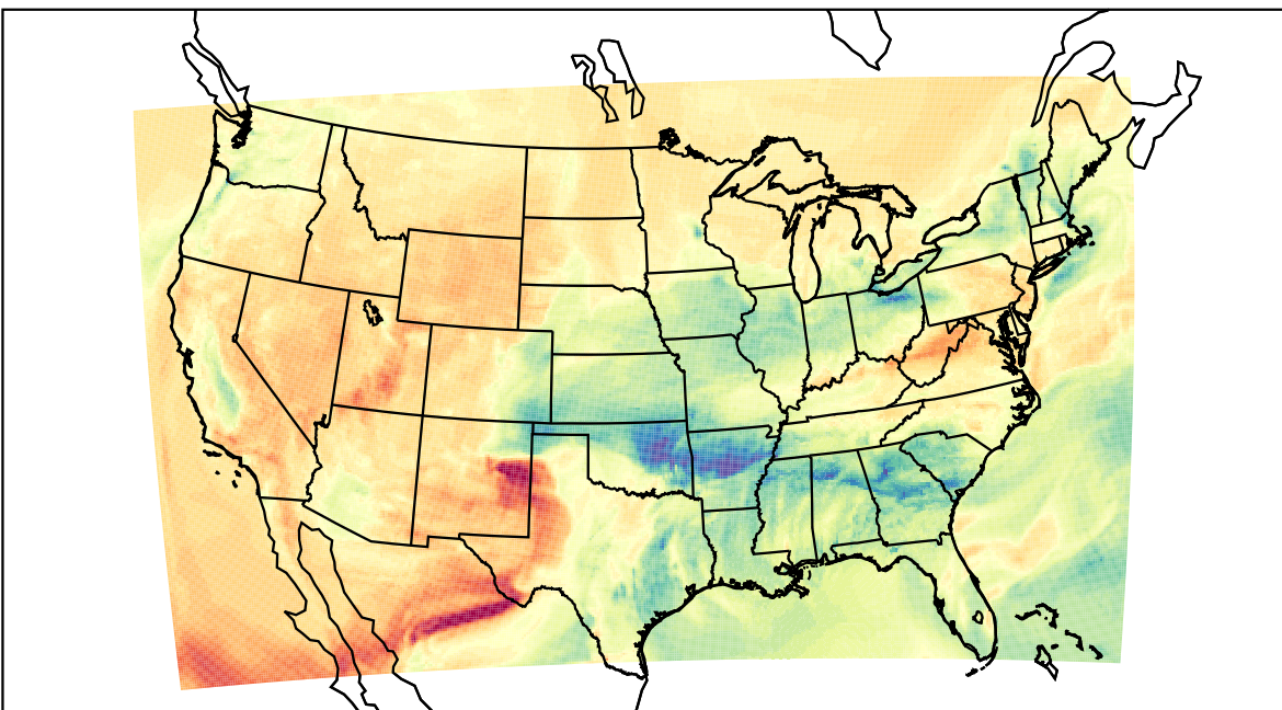
WRF (2023-03-02_20:00:00)
