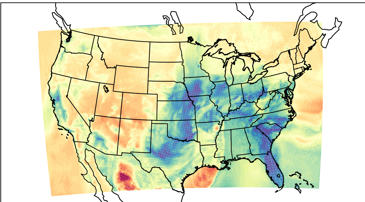
WRF (2023-03-03_11:00:00)
