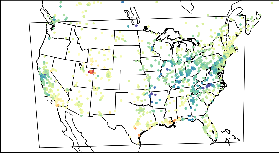
AirNOW (2023-03-03_20:00:00)
