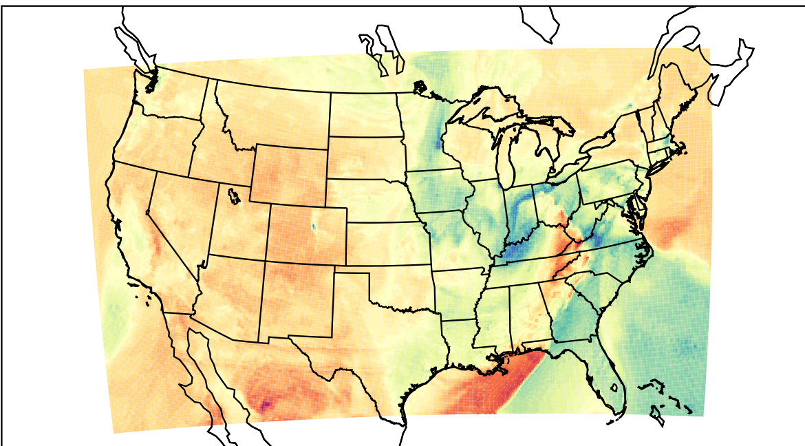
WRF (2023-03-03_23:00:00)
