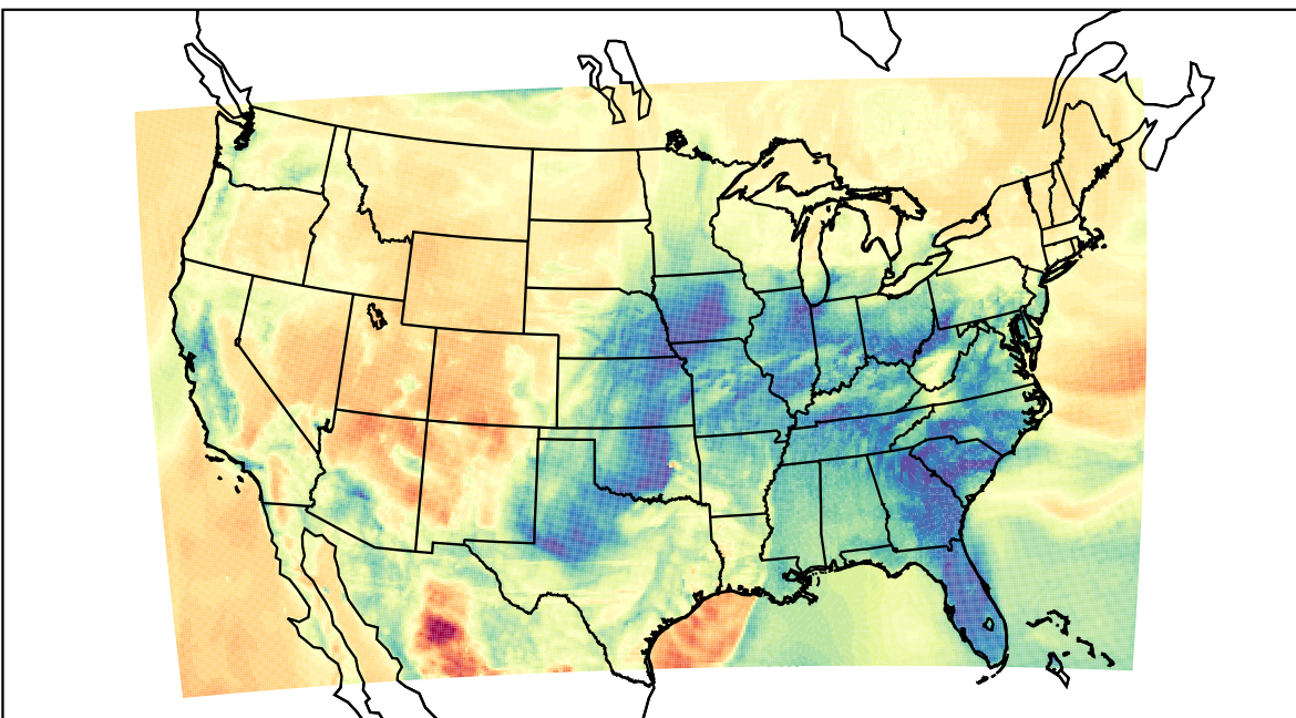
WRF (2023-03-03_09:00:00)
