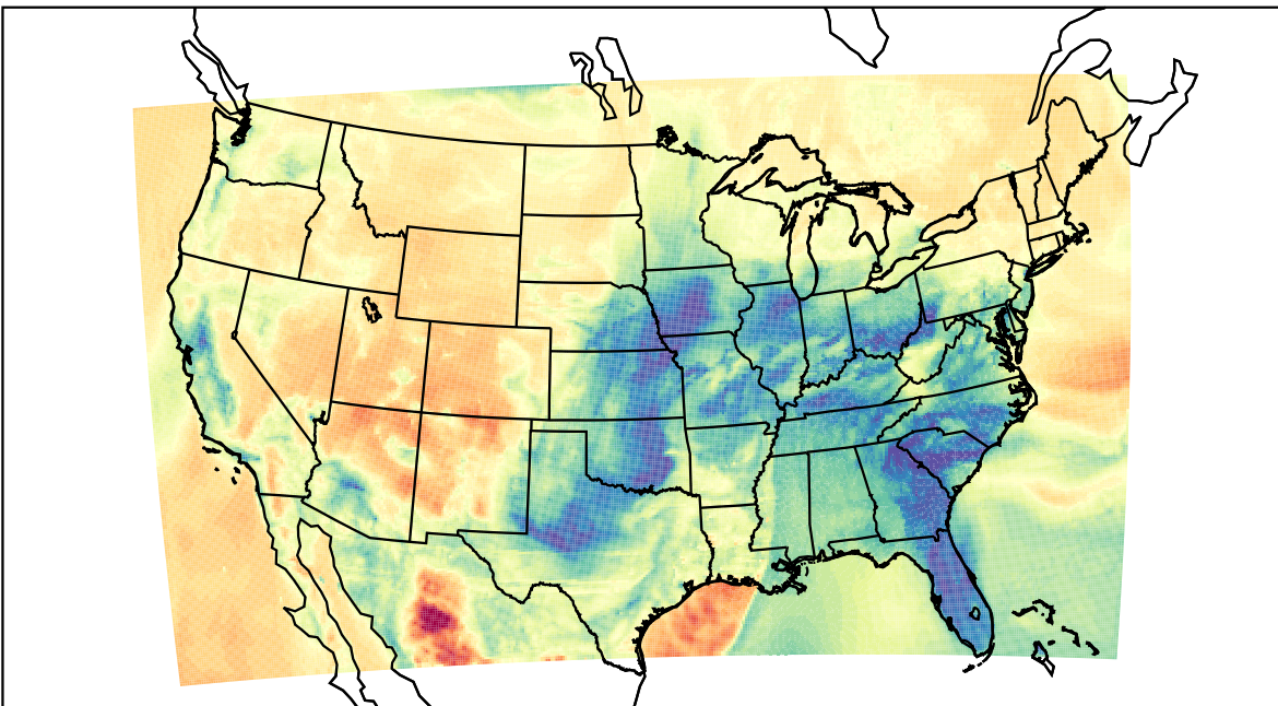
WRF (2023-03-03_10:00:00)
