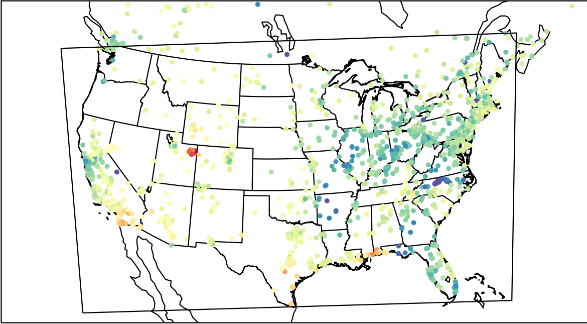
AirNOW (2023-03-03_23:00:00)
