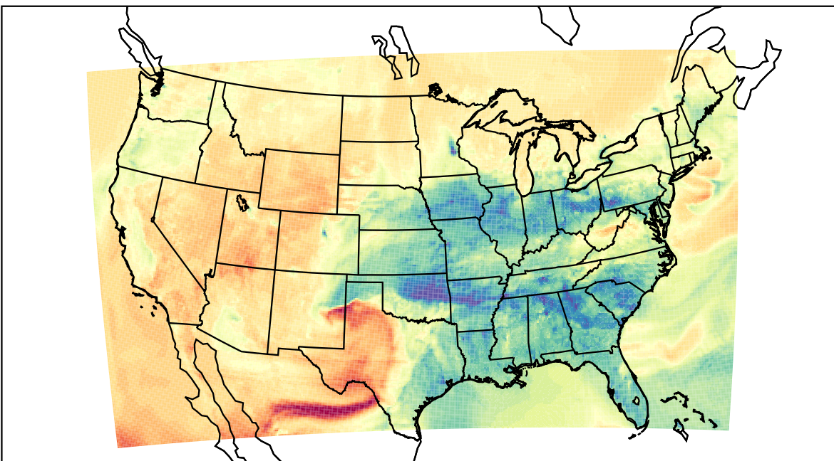
WRF (2023-03-03_00:00:00)
