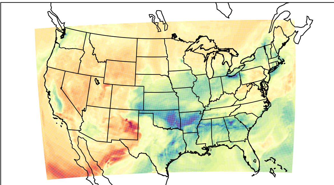
WRF (2023-03-02_18:00:00)
