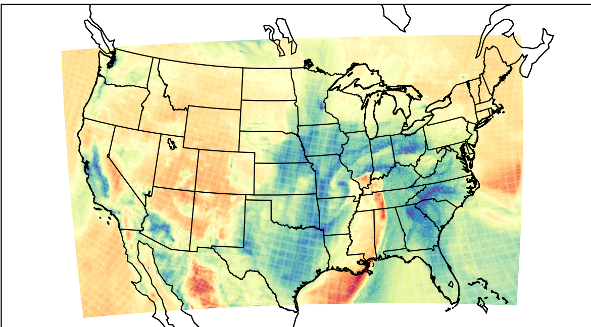
WRF (2023-03-03_15:00:00)
