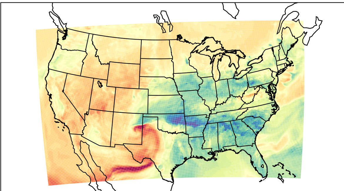
WRF (2023-03-02_23:00:00)
