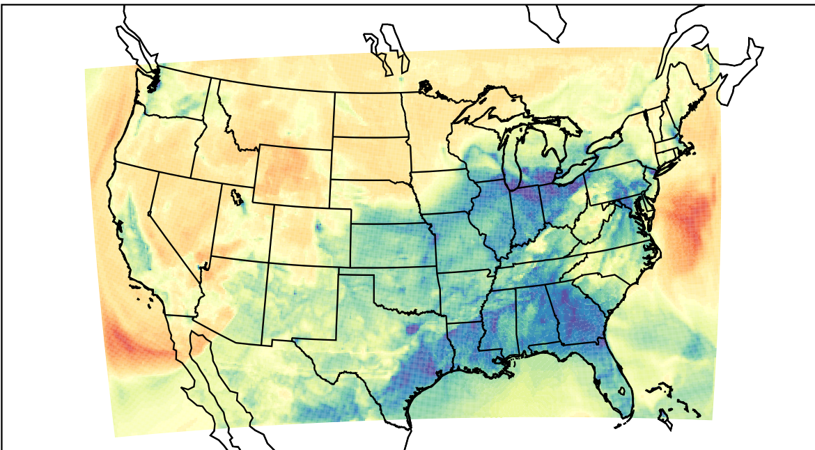
WRF (2023-03-02_03:00:00)
