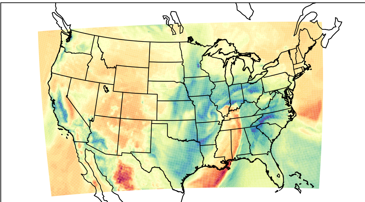
WRF (2023-03-03_16:00:00)
