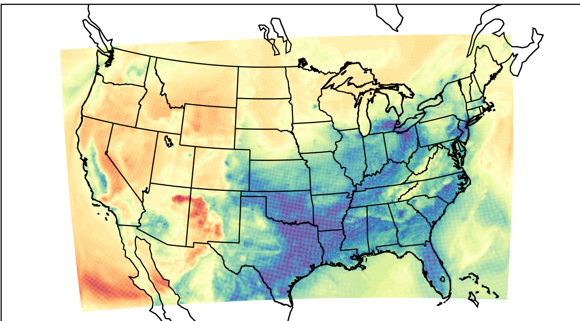
WRF (2023-03-02_14:00:00)
