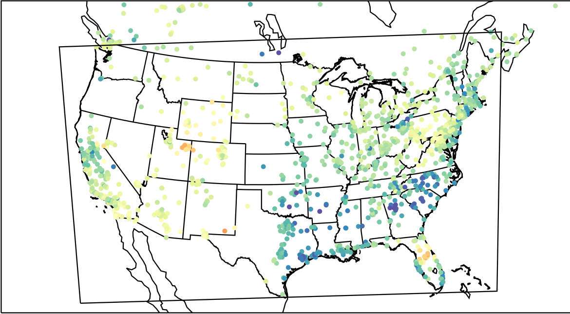
AirNOW (2023-03-02_20:00:00)
