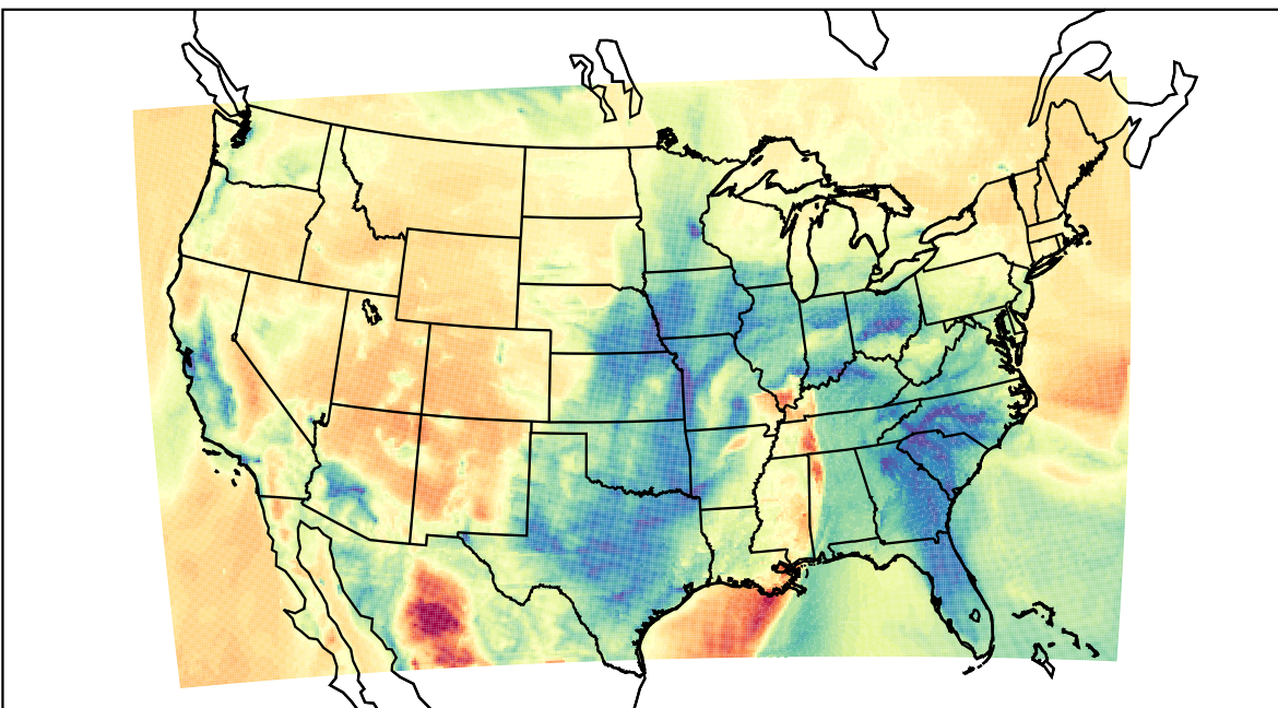
WRF (2023-03-03_14:00:00)
