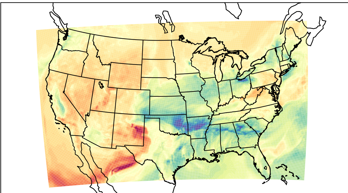
WRF (2023-03-02_19:00:00)
