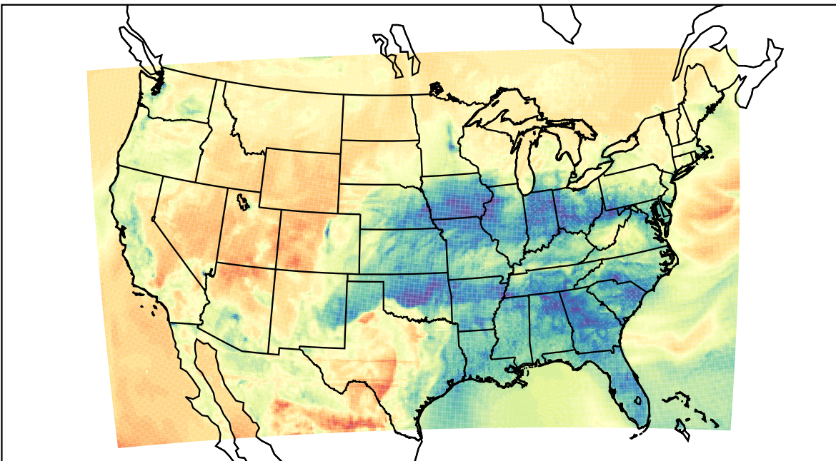
WRF (2023-03-03_03:00:00)
