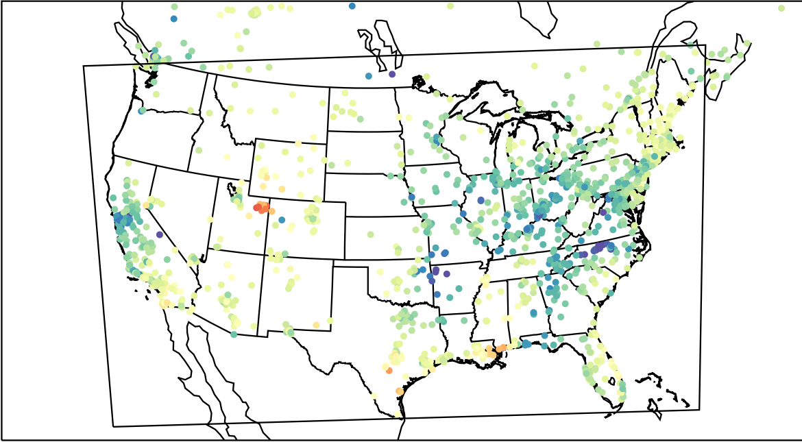
AirNOW (2023-03-03_19:00:00)
