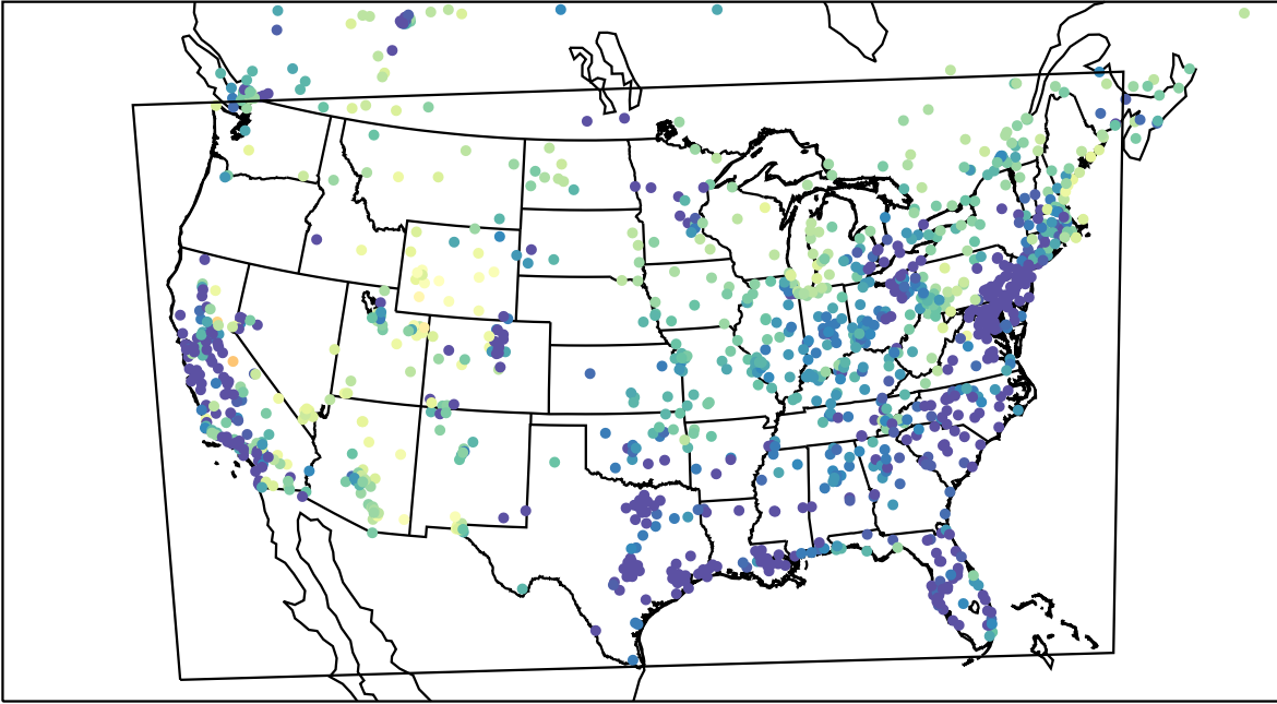
AirNOW (2023-03-02_13:00:00)
