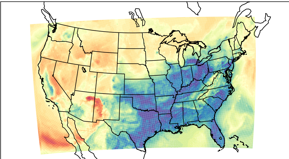
WRF (2023-03-02_13:00:00)
