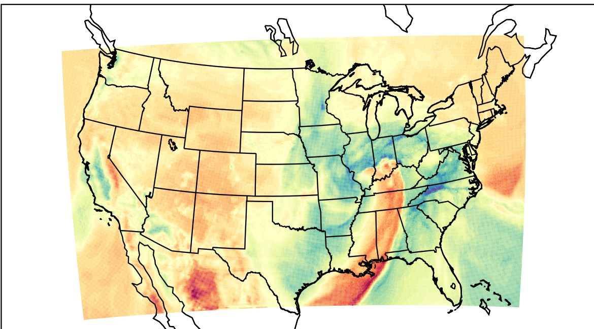
WRF (2023-03-03_18:00:00)
