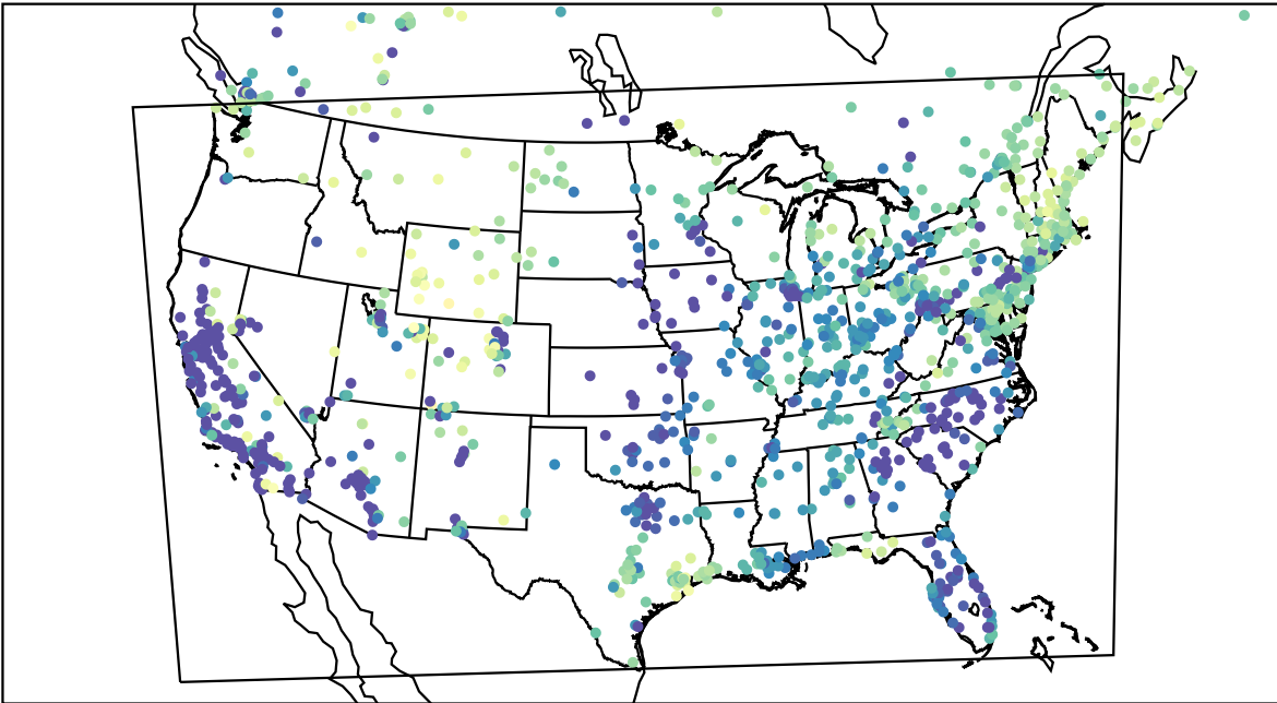
AirNOW (2023-03-03_13:00:00)
