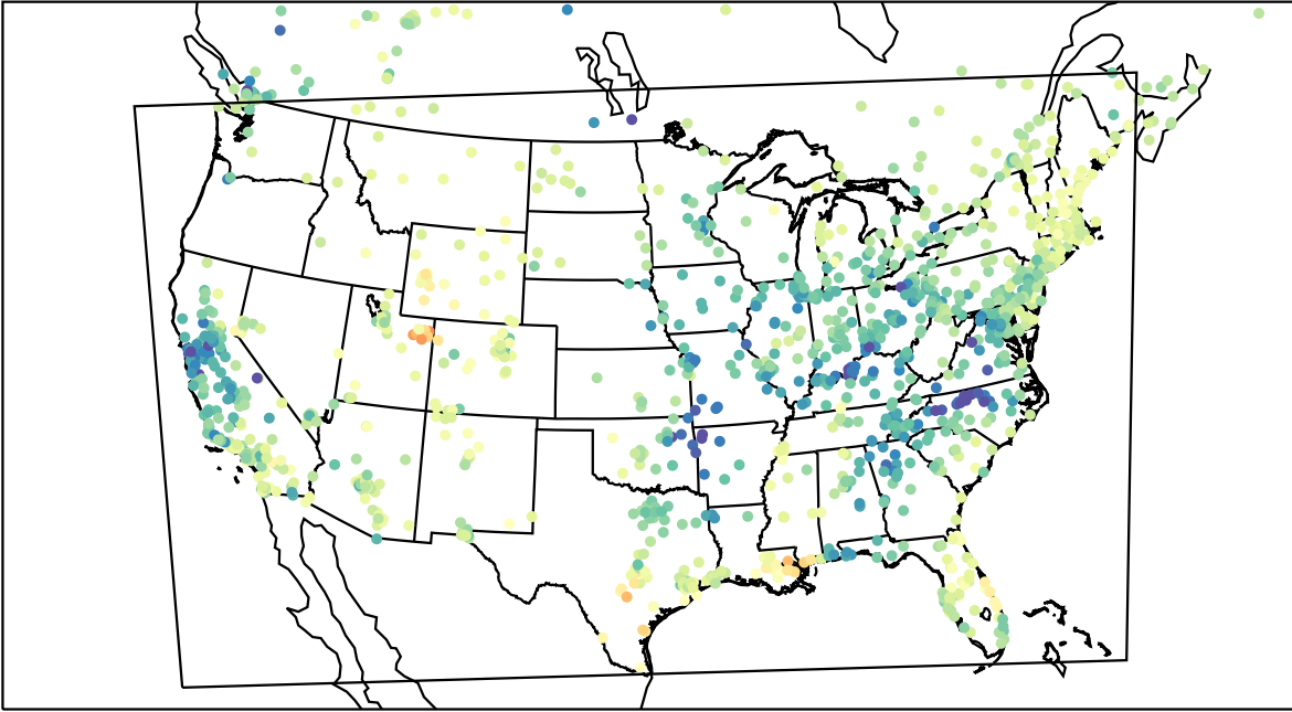
AirNOW (2023-03-03_18:00:00)
