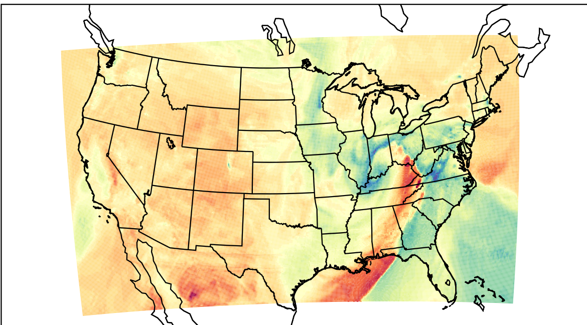
WRF (2023-03-03_22:00:00)
