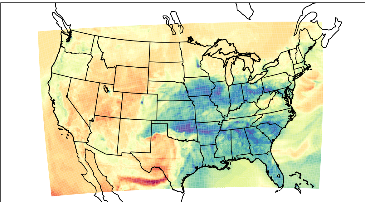
WRF (2023-03-03_01:00:00)
