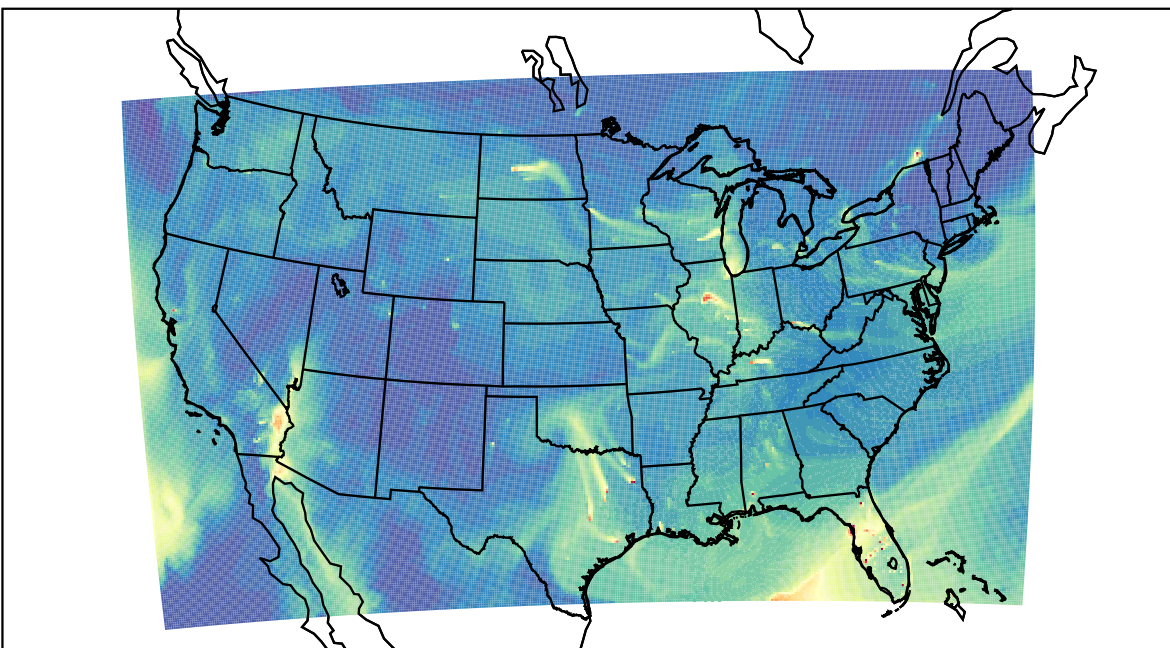
WRF 2023-03-04_20:00:00
