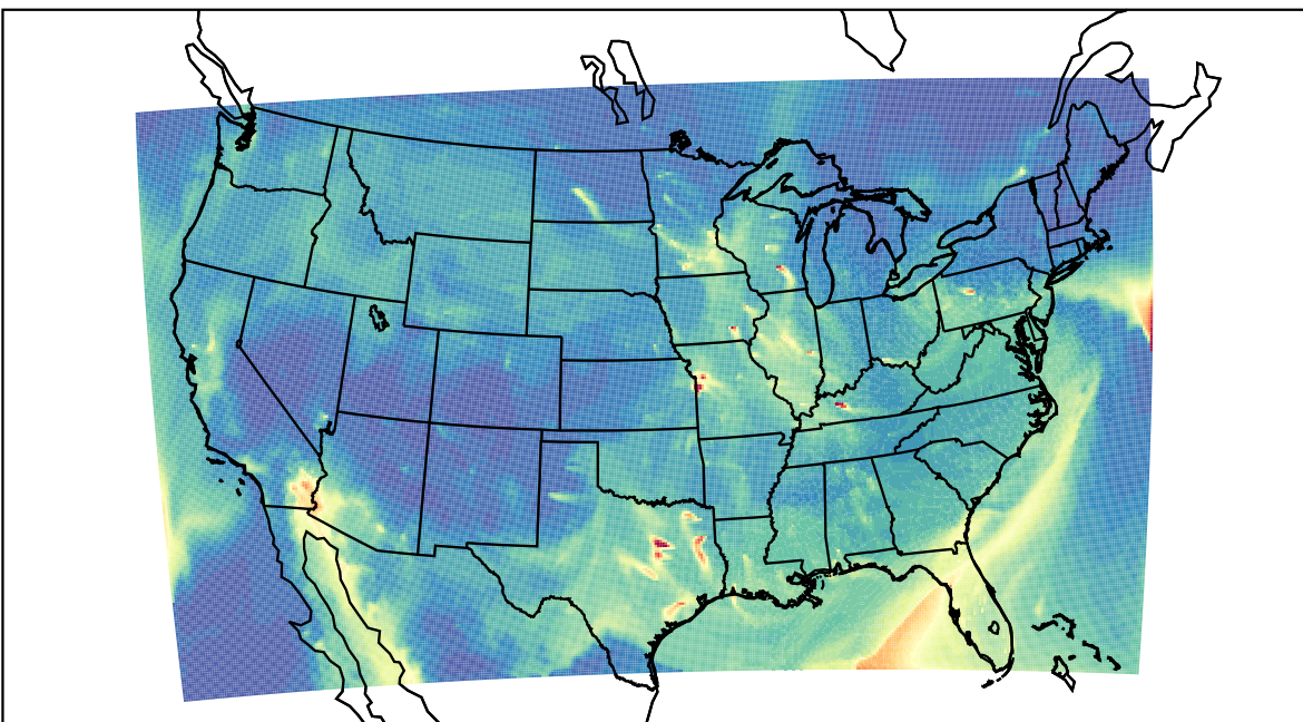
WRF 2023-03-04_10:00:00
