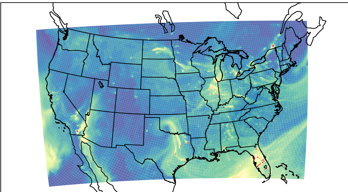
WRF 2023-03-04_23:00:00
