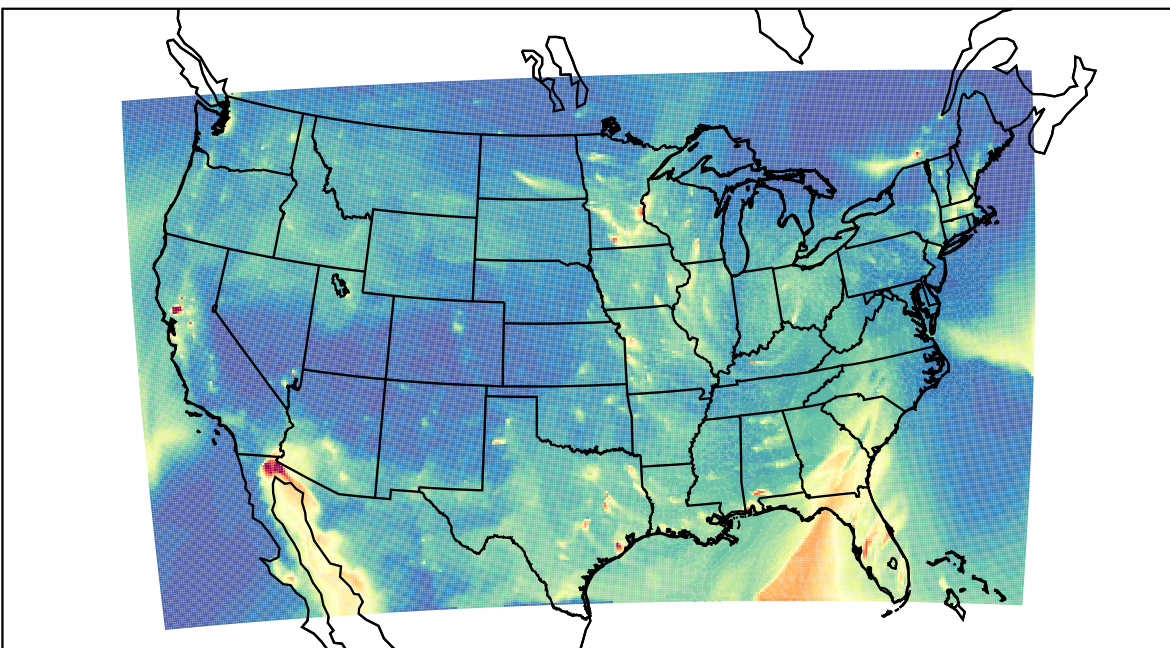
WRF 2023-03-04_03:00:00
