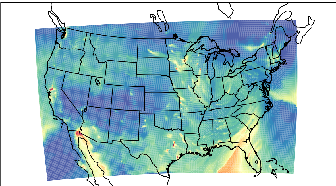
WRF 2023-03-04_04:00:00
