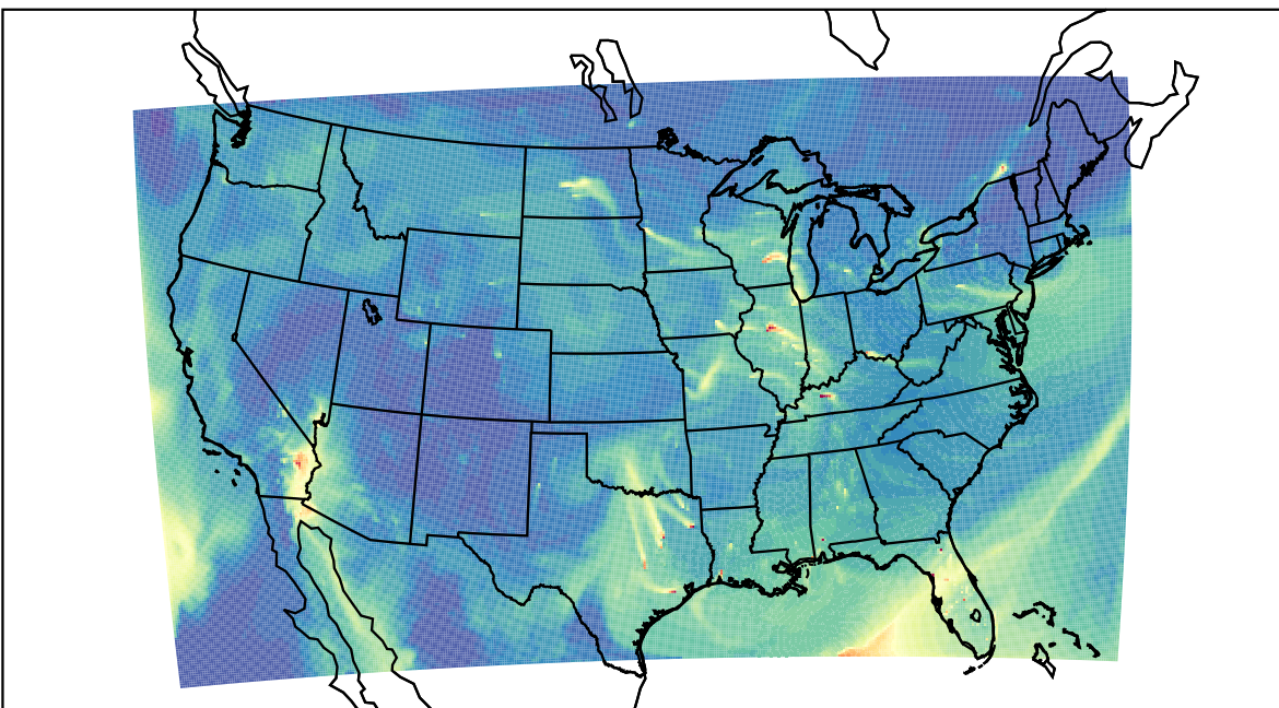
WRF 2023-03-04_18:00:00
